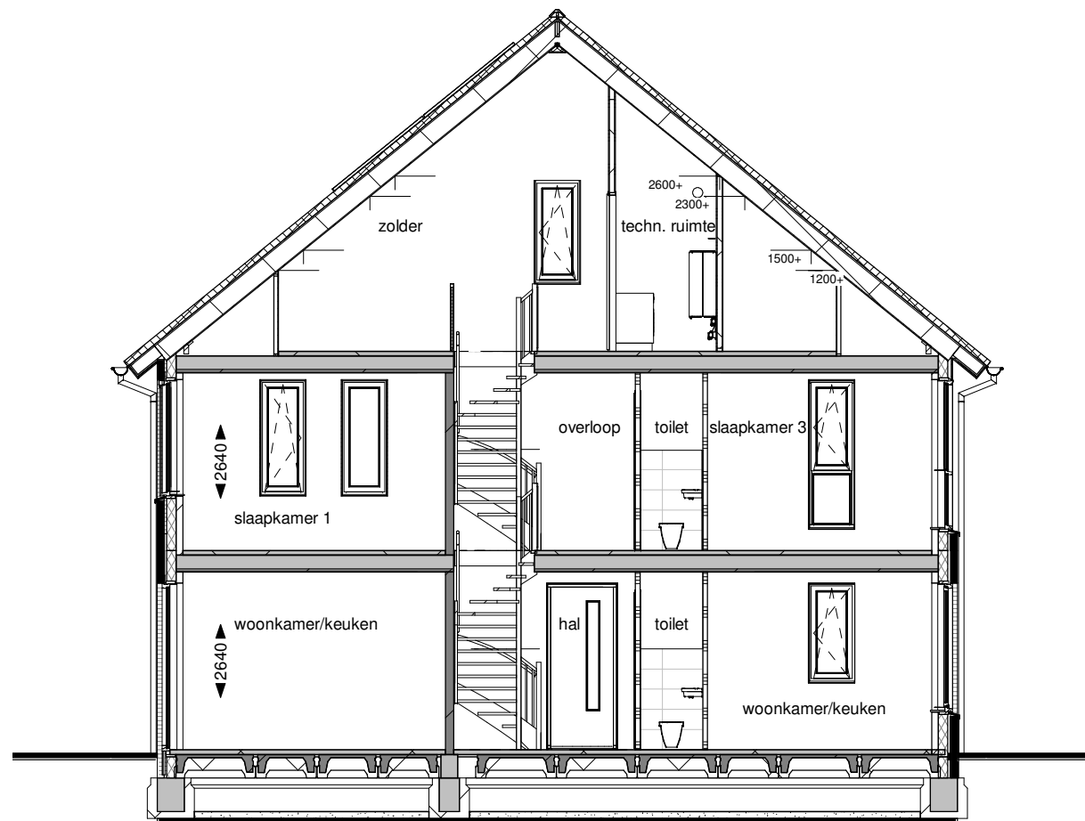
Doorsnede A
