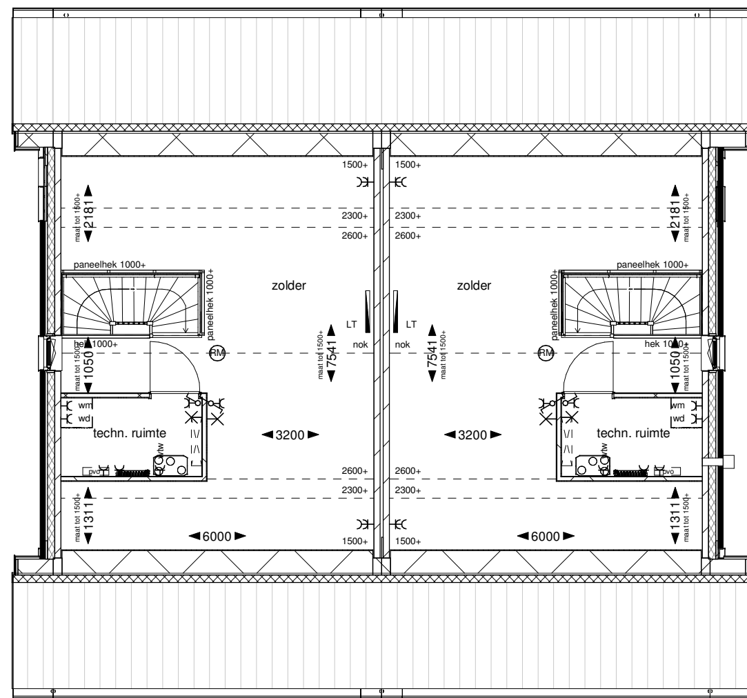
Tweede verdieping
