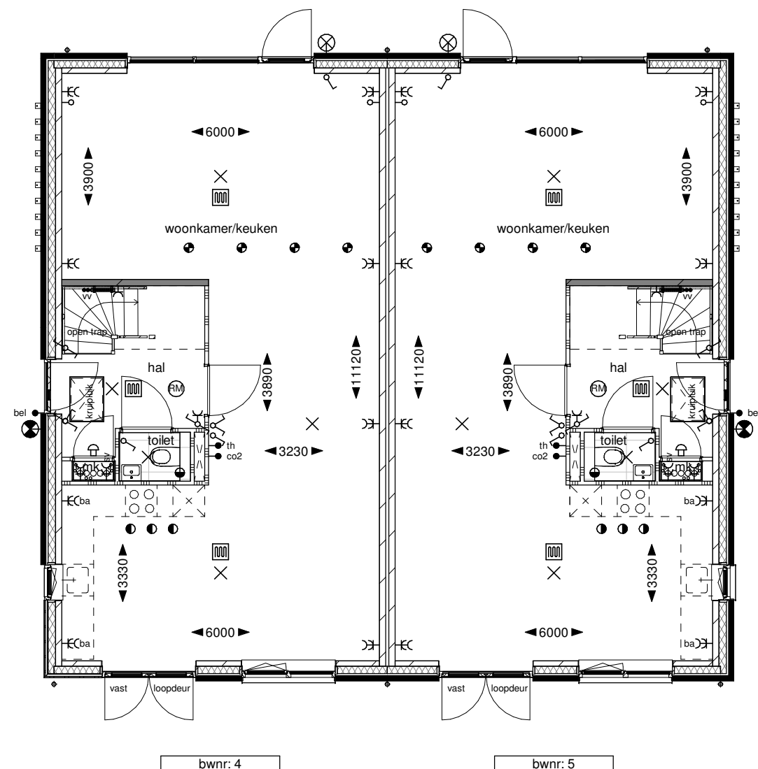
Begane grond
