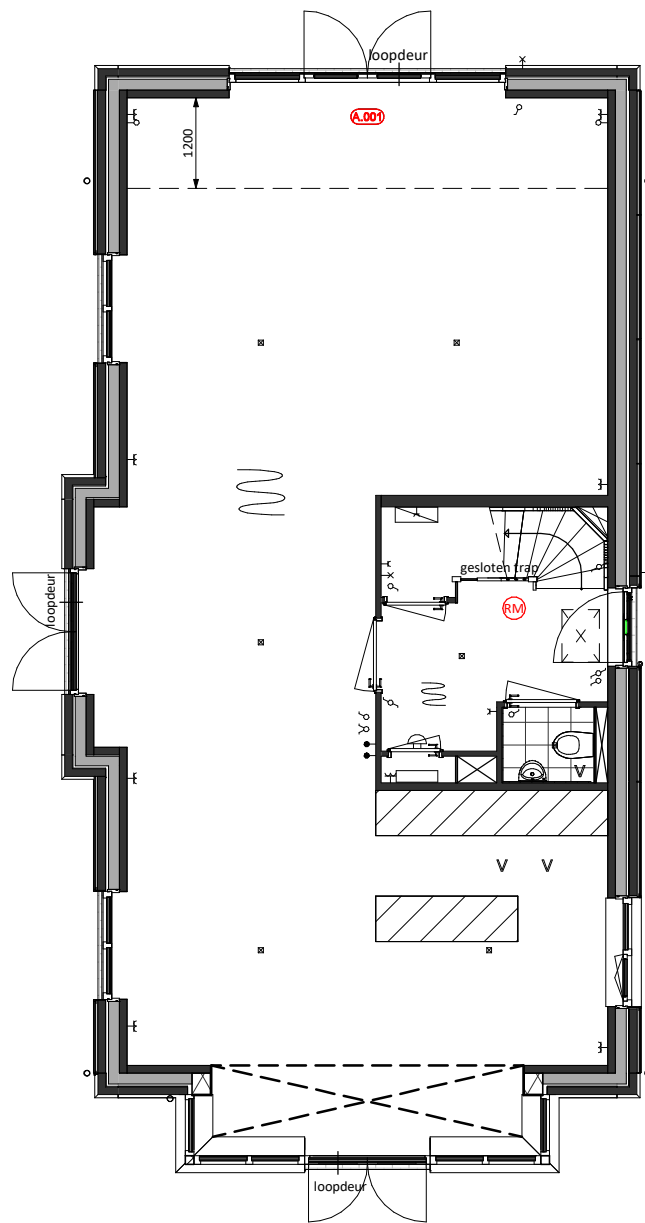
Begane grond A.001 = Uitbouw achtergevel 1.2m
