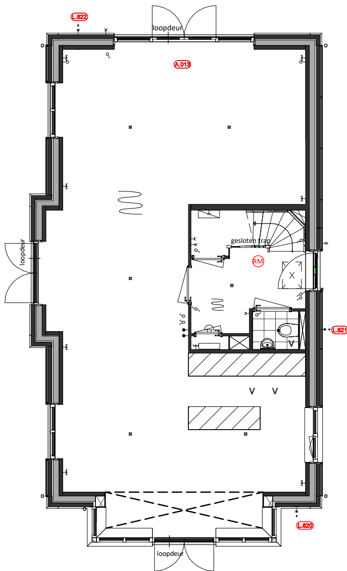
Begane grond A.013 = Wijzigen loopdeur openslaande deuren L.820 = Vorstvrije buitenkraan (gevelplaat) op de voorgevel L.821 = Vorstvrije buitenkraan (gevelplaat) op de Zijgevel L.822 = Vorstvrije buitenkraan (gevelplaat) op de achtergevel
