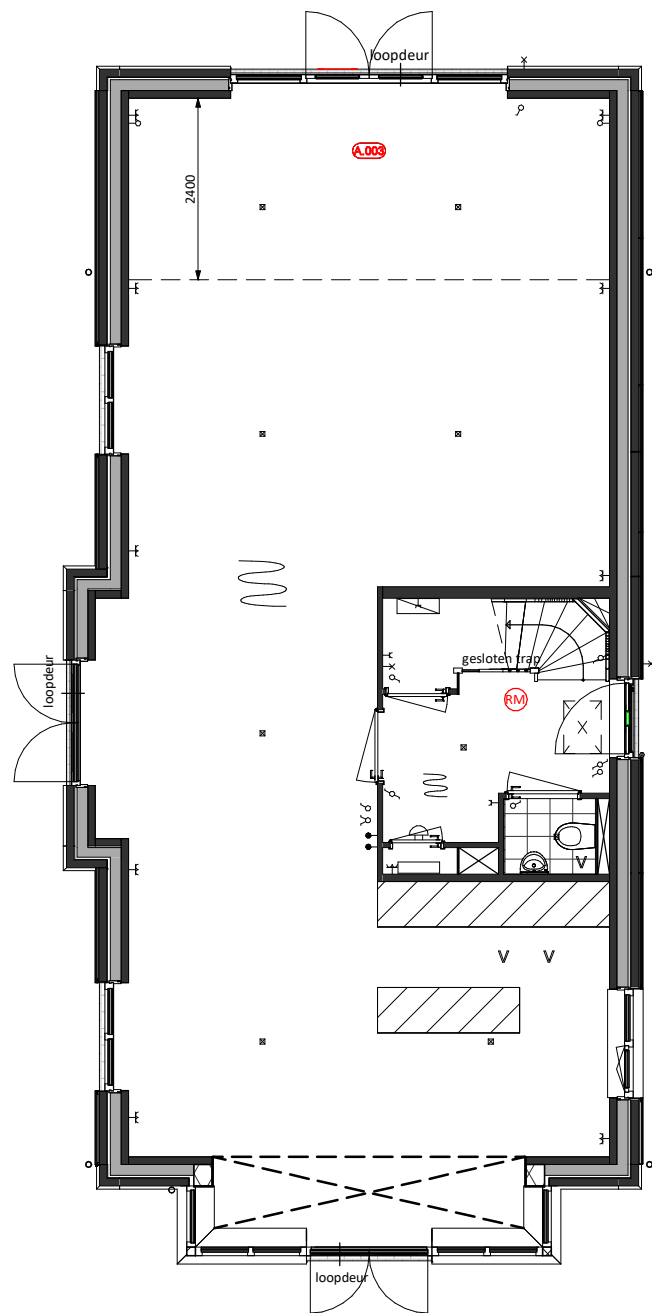
Begane grond A.003 = Uitbouw achtergevel 2.4m
