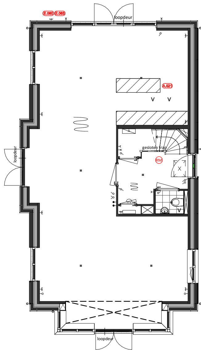
Begane grond A.021 = De keuken wordt naar de achterzijde van de woning geplaatst E.060 = Extra buitenlichtpunt E.063 = Dubbele WCD op achtergevel
