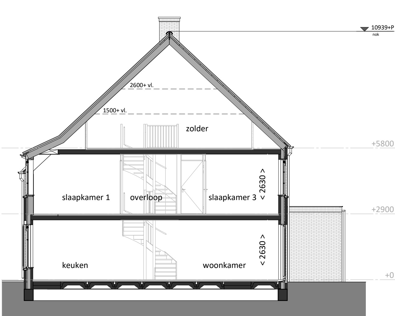
doorsnede schaal 1:100
