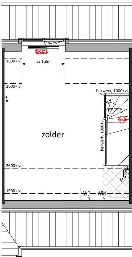
Tweede Verdieping DK.211 = Dakkapel ca.1,8m
