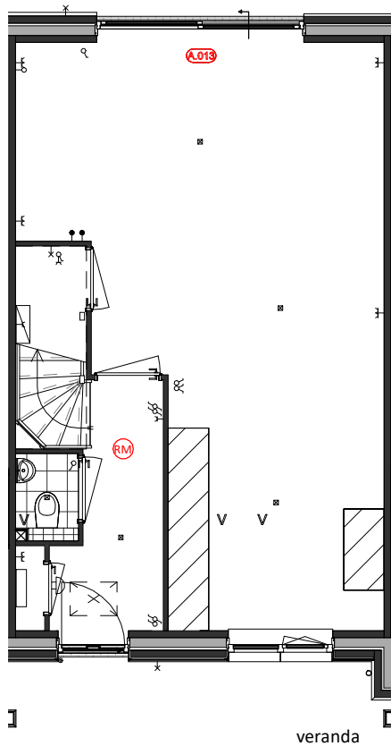
Begane Grond A.013 = Wijzigen schuivend deel schuipui of loopdeur
