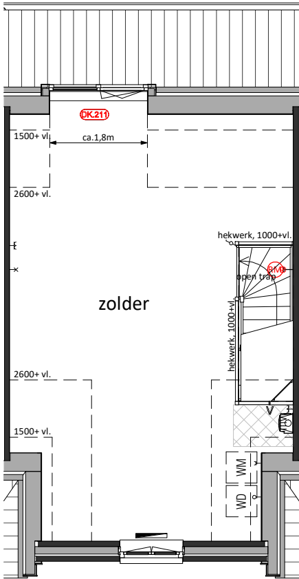
Tweede Verdieping DK.211 = Dakkapel ca.1,8m
