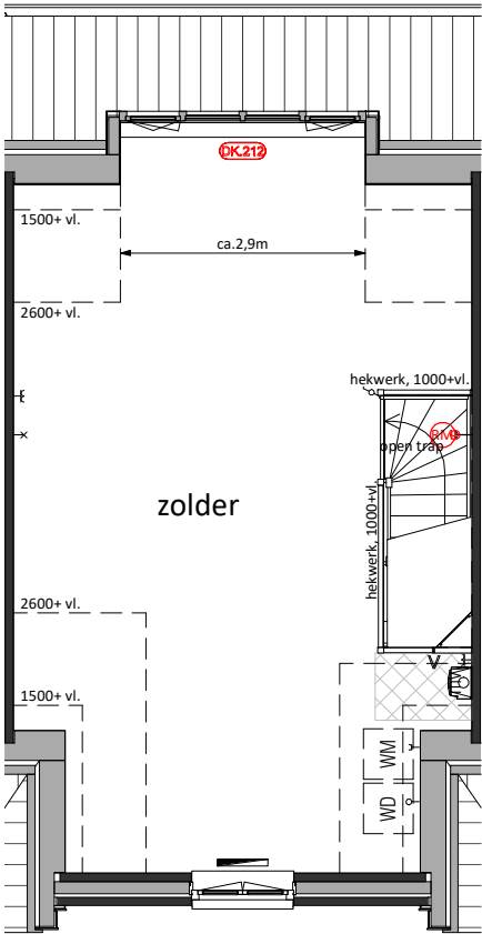
Tweede Verdieping DK.212 = Dakkapel ca.2,9m
