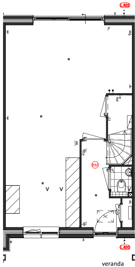
Begane Grond L.820 = Buitenkraan voorgevel L.822 = Buitenkraan achtergevel
