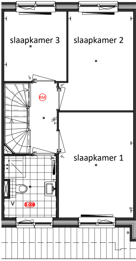
Eerste Verdieping S.009 = Verplaatsing toilet voorzijde schacht
