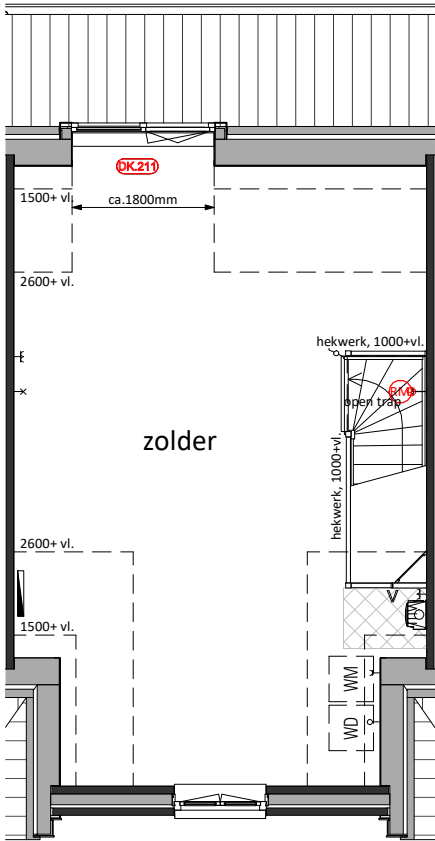
Tweede Verdieping DK.211 = Dakkapel ca.1800mm
