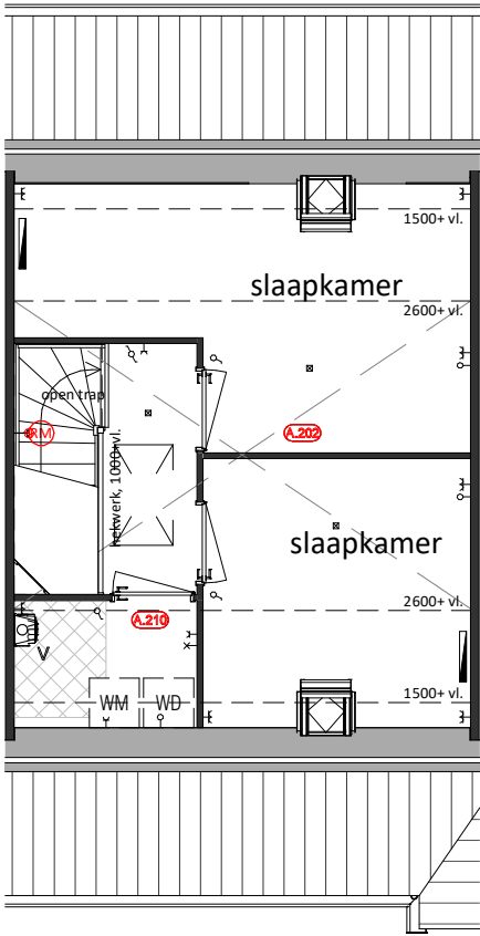
Tweede Verdieping A.202 = Zolderindeling met overloop en 2 slaapkamers A.206 = Afgesloten technische ruimte
