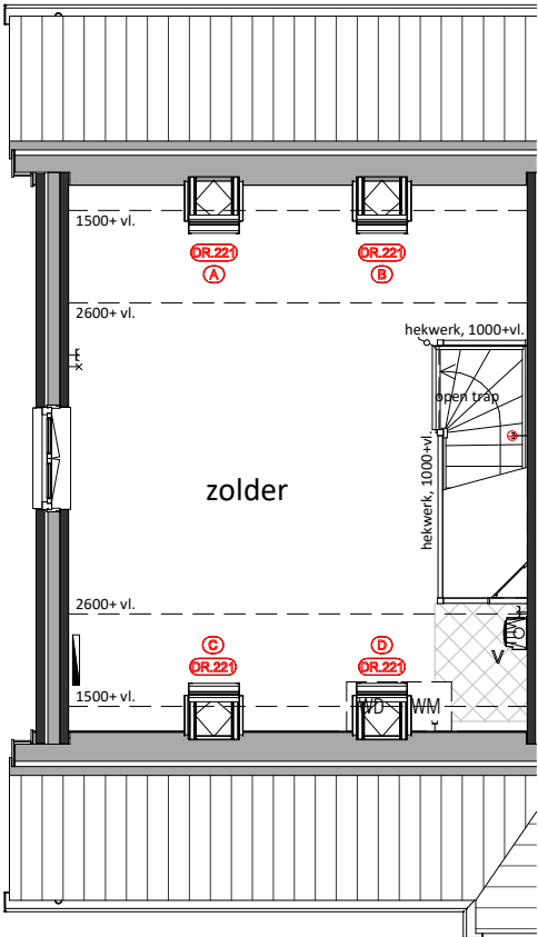
Tweede Verdieping DR.221 = Dakraam
