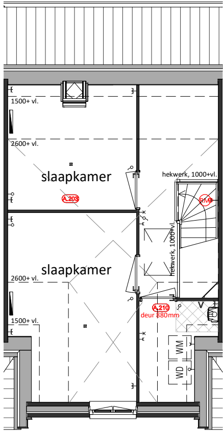
Tweede Verdieping A.203 = Zolderindeling met ruime overloop en 2 slaapkamers A.210 = Afgesloten technische ruimte
