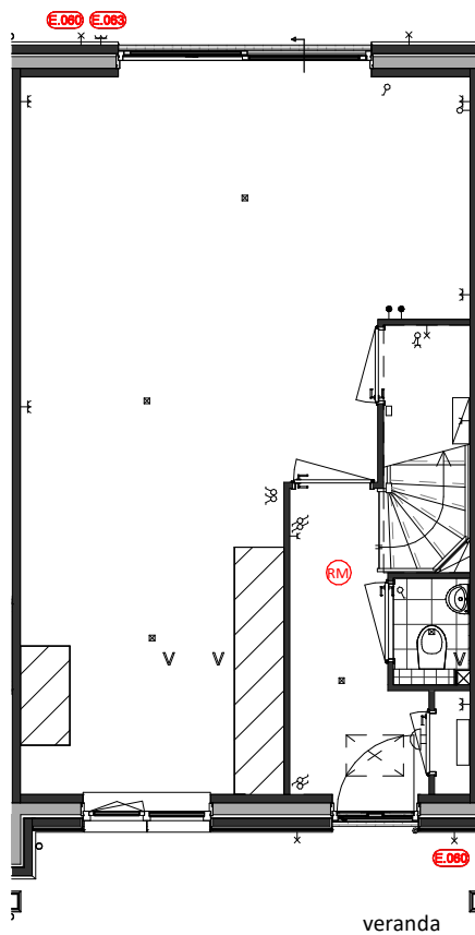
Begane Grond E.063 = Dubbele wcd op achtergevel E.060 = Extra buitenlichtpunt
