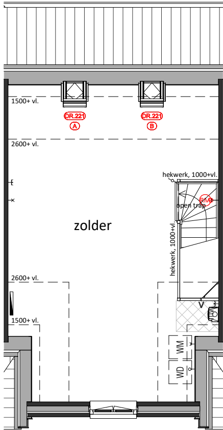
Tweede Verdieping DR.221 = Dakraam
