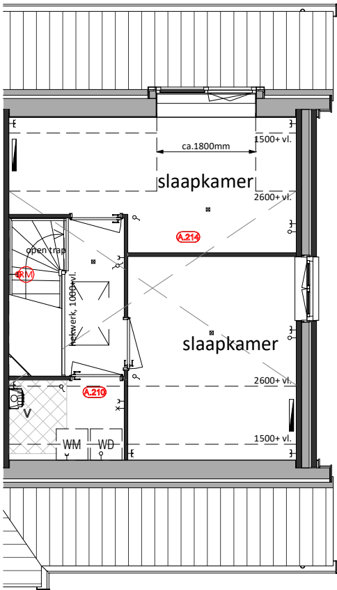
Tweede Verdieping A.214 = Upgrade van onbenoemde ruimte naar slaapkamer A.210 = Afgesloten technische ruimte
