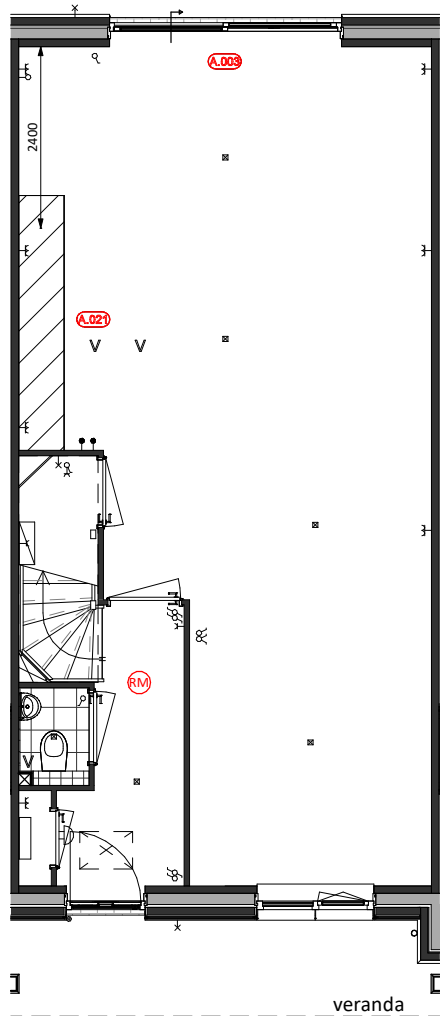
Begane Grond A.003 = Uitbouw achtergevel 2,4m A.021 = Keuken opstelling naar achtergevel (met A.001 of A.003)
