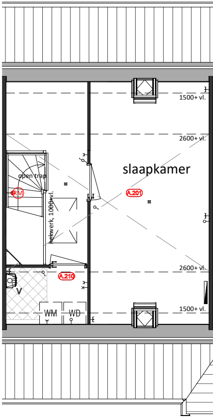
Tweede Verdieping A.201 = Zolderindeling met overloop en slaapkamer A.210 = Afgesloten technische ruimte
