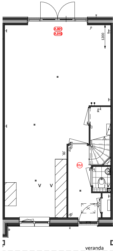
Begane Grond A.001 = Uitbouw achtergevel 1,2m A.010 = Openslaande deuren met zijlichten
