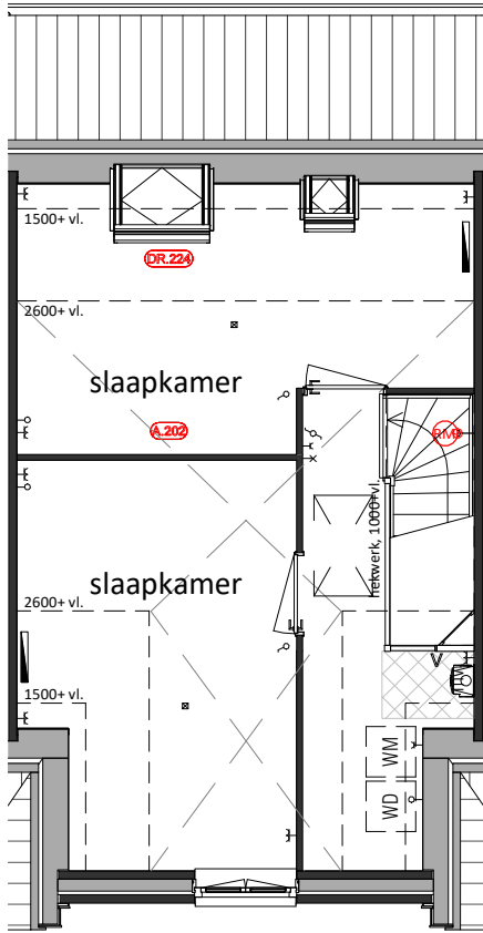
Tweede Verdieping A.202 = Zolderindeling met overloop en 2 slaapkamers DR.224 = Dakraam vergroten
