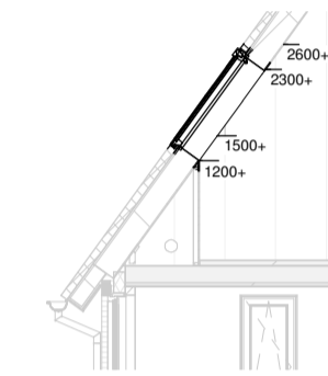
Doorsnede
