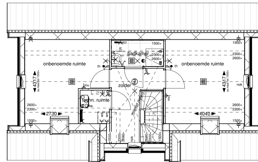
Tweede verdieping
