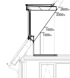
Doorsnede
