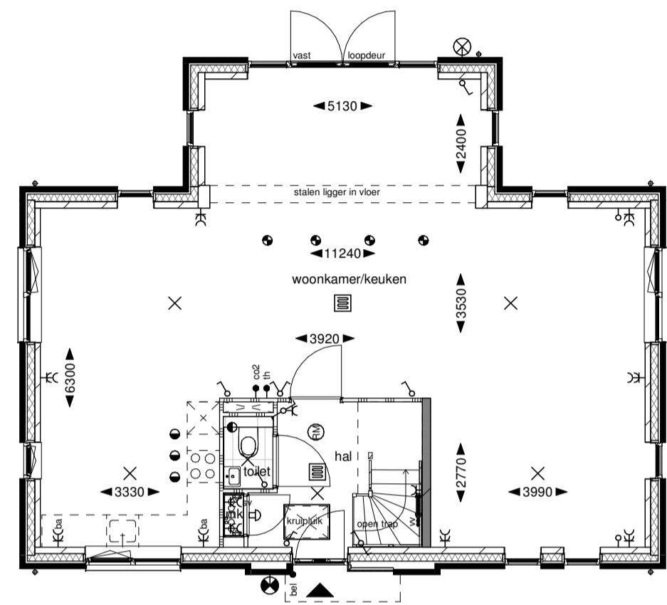
Begane grond
