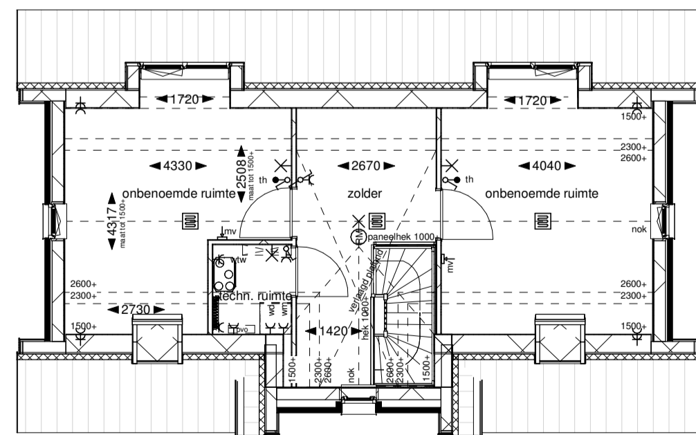
Tweede verdieping
