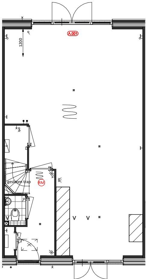
Begane Grond A.001 = Uitbouw achtergevel 1,2m
