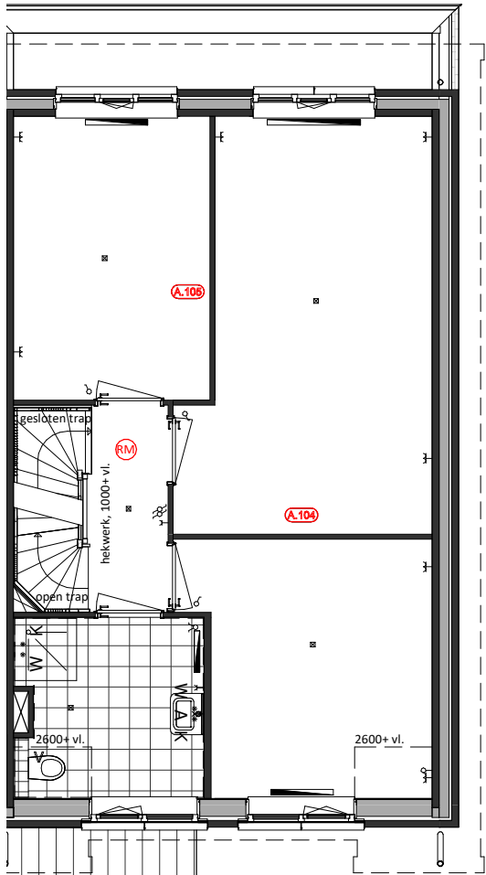
Eerste Verdieping A.104 = Scheidingwand verplaatsen 700mm A.105 = Scheidingwand verplaatsen 200mm
