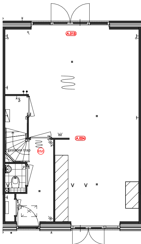
Begane Grond A.013 = Wijziging schuifvenddeel schuifpui of loopdeur A.024 = kopse wand tpv. keuken
