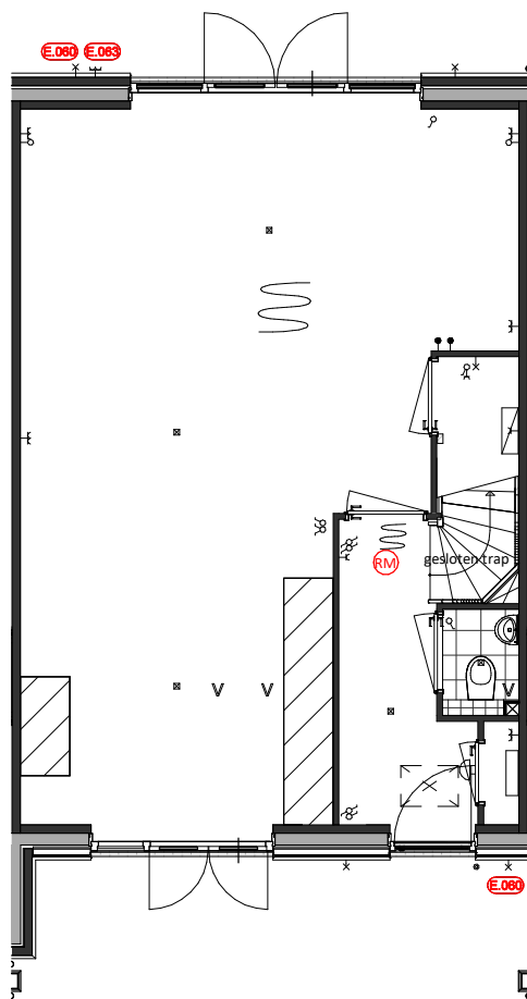
Begane Grond E.060 = Dubbele wcd op achtergevel E.063 = Extra buitenlichtpunt
