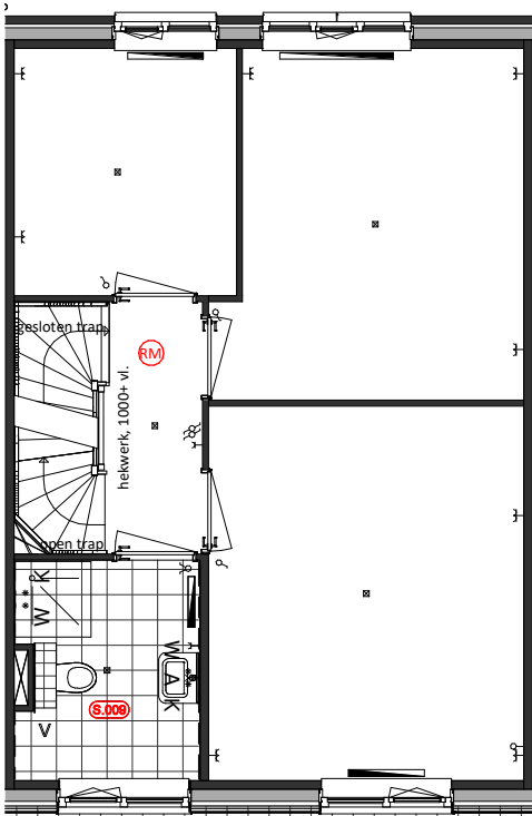
Eerste Verdieping A.106 = Slaapkamers achterzijde samenvoegen S.007 = Bad in badkamer (alleen met optie S.009) (draaistand raam vastzetten)
