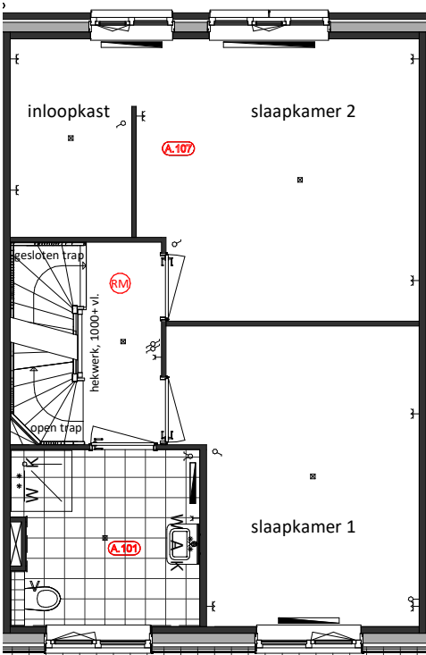
Eerste Verdieping Basis
