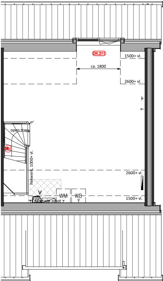
Tweede Verdieping DK.211 = Dakkapel ca.1800mm
