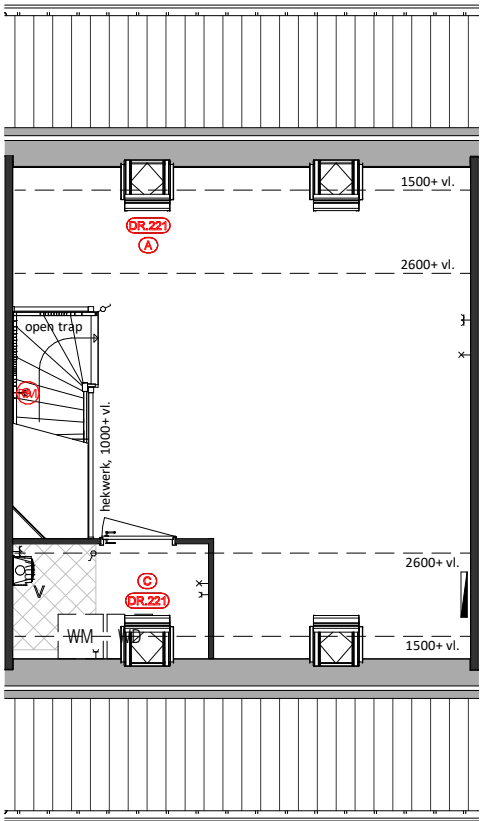
Tweede Verdieping DR.221 = Dakraam
