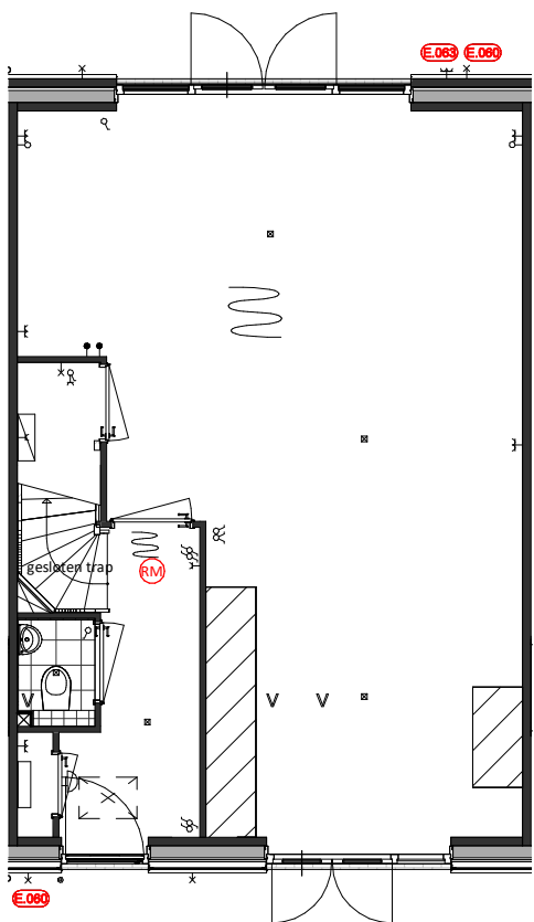
Begane Grond A.003 = Uitbouw achtergevel 2,4m A.021 = Keuken opstelling naar achtergevel (met A.001 of A.003)
