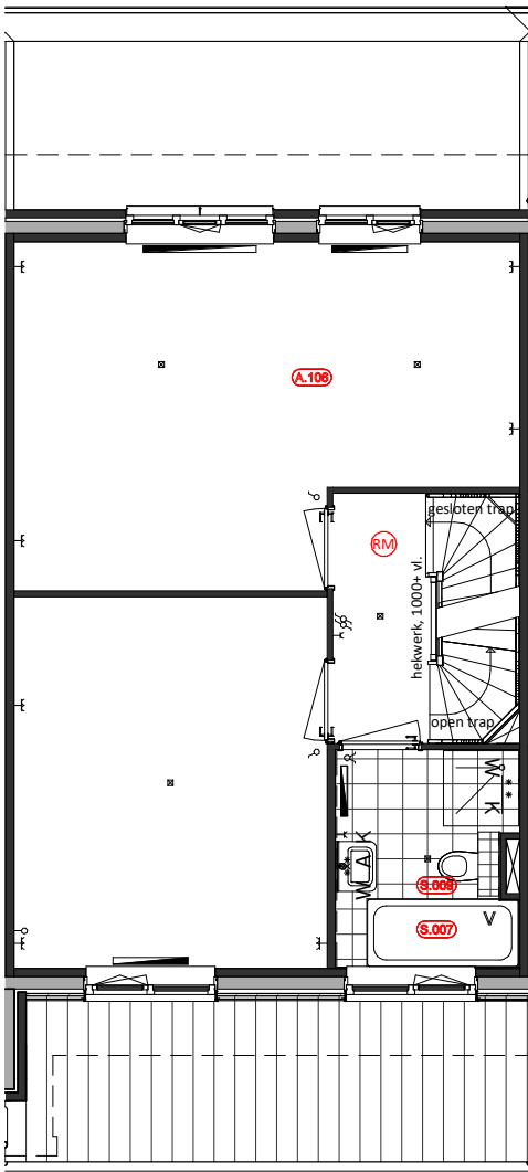
Eerste Verdieping A.106 = Slaapkamers achterzijde samenvoegen S.007 = Bad in badkamer (alleen met optie S.009) (draaistand raam vastzetten)
