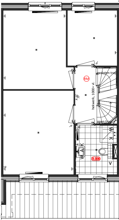
Eerste Verdieping S.009 = Verplaatsing toilet voorzijde schacht
