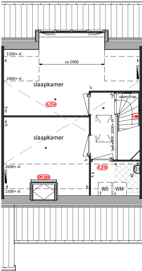
Tweede Verdieping A.214 = Upgrade van onbenoemde ruimte naar slaapkamer A.210 = Afgesloten technische ruimte DR.224 = Dakraam vergroten
