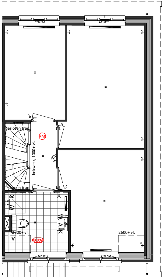
Eerste Verdieping S.009 = Verplaatsing toilet voorzijde schacht
