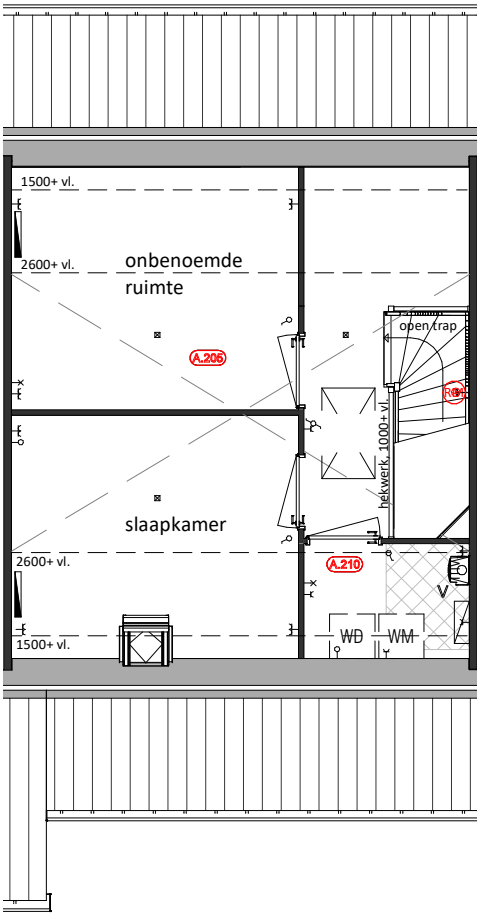
Tweede Verdieping A.205 = Zolderindeling met overloop, slaapkamer en onbenoemde ruimte A.210 = Afgesloten technische ruimte
