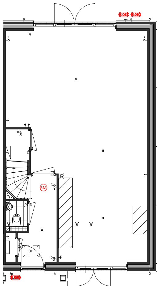
Begane Grond E.063 = Dubbele wcd op achtergevel E.060 = Extra buitenlichtpunt
