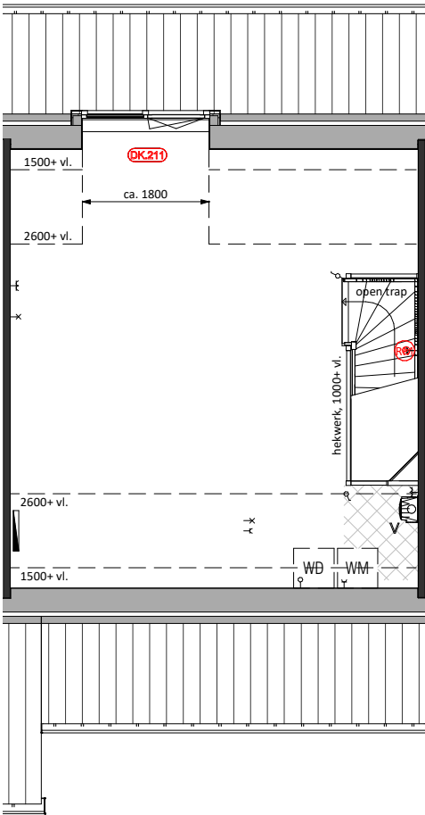
Tweede Verdieping DK.211 = Dakkapel ca.1800mm
