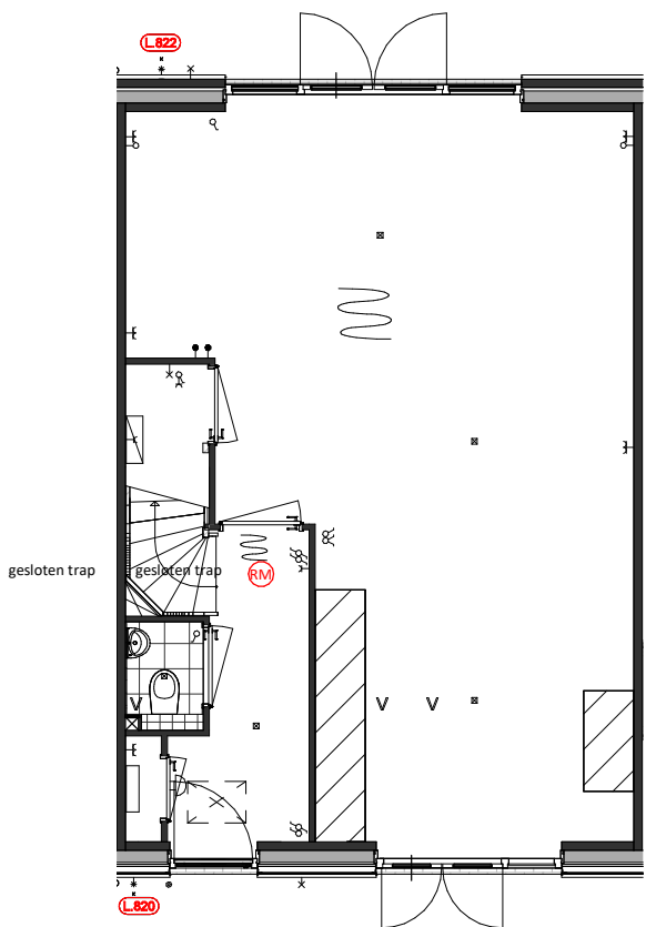
Begane Grond L.820 = Buitenkraan voorgevel L.822 = Buitenkraan achtergevel
