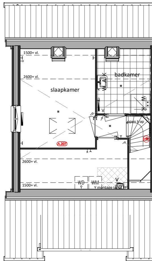
Tweede Verdieping A.207 = Zolderindeling met overloop, slaapkamer en badkamer A.210 = Afgesloten technische ruimte
