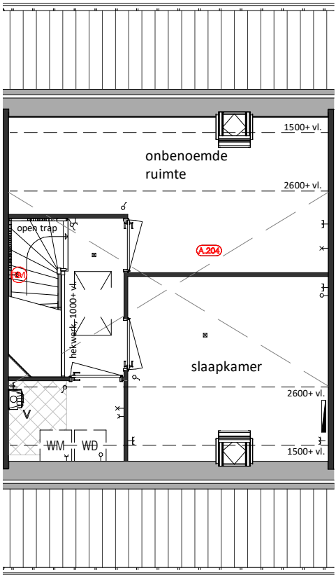
Tweede Verdieping A.204 = Zolderindeling met overloop, slaapkamer en badkamer A.210 = Afgesloten technische ruimte
