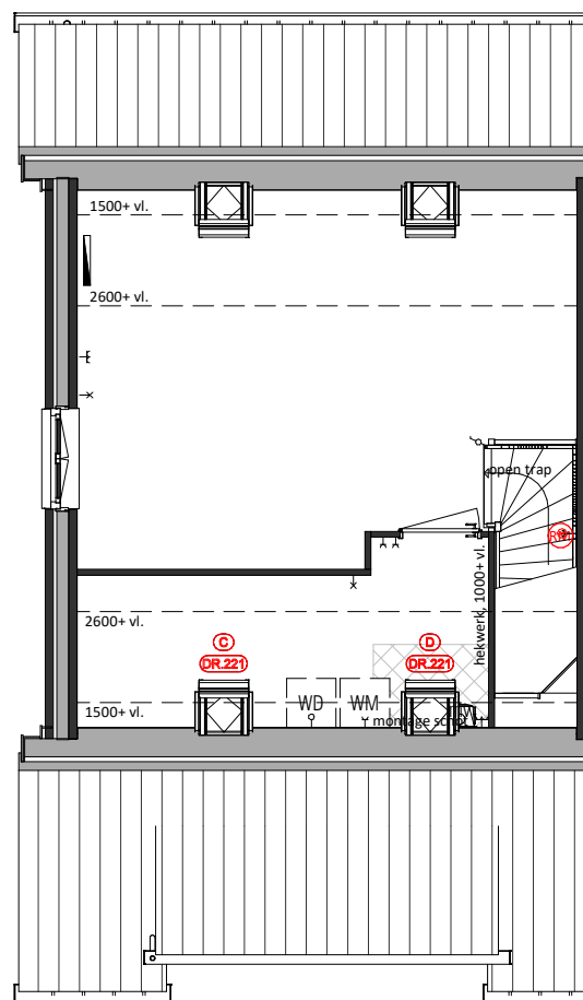
Tweede Verdieping DK.221 = Dakraam
