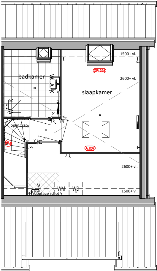
Tweede Verdieping A.207 = Zolderindeling met overloop, slaapkamer en badkamer A.210 = Afgesloten technische ruimte DR.224 = Dakraam vergroten
