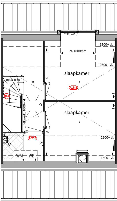
Tweede Verdieping A.213 = Upgrade van onbenoemde ruimte naar slaapkamer A.210 = Afgesloten technische ruimte
