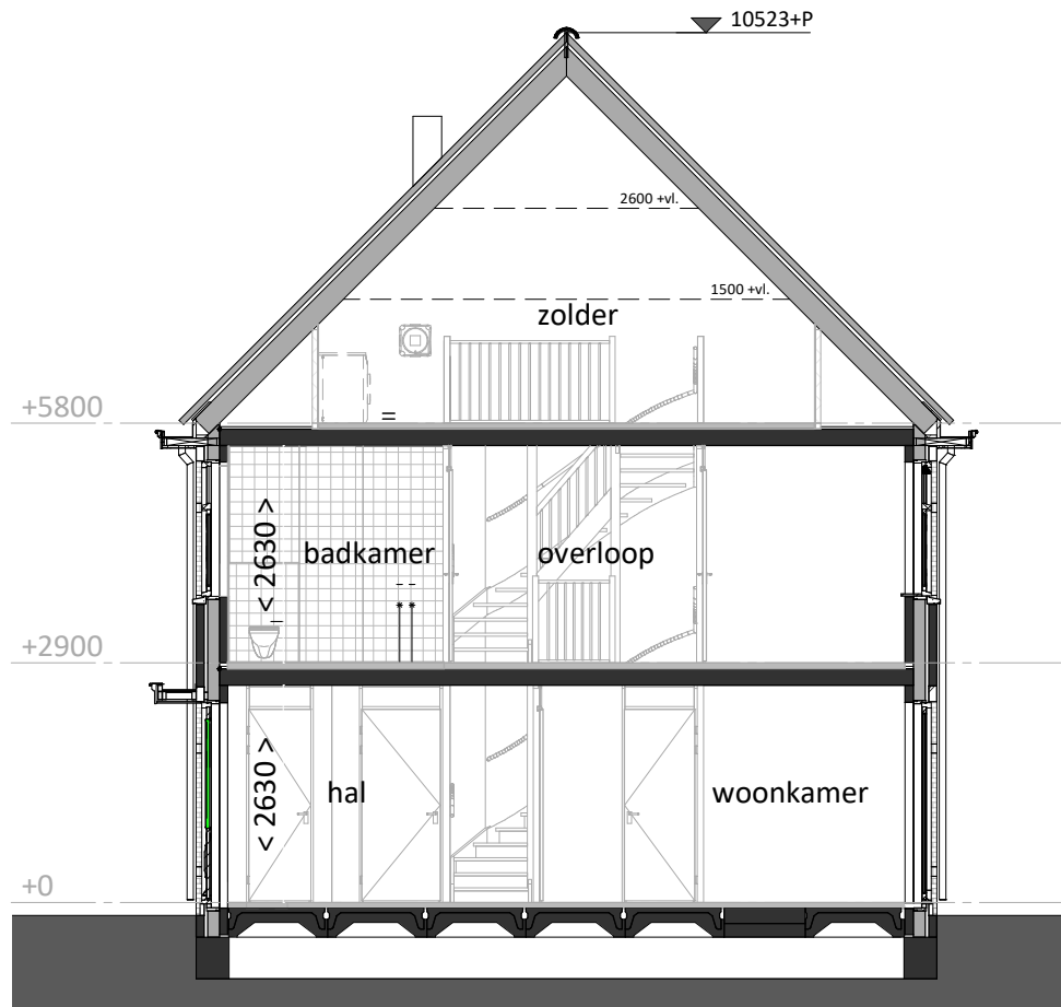
doorsnede schaal 1:100
