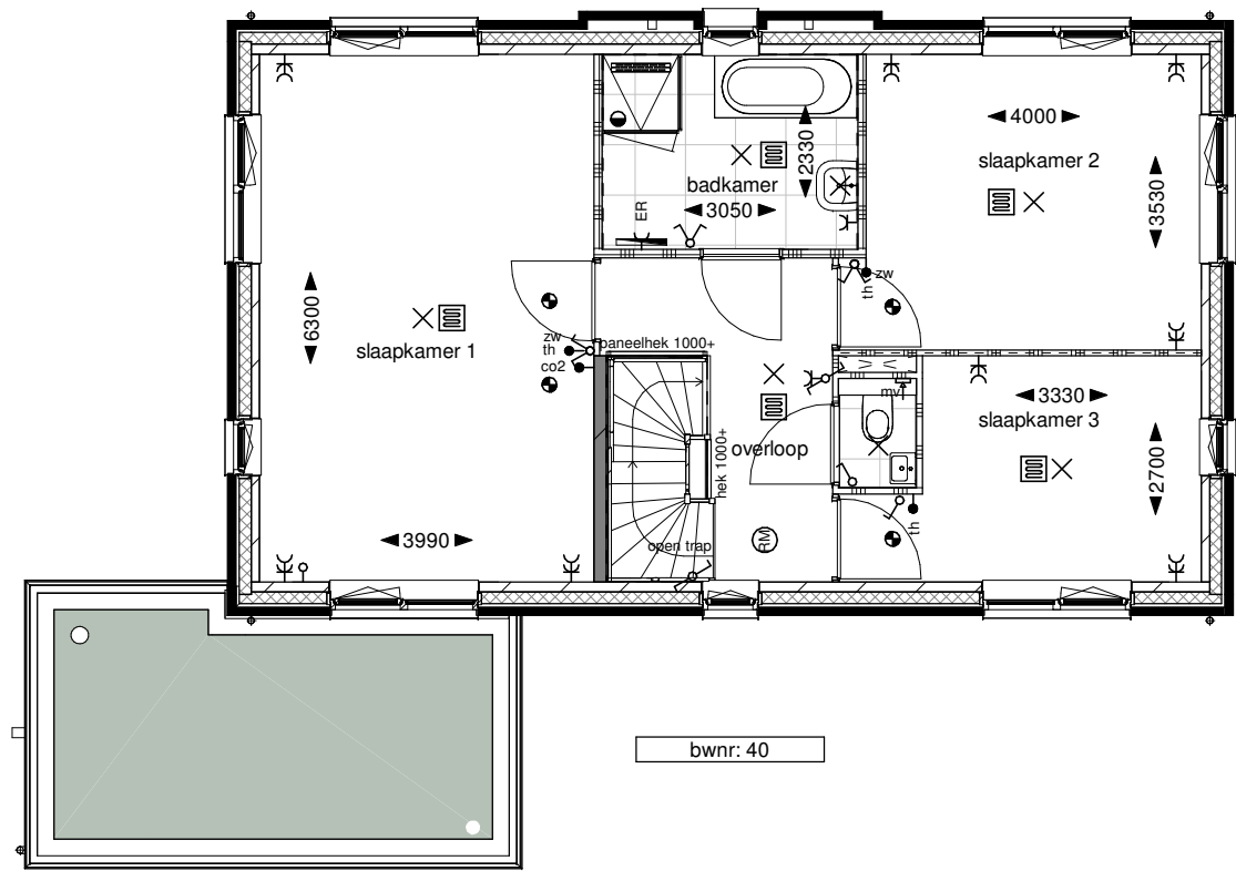
Eerste verdieping
