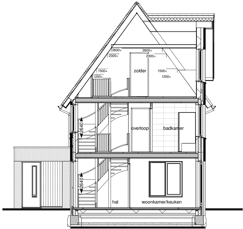
Doorsnede A
