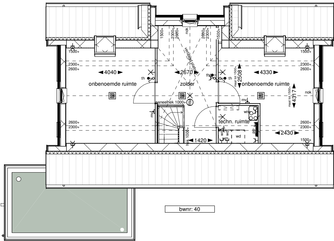
Tweede verdieping
