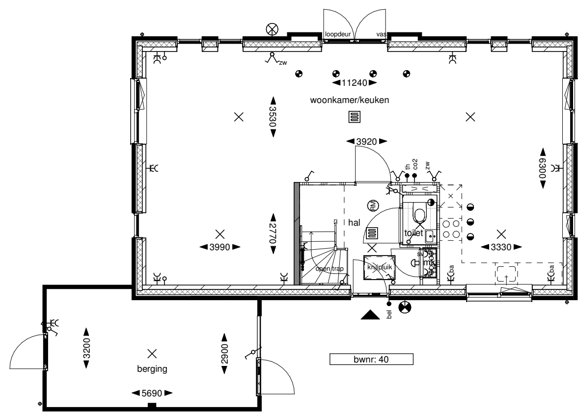
Begane grond
