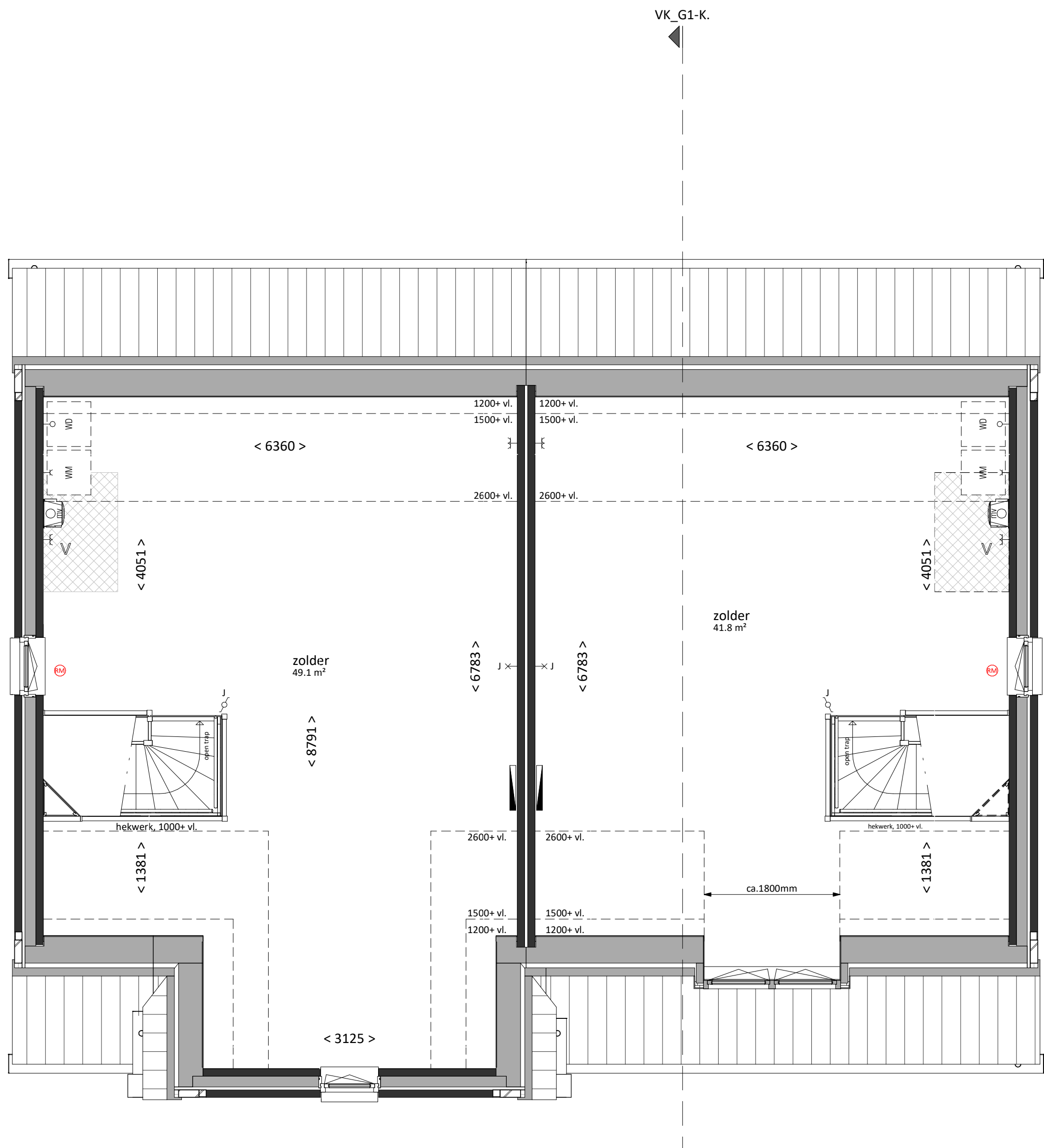
tweede verdieping bk. vloer = 5800+ schaal 1:50
