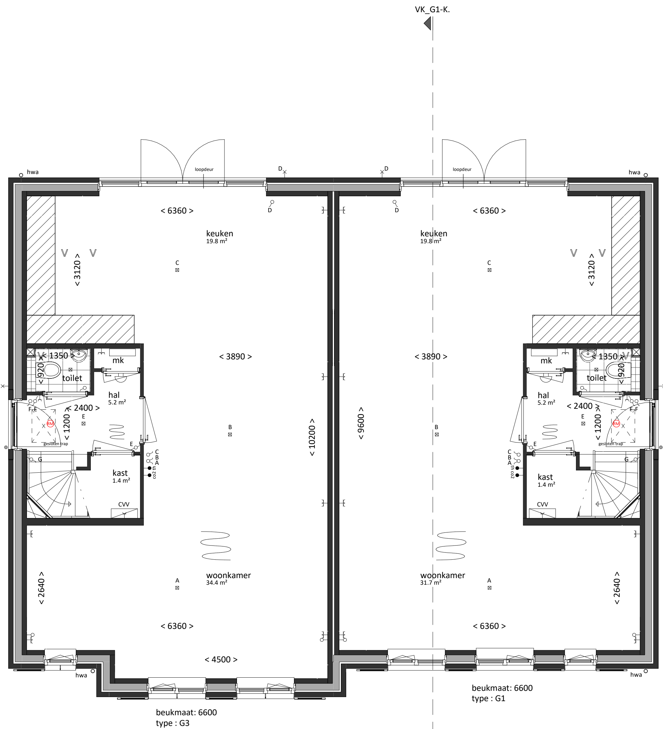
begane grond bk. vloer = P = 0 schaal 1:50
