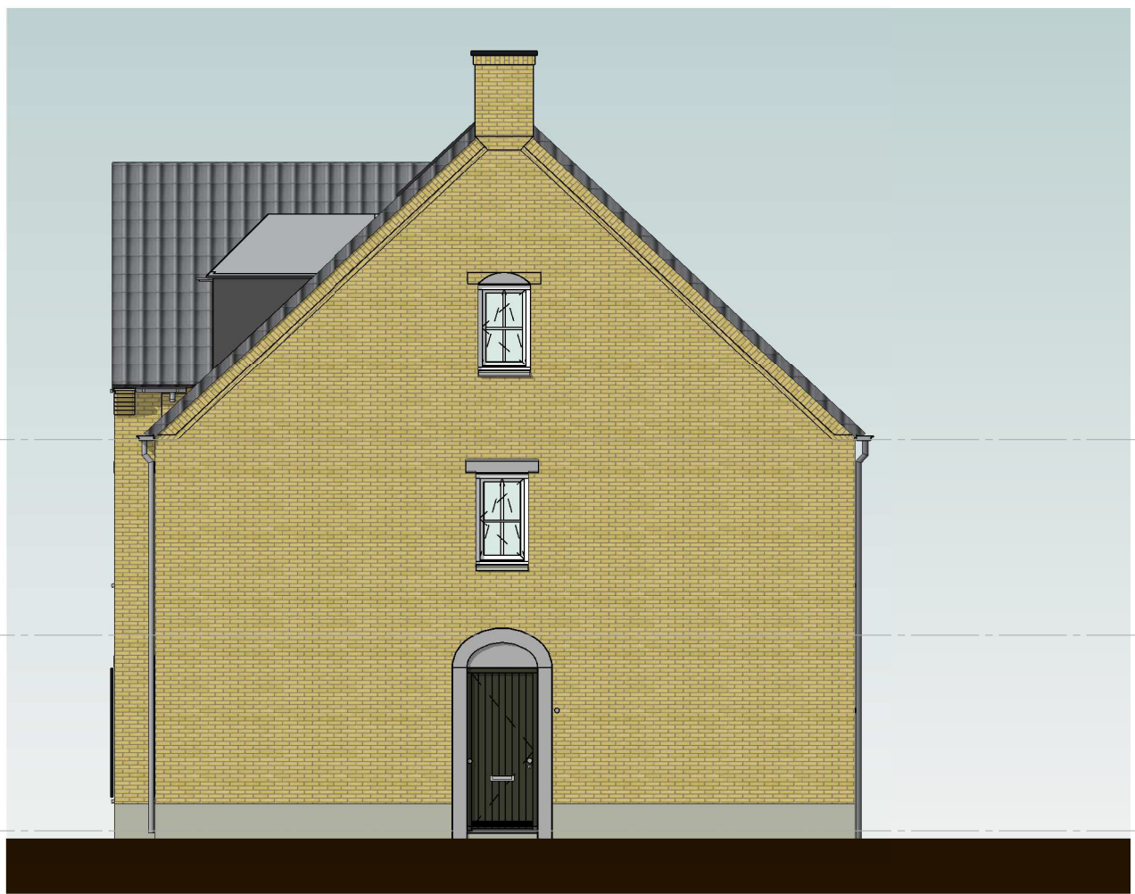
rechttergevel schaal 1:100
