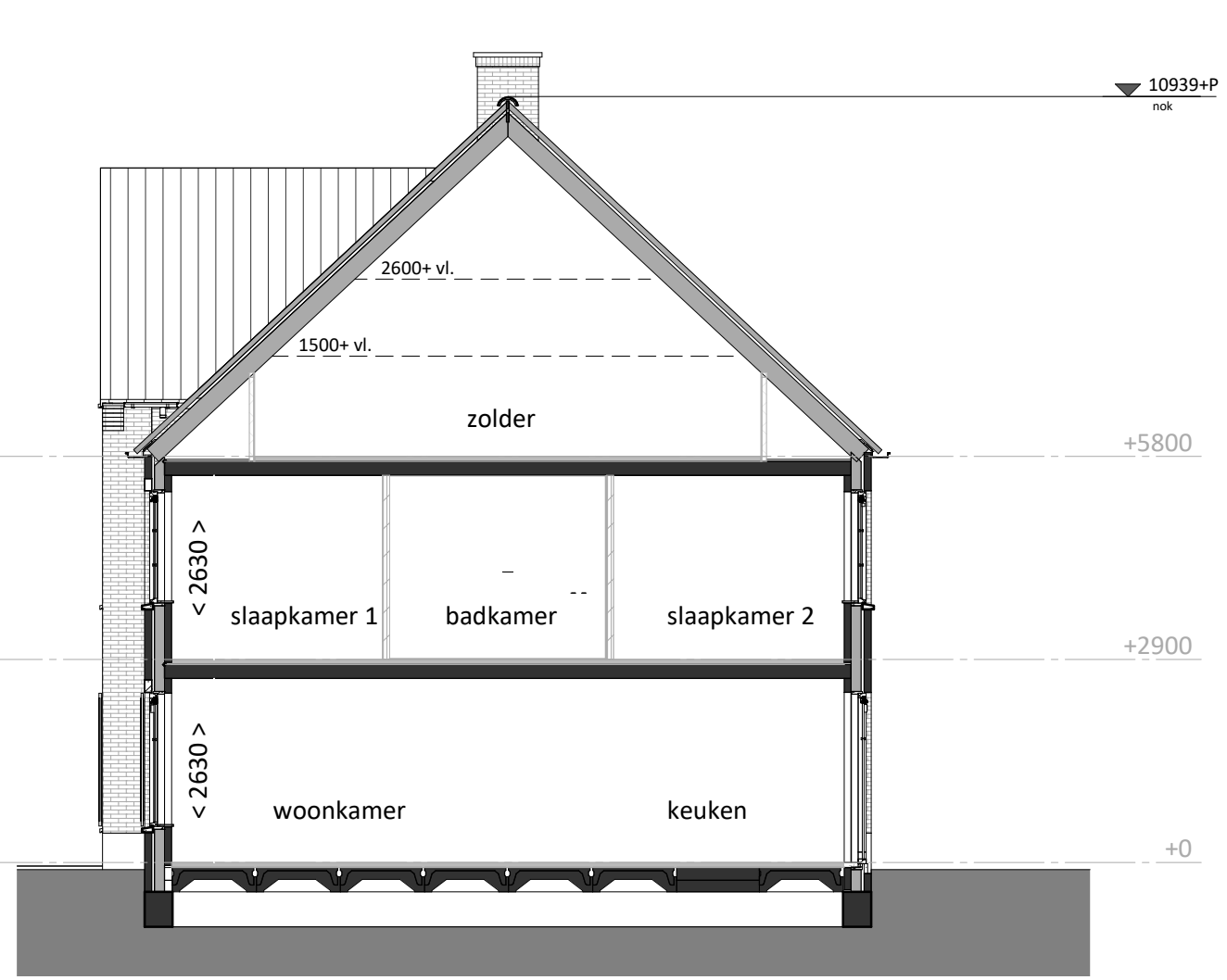
doorsnede schaal 1:100
