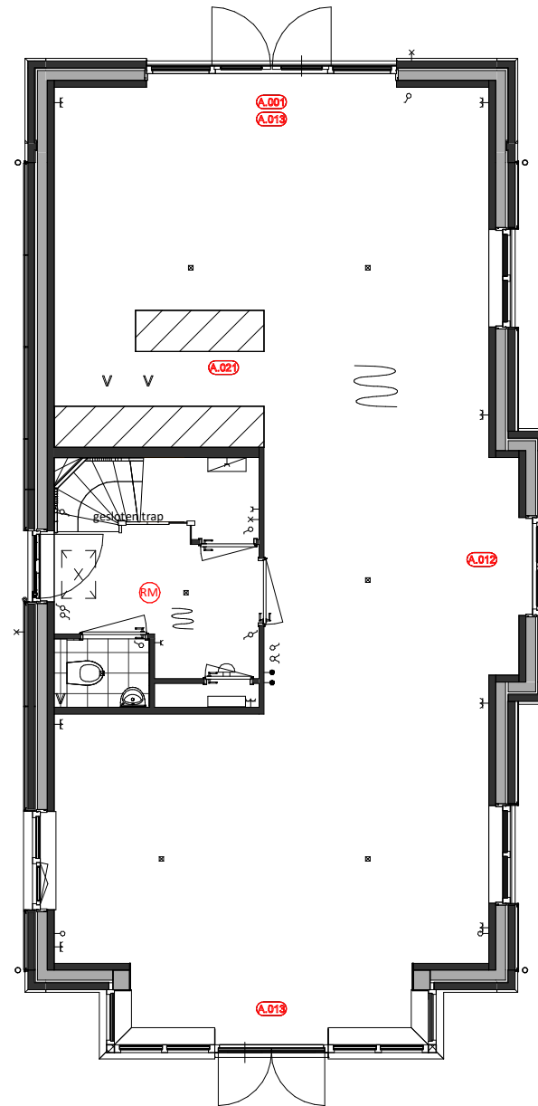
Begane Grond A.001 = Uitbouw achtergevel 1,2m A.009 = Keuken opstelling naar achtergevel (met A.001 of A.003) A.012 = Draairichting naar buiten A.013 = Wijzigen loopdeur
