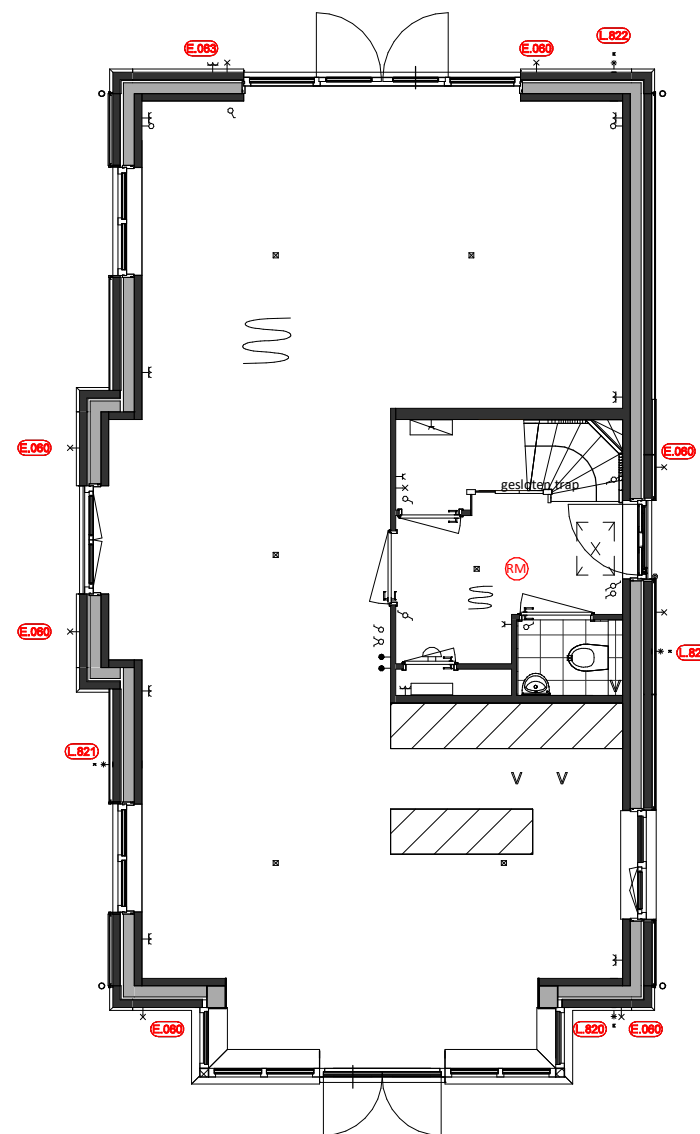
Begane Grond L.820 = Buitenkraan voorgevel L.821 = Buitenkraan zijgevel L.822 = Buitenkraan achtergevel E.060 = Extra buitenlichtpunt E.063 = Dubbele wcd op achtergevel
