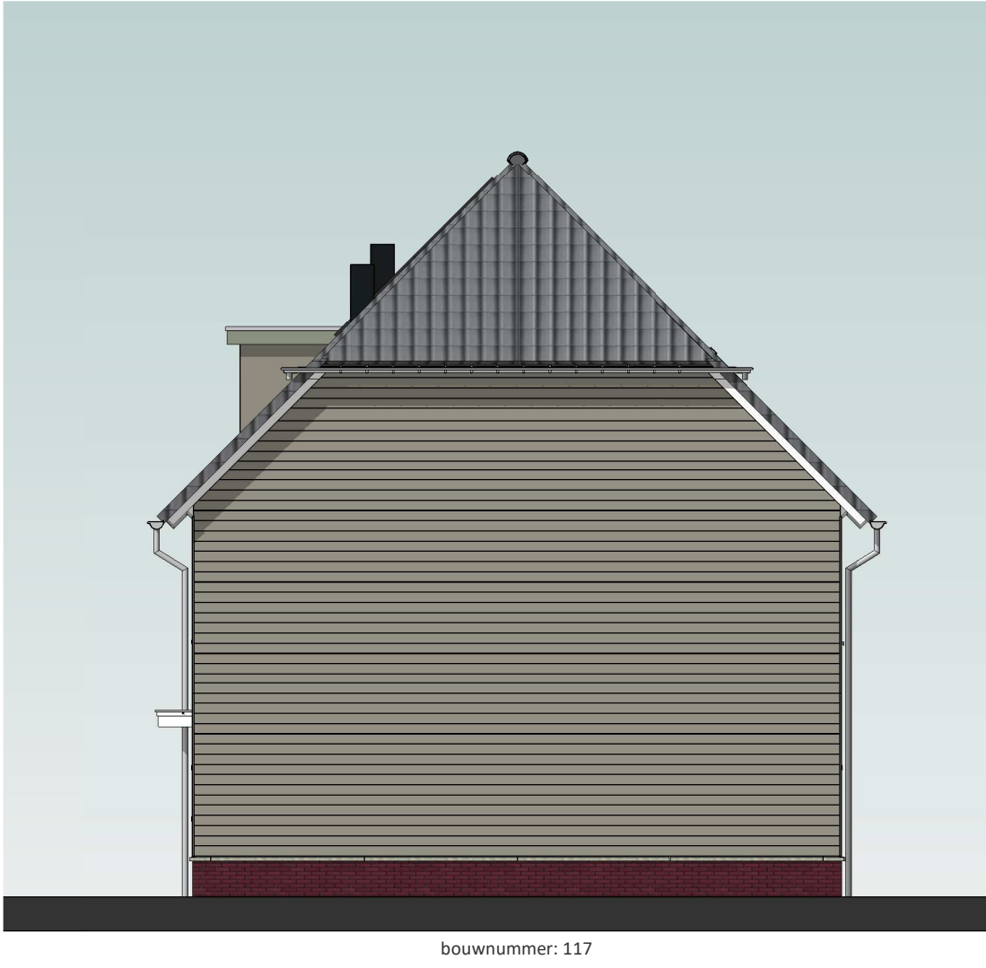
rechtegevel orientatie: oost schaal 1:100
