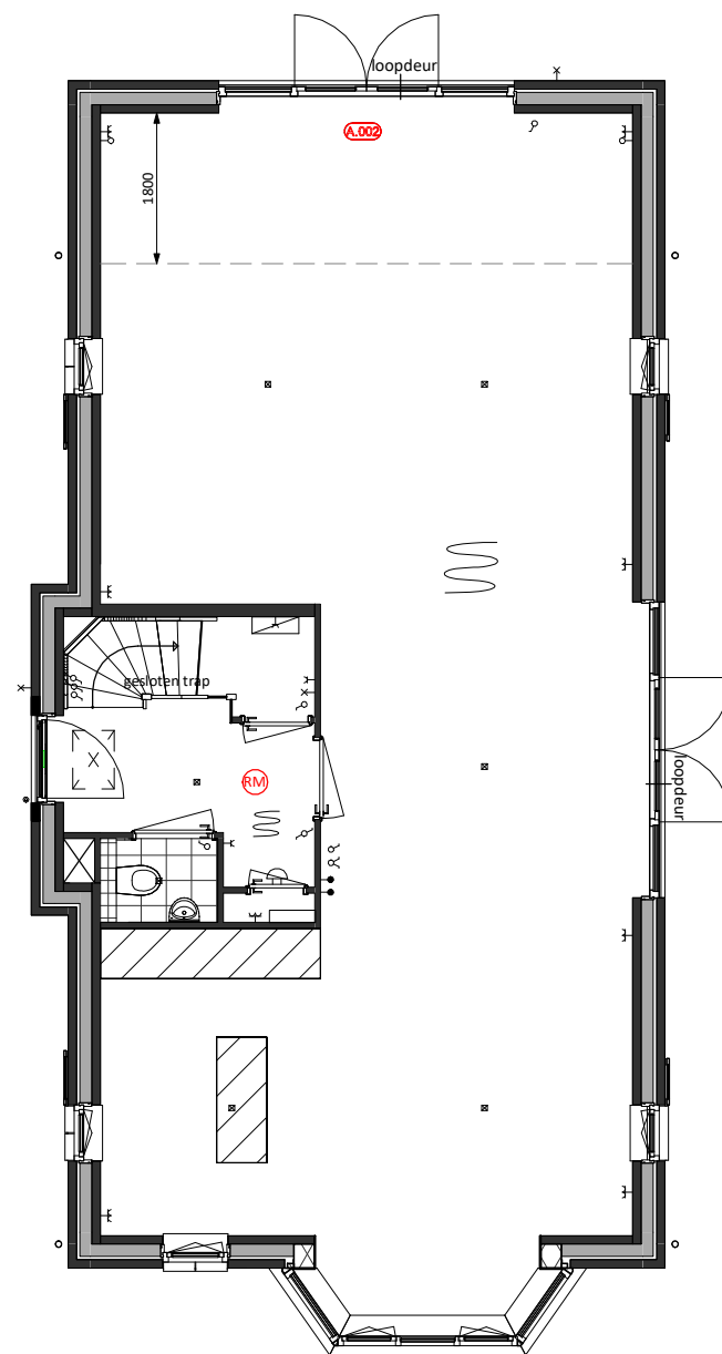
Begane grond A.002 = Uitbouw achtergevel 1.8m
