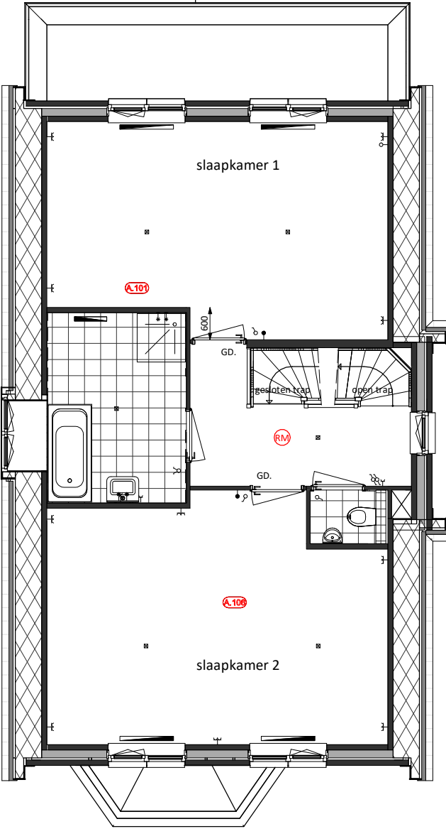
Eerste verdieping A.101 = Badkamer vergroot 600mm A.106 = Slaapkamers voorzijde samenvoegen
