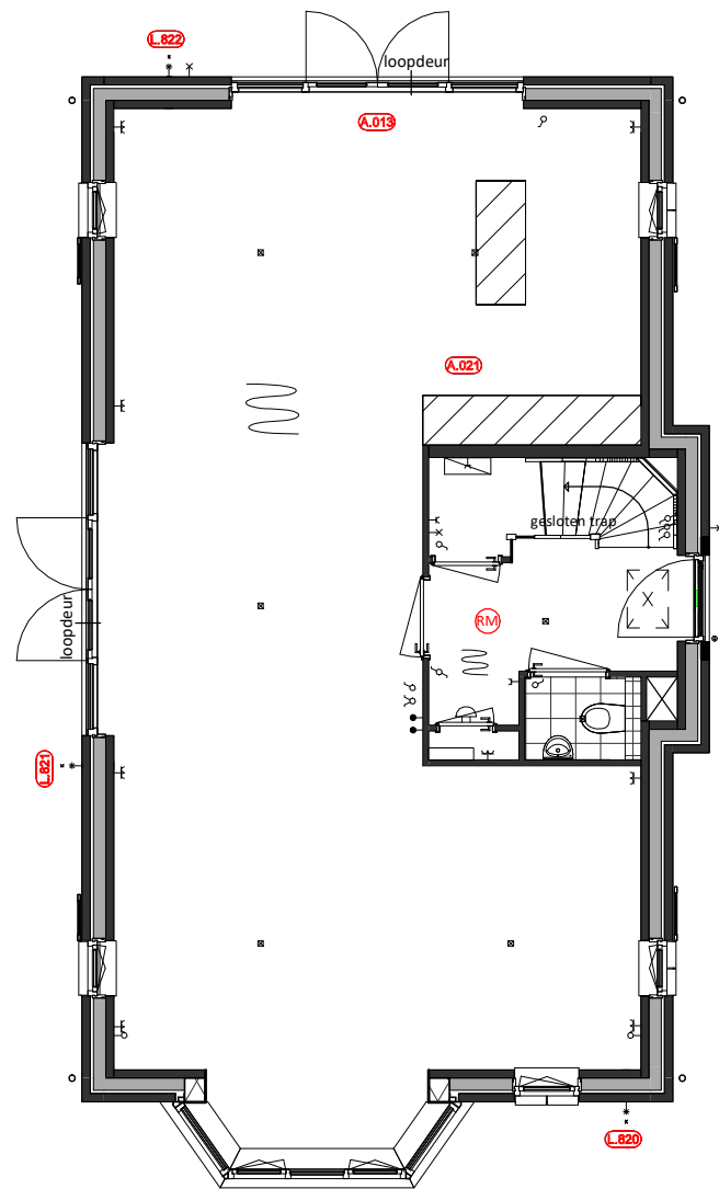
Begane grond A.021 = Keuken naar achterzijde woning L.820 = Buitenkraan voorgevel L.821 = Buitenkraan zijgevel L.822 = Buitenkraan achtergevel A.013 = Wijzigen schuivend deel schuifpui of loopdeur
