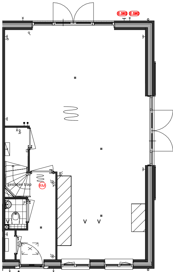
Begane Grond E.063 = Dubbele wcd op achtergevel E.060 = Extra buitenlichtpunt
