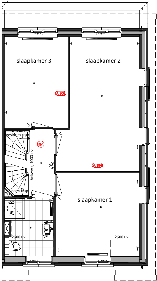
Eerste Verdieping A.104 = Scheidingswand verplaatsen 700mm A.105 = Scheidingswand verplaatsen 200mm
