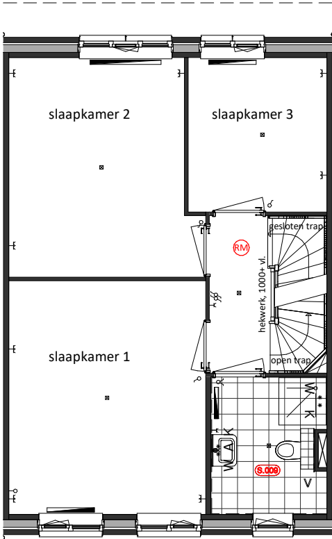
Eerste Verdieping A.106 = Slaapkamers achterzijde samenvoegen S.007 = Bad in badkamer (alleen met optie S.009) (draaistand raam vastzetten)
