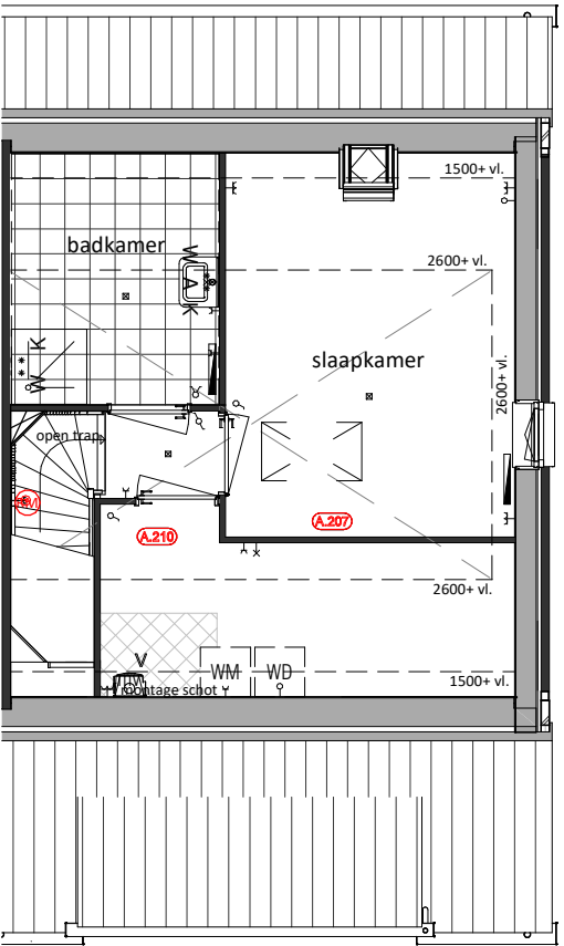
Tweede Verdieping A.207 = Zolderindeling met overloop, slaapkamer en badkamer A.210 = Afgesloten technische ruimte DR.224 = Dakraam vergroten
