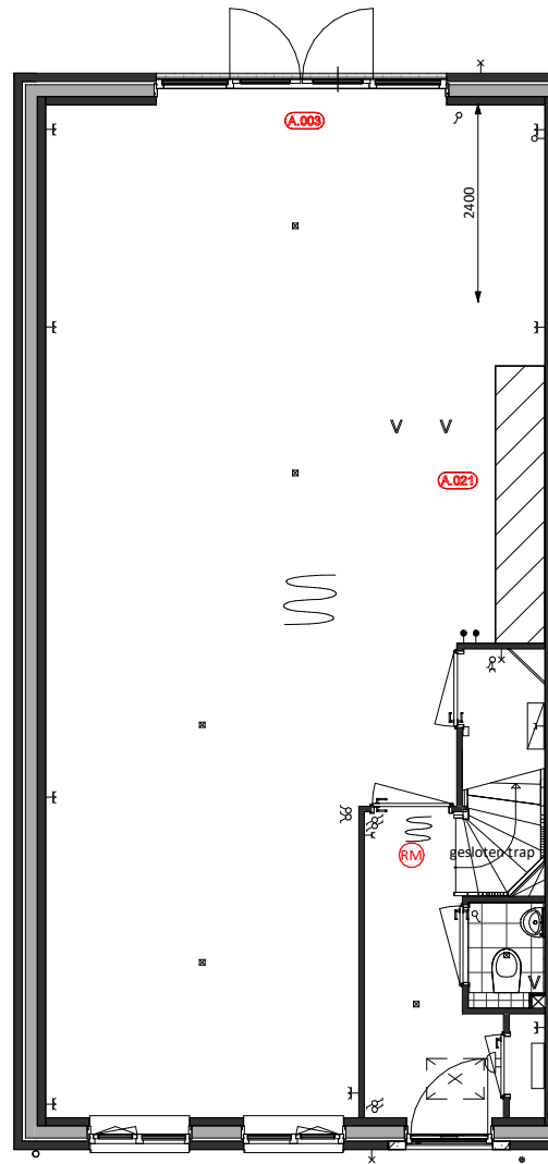
Begane Grond A.003= Uitbouw achtergevel 2,4m A.021 = Keuken opstelling naar achtergevel (met A.001 of A.003)
