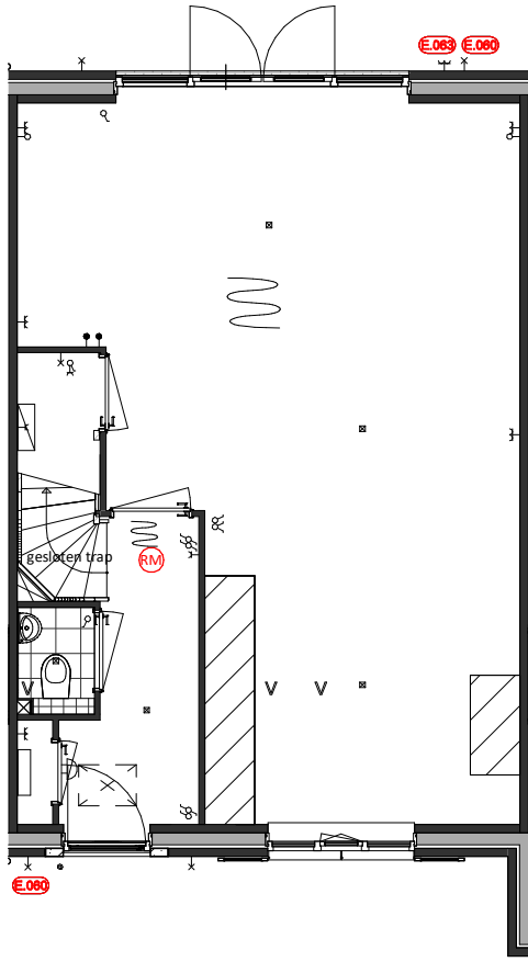
Begane Grond E.063 = Dubbele wjd op achtergevel E.060 = Extra buitenlichtpunt
