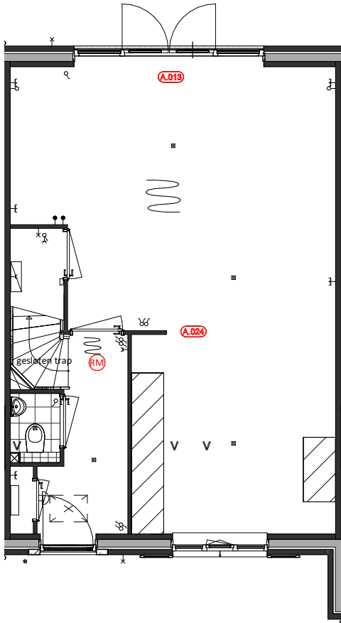
Begane Grond A.013 = Wijzigen schuifdeel schuifpui of loopdeur A.024 = kopse wand tpv. keuken
