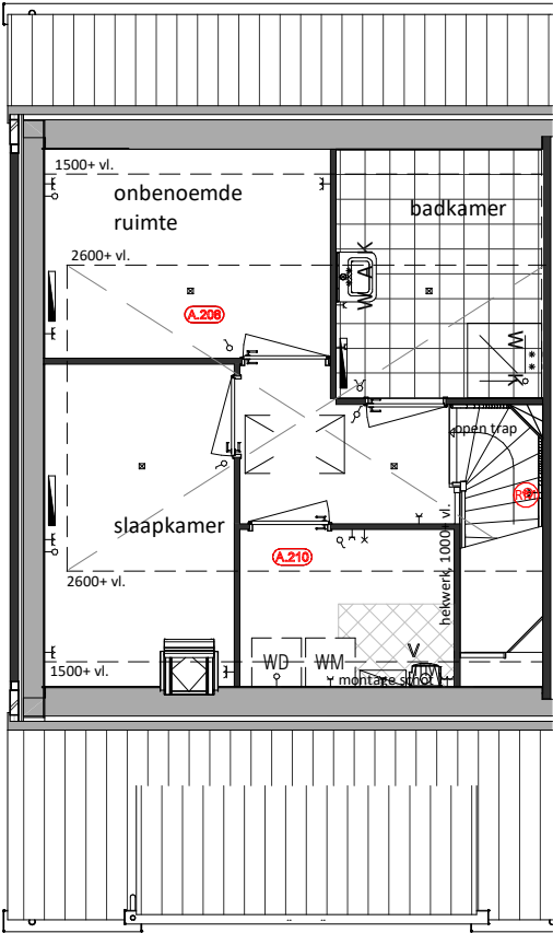
Tweede Verdieping A.208 = Zolderindeling met overloop, slaapkamers en badkamer A.210 = Afgesloten technische ruimte
