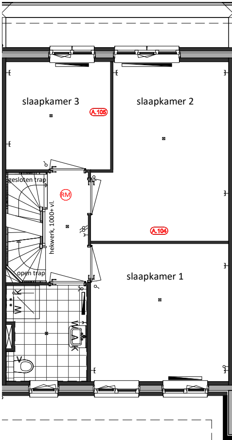
Eerste Verdieping A.104 = Scheidingswand verplaatsen 700mm A.105 = Scheidingswand verplaatsen 200mm
