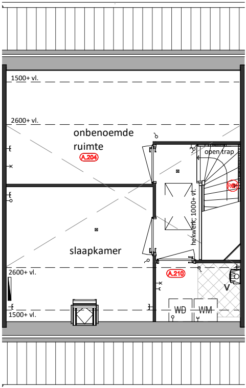
Tweede Verdieping A.204 = Zolderindeling met overloop, slaapkamer en onbenoemde ruimte A.210 = Afgesloten technische ruimte
