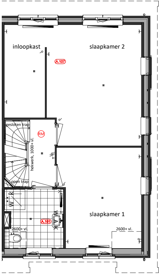
Eerste Verdieping A.107 = Masterbedroom met inloopkast achterzijde woning A.101 = Badkamer verbreden met 600mm
