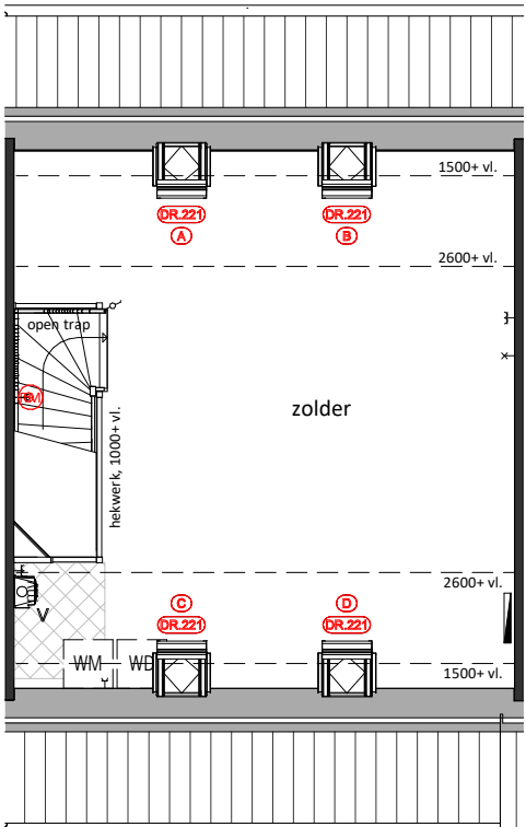
Tweede Verdieping DR.221 = Dakraam
