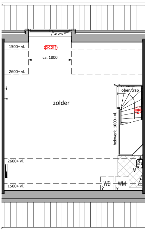
Tweede Verdieping DK.211 = Dakkapel ca.1800mm
