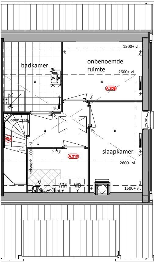
Tweede Verdieping A.208 = Zolderindeling met overloop, slaapkamers en badkamer A.210 = Afgesloten technische ruimte
