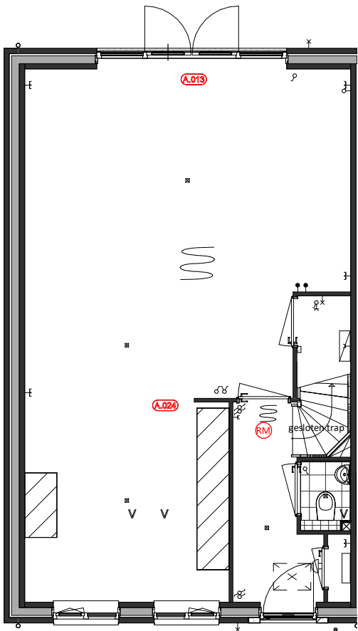
Begane Grond A.013 = Wijzigen schuifenddeel schuifpui of loopdeur A.024 = kopse wand tpv. keuken
