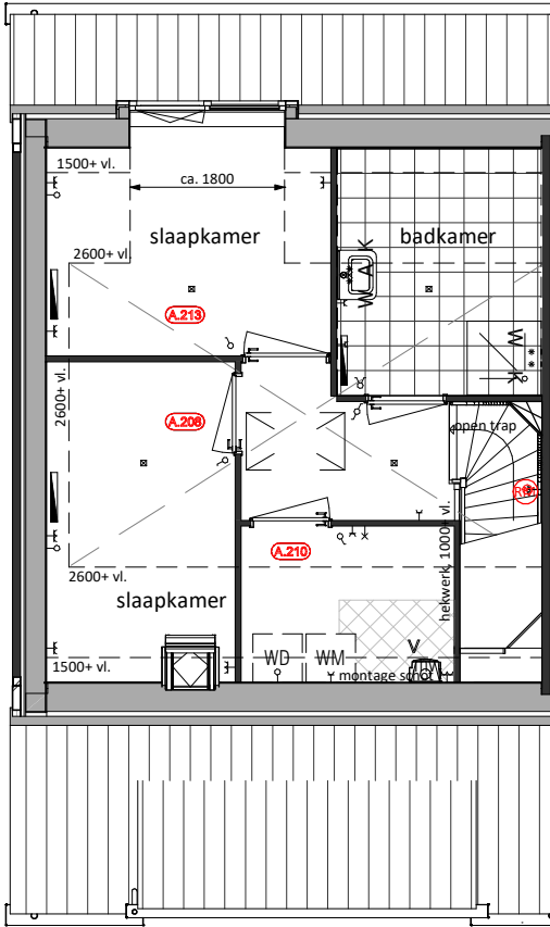
Tweede Verdieping A.208 = Zolderindeling met overloop, slaapkamers en badkamer A.210 = Afgesloten technische ruimte A.213 = Upgrade van onbenoemde ruimte naar slaapkamer
