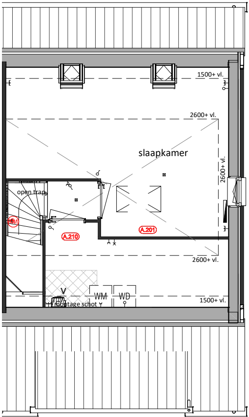
Tweede Verdieping A.201 = Zolderindeling met overloop en slaapkamer A.206 = Afgesloten technische ruimte
