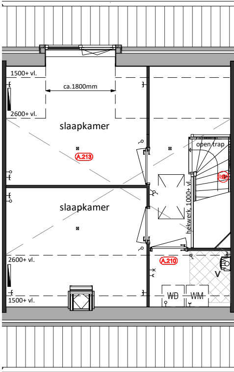
Tweede Verdieping A.213 = Upgrade van onbenoemde ruimte naar slaapkamer A.210 = Afgesloten technische ruimte
