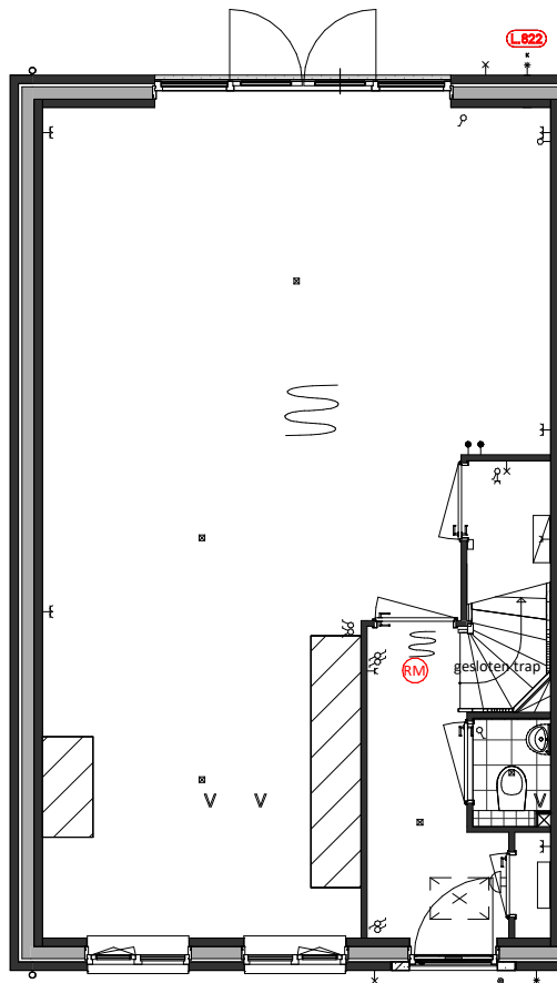
Begane Grond L.820 = Buitenkraan voorgevel L.822 = Buitenkraan achtergevel
