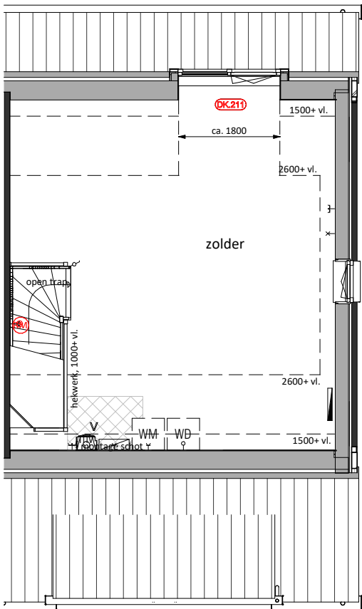
Tweede Verdieping DK.211 = Dakkapel ca.1800mm
