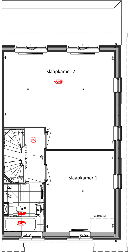
Eerste Verdieping A.106 = Slaapkamers achterzijde samenvoegen S.007 = Bad in badkamer (alleen met optie S.009) (draaistand raam vastzetten)
