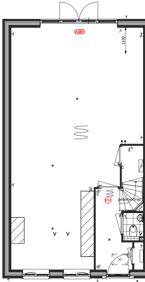
Begane Grond A.001 = Uitbouw achtergevel 1,2m
