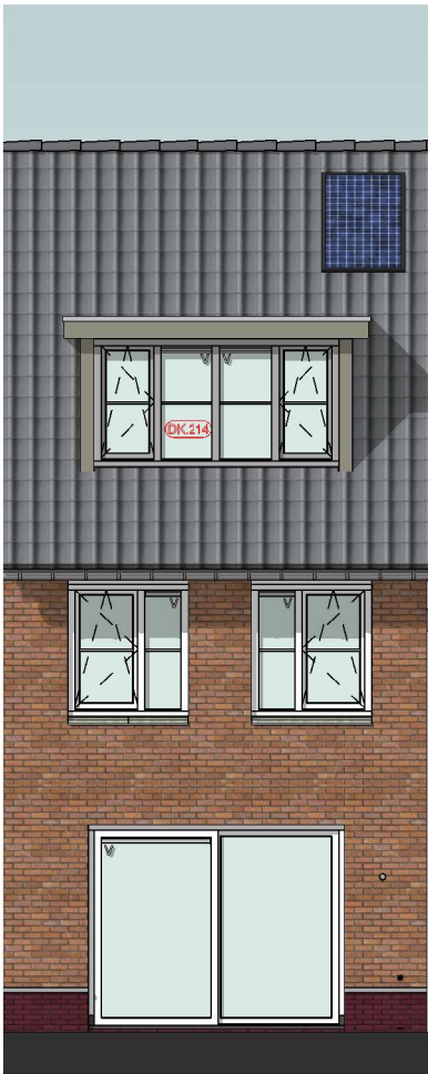
Achtergevel DK.241= Dakkapel ca.2900mm
