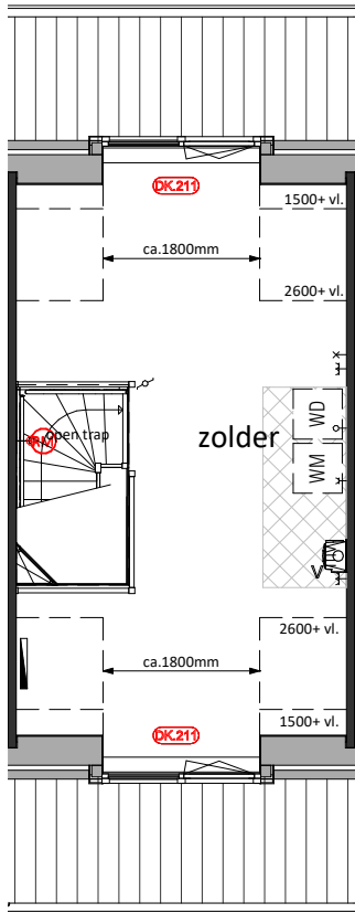
Tweede Verdieping DK.211 = Dakkapel ca.1800mm
