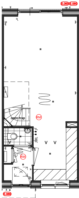
Begane Grond E.063 = Dubbele wcd op achtergevel E.060 = Extra buitenlichtpunt
