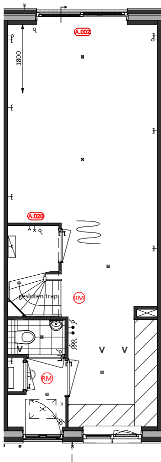
Begane Grond A.002 = Uitbouw achtergevel 1,8m A.020 = Trapkast
