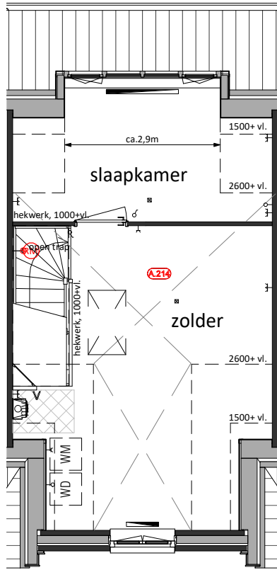
Tweede Verdieping A.214 = Upgrade van onbenoemde ruimte naar slaapkamer
