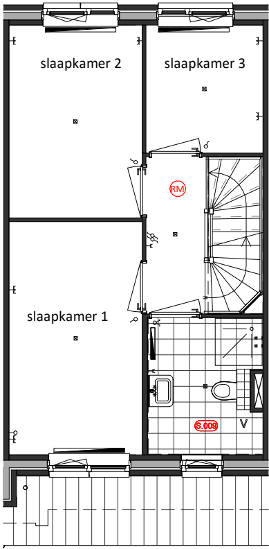
Eerste Verdieping S.009 = Verplaatsing toilet voorzijde schacht
