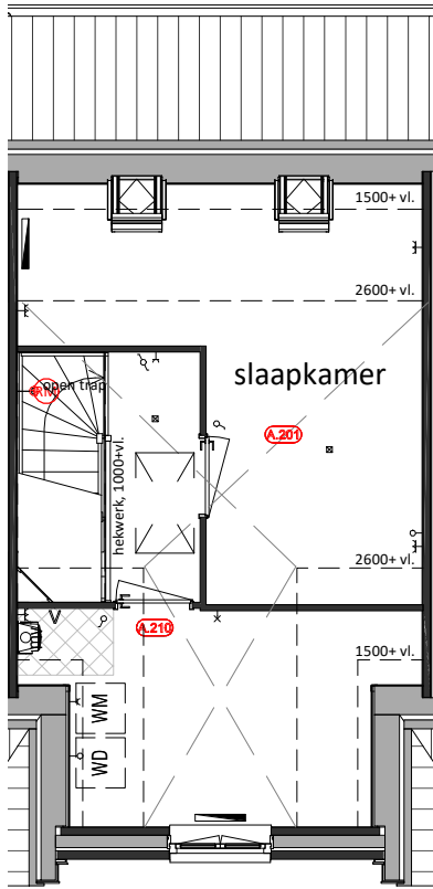
Tweede Verdieping A.201 = Zolderindeling met overloop en slaapkamer A.210 = Afgesloten technische ruimte
