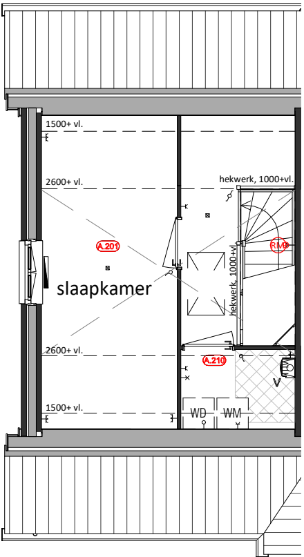
Tweede Verdieping A.201 = Zolderindeling met overloop en slaapkamer A.210 = Afgesloten technische ruimte
