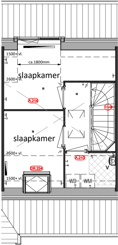
Tweede Verdieping A.214 = Upgrade van onbenoemde ruimte naar slaapkamer A.210 = Afgesloten technische ruimte DR.224 = Dakraam vergroten
