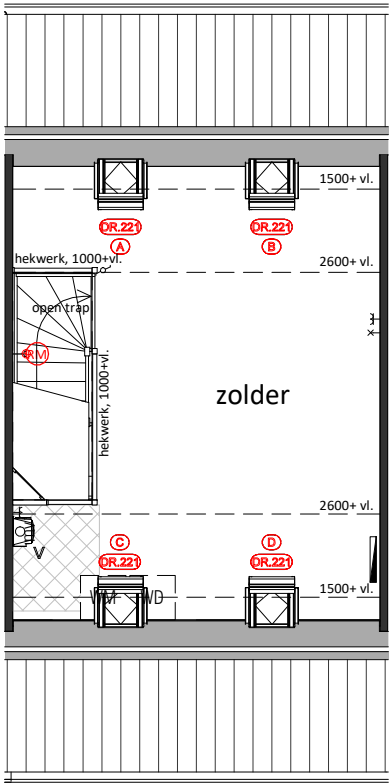
Tweede Verdieping DR.221 = Dakraam
