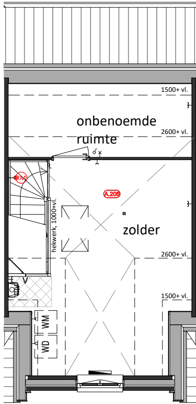
Tweede Verdieping A.206 = Zolderindeling met overloop en onbenoemde ruimte
