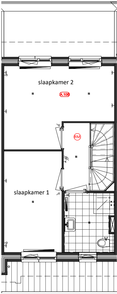
Eerste Verdieping A.106 = Slaapkamers achterzijde samenvoegen
