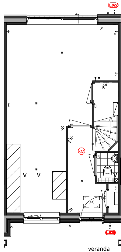
Begane Grond L.820 = Buitenkraan voorgevel L.822 = Buitenkraan achtergevel
