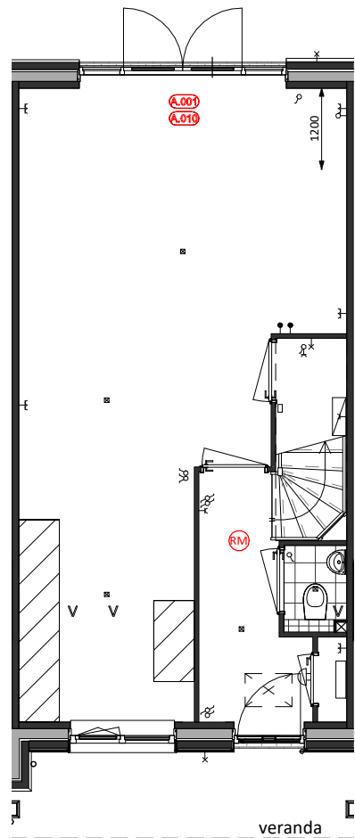
Begane Grond A.001 = Uitbouw achtergevel 1,2m A.010 = Openslaande deuren met zijlichten
