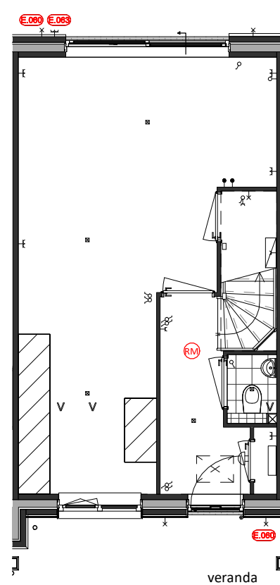
Begane Grond E.063 = Dubbele wcd op achtergevel E.060 = Extra buitenlichtpunt
