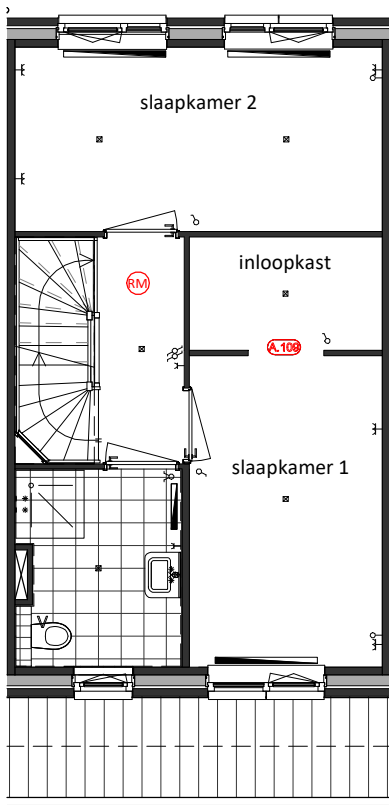
Eerste Verdieping A.109 = masterbedroom met inloopkast voorzijde woning
