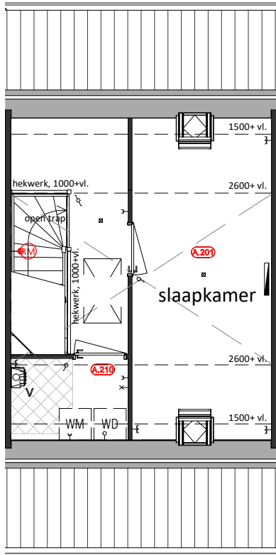
Tweede Verdieping A.201 = Zolderindeling met overloop en slaapkamer A.206 = Afgesloten technische ruimte
