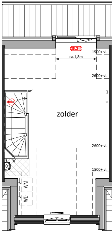
Tweede Verdieping DK.211 = Dakkapel ca.1,8m
