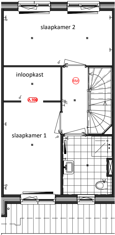
Eerste Verdieping A.109 = masterbedroom met inloopkast voorzijde woning
