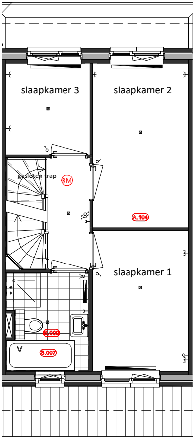
Eerste Verdieping A.104 = Scheidingswand verplaatsen 600mm S.007 = Bad in badkamer (alleen met optie S.009) (draaistand raam vastzetten)
