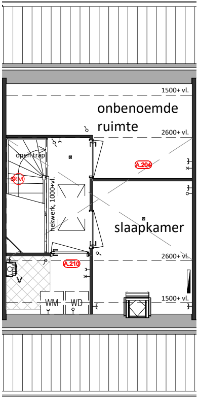
Tweede Verdieping A.204 = Zolderindeling met overloop, slaapkamer en onbenoemde ruimte A.210 = Afgesloten technische ruimte
