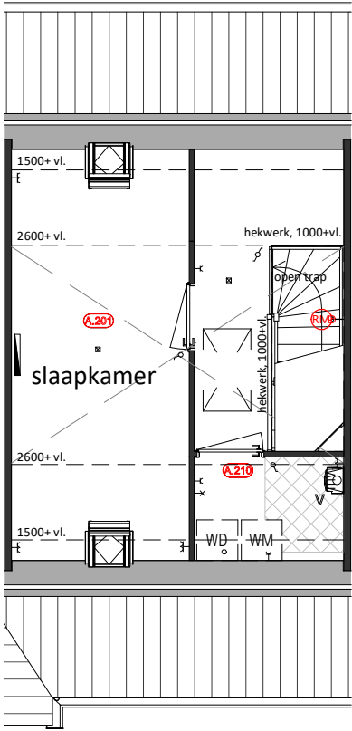
Tweede Verdieping A.201 = Zolderindeling met overloop en slaapkamer A.210 = Afgesloten technische ruimte
