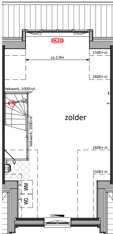
Tweede Verdieping DK.212 = Dakkapel ca.2,9m
