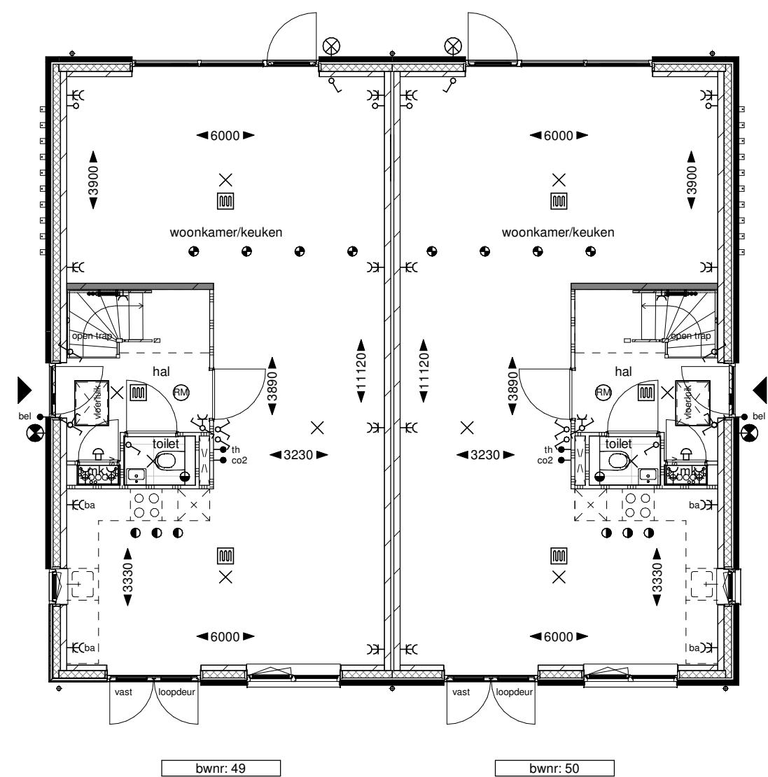
Begane grond
