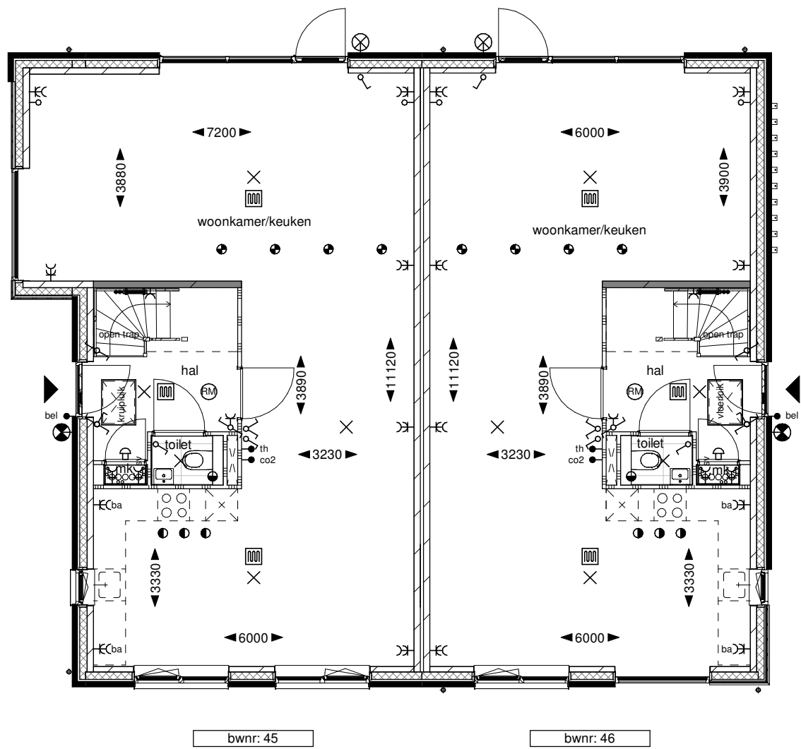
Begane grond
