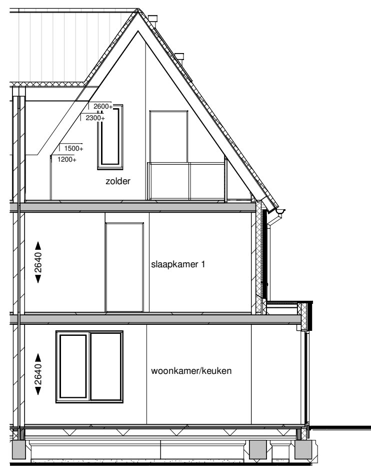
Doorsnede B
