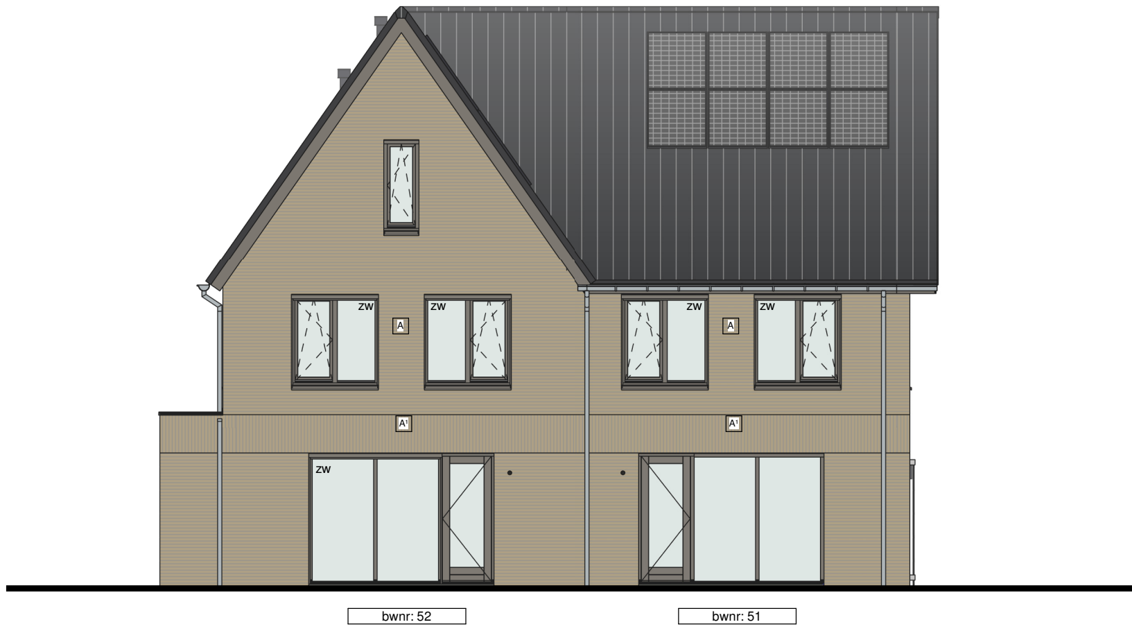
Achtergevel
