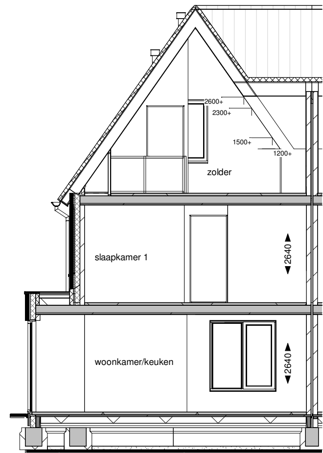
Doorsnede B
