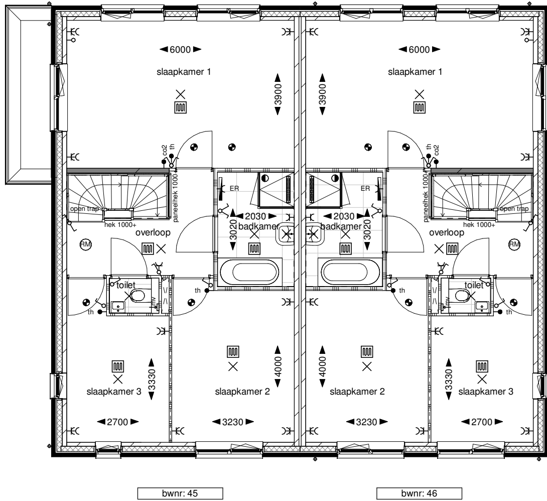
Eerste verdieping
