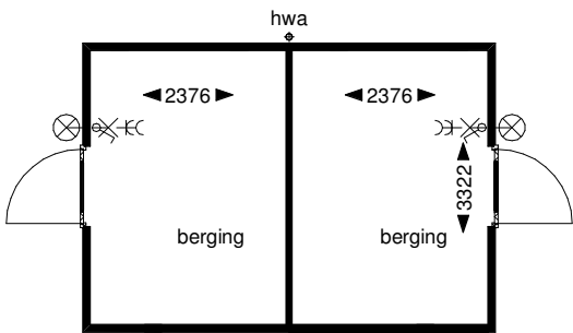
Begane grond
