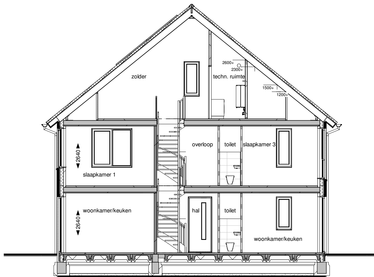
Doorsnede A
