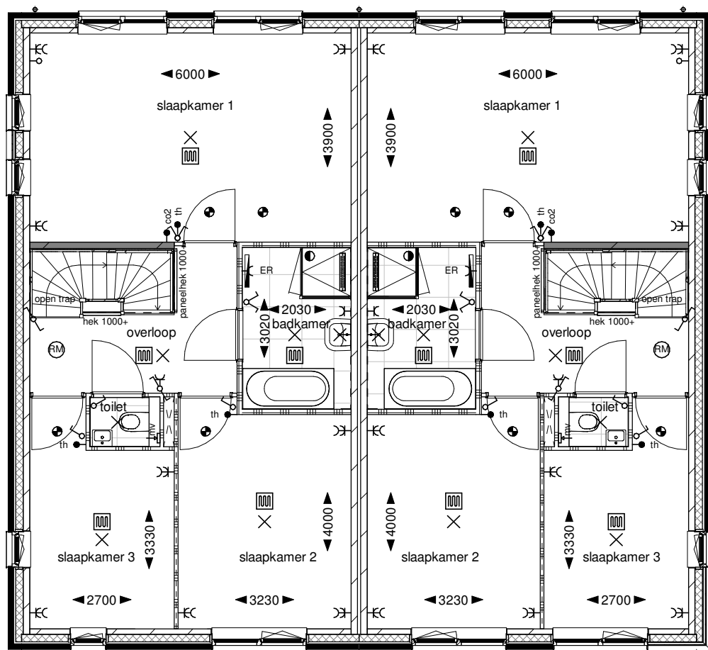
Eerste verdieping
