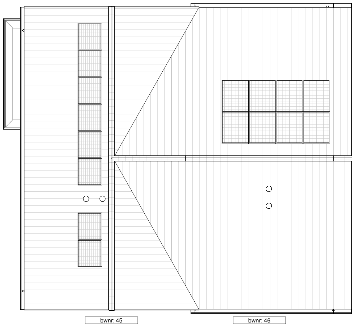
Dakaanzicht
