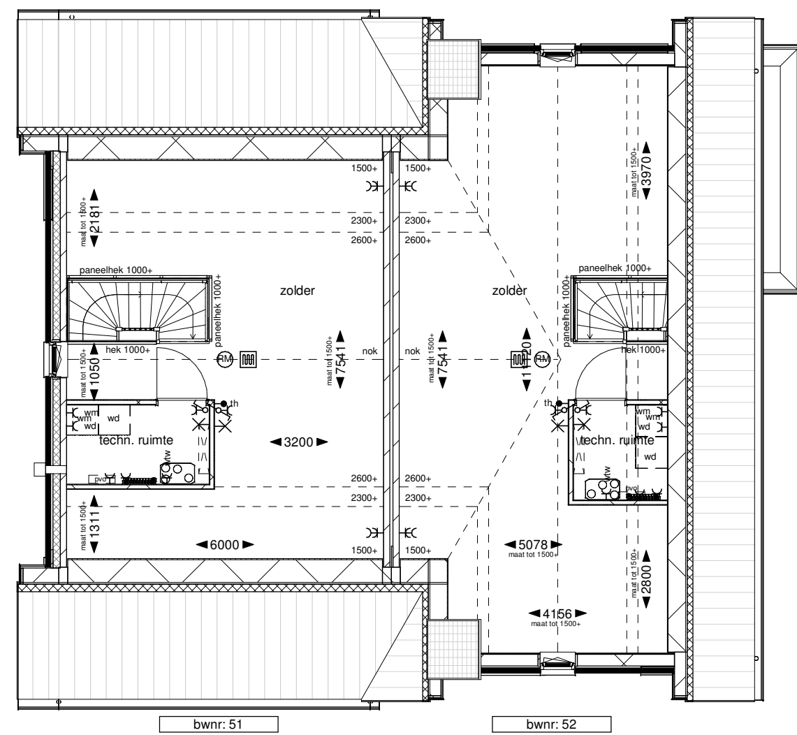
Tweede verdieping
