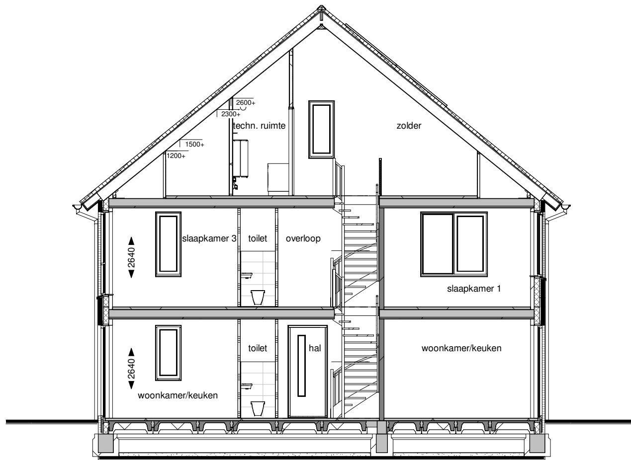
Doorsnede A
