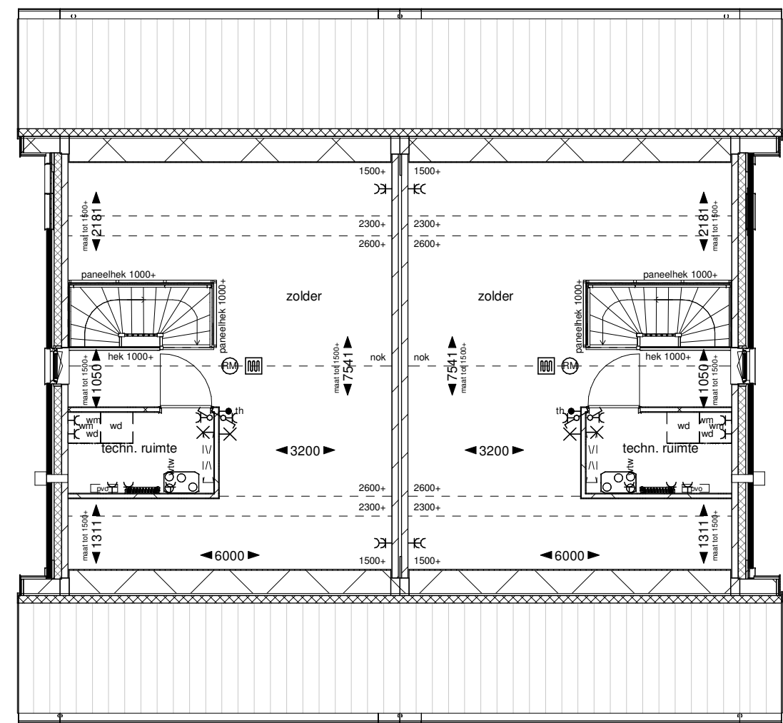
Tweede verdieping
