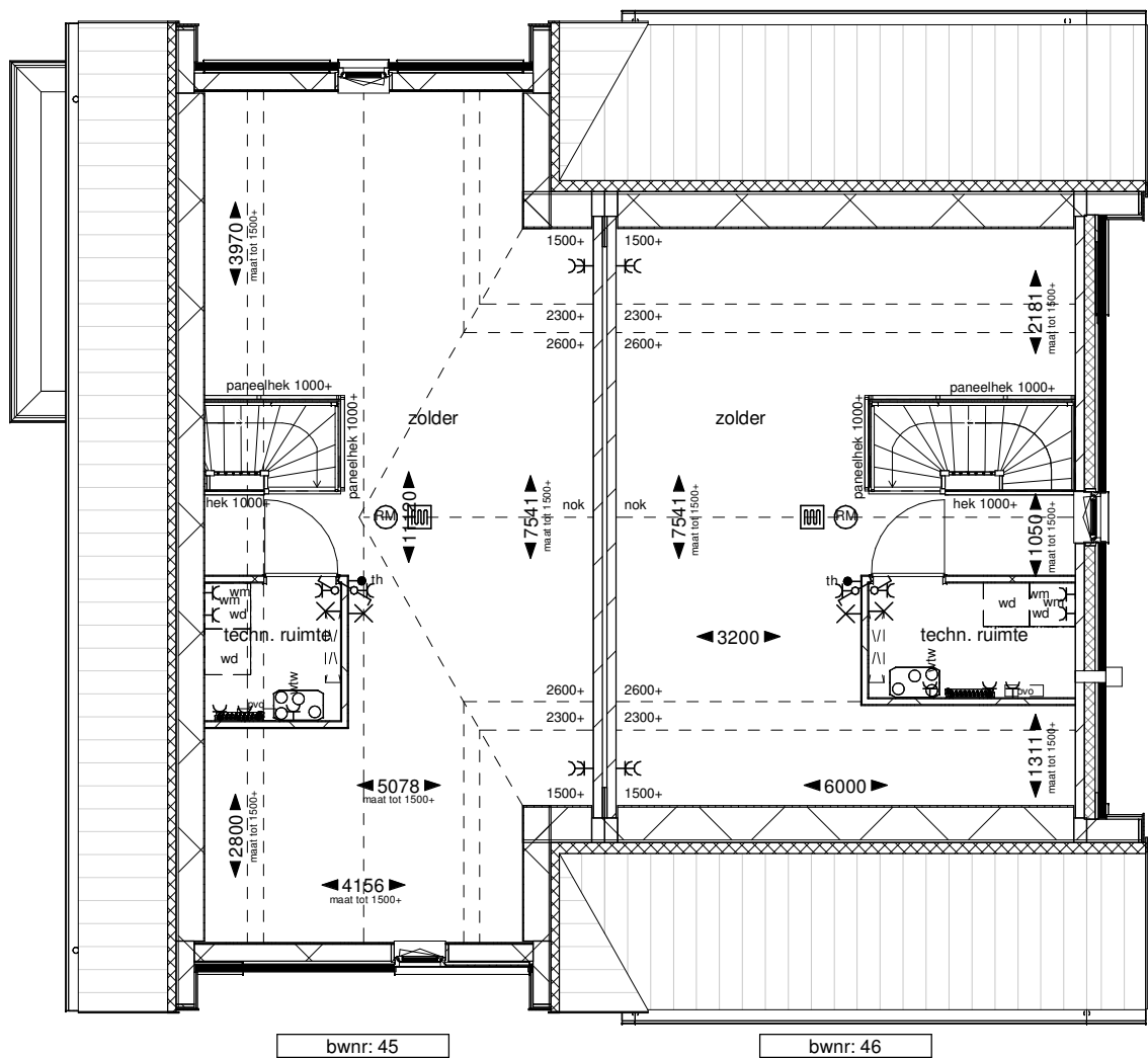
Tweede verdieping
