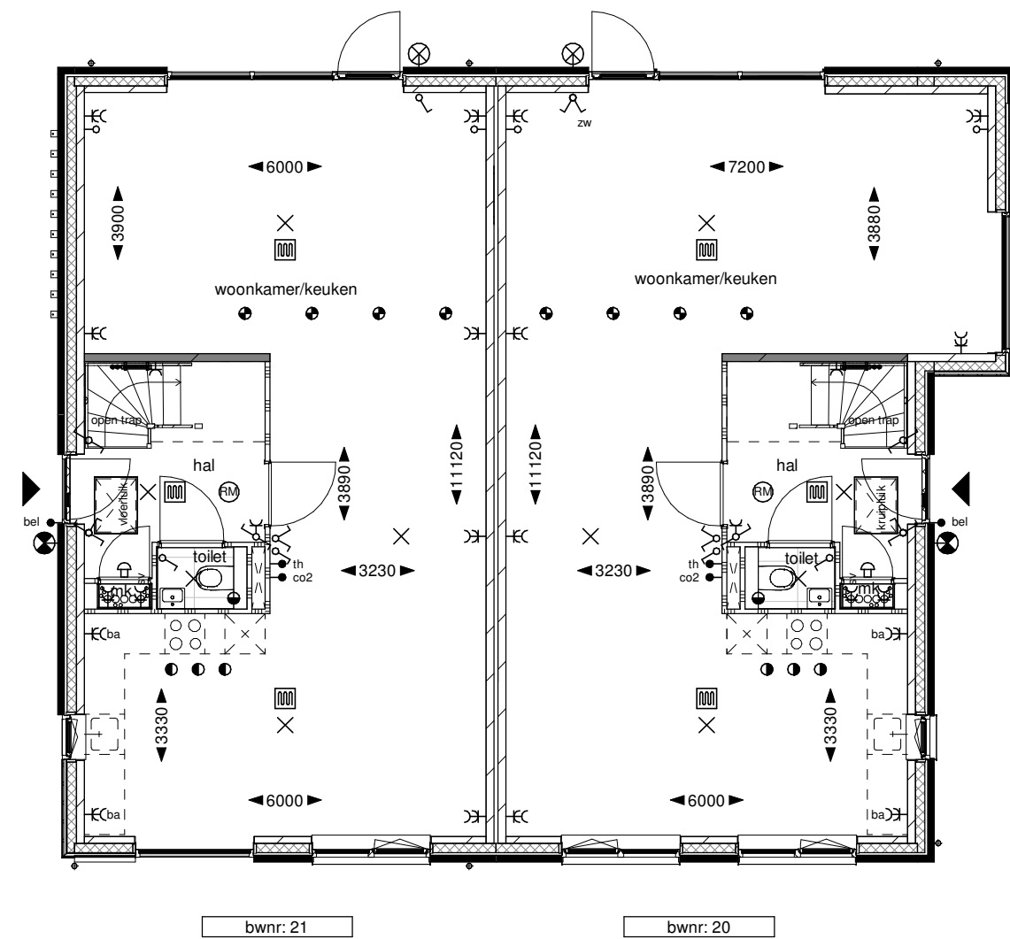
Begane grond
