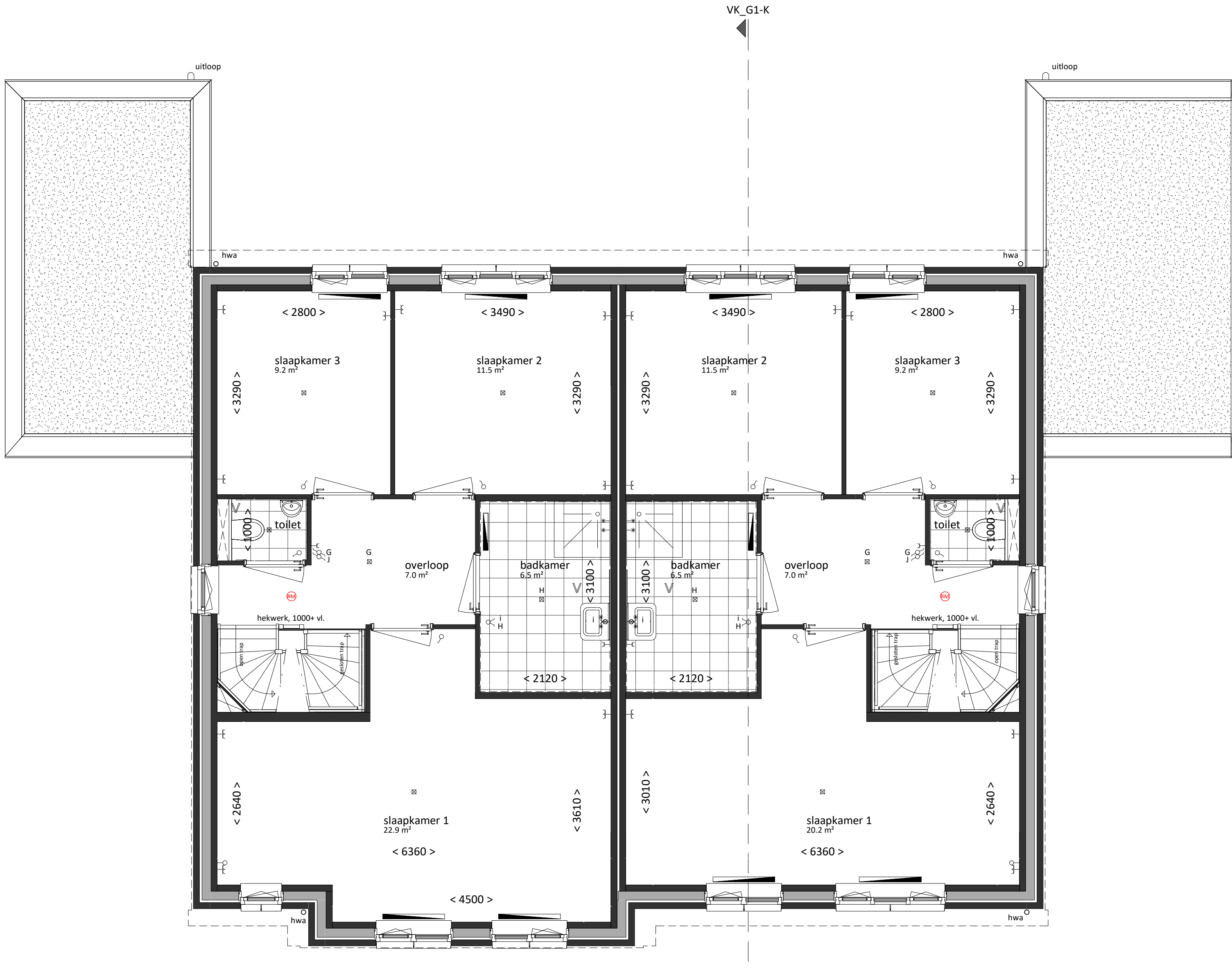
eerste verdieping bk. vloer = 2900+ schaal 1:50
