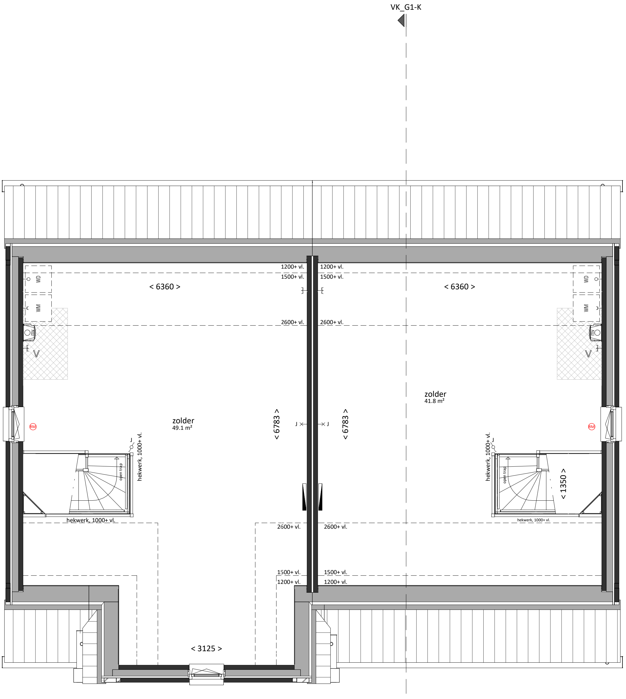
tweede verdieping bk. vloer = 5800+ schaal 1:50
