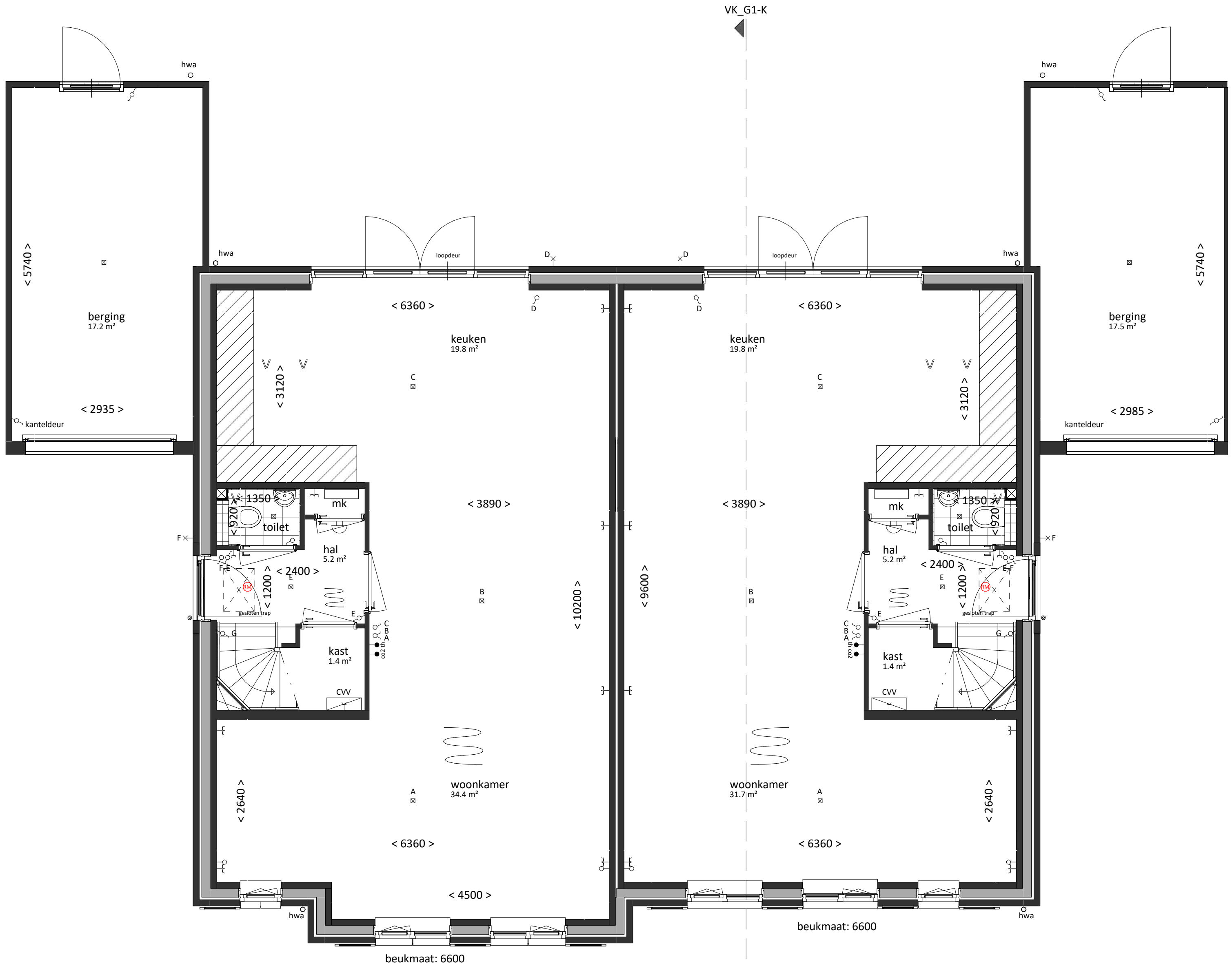
begane grond bk. vloer = P = 0 schaal 1:50
