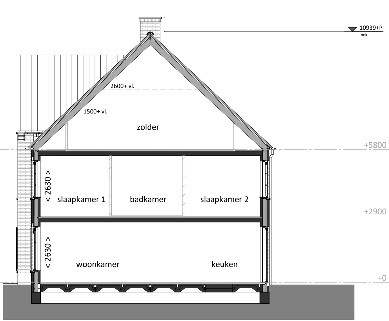
doorsnede schaal 1:100
