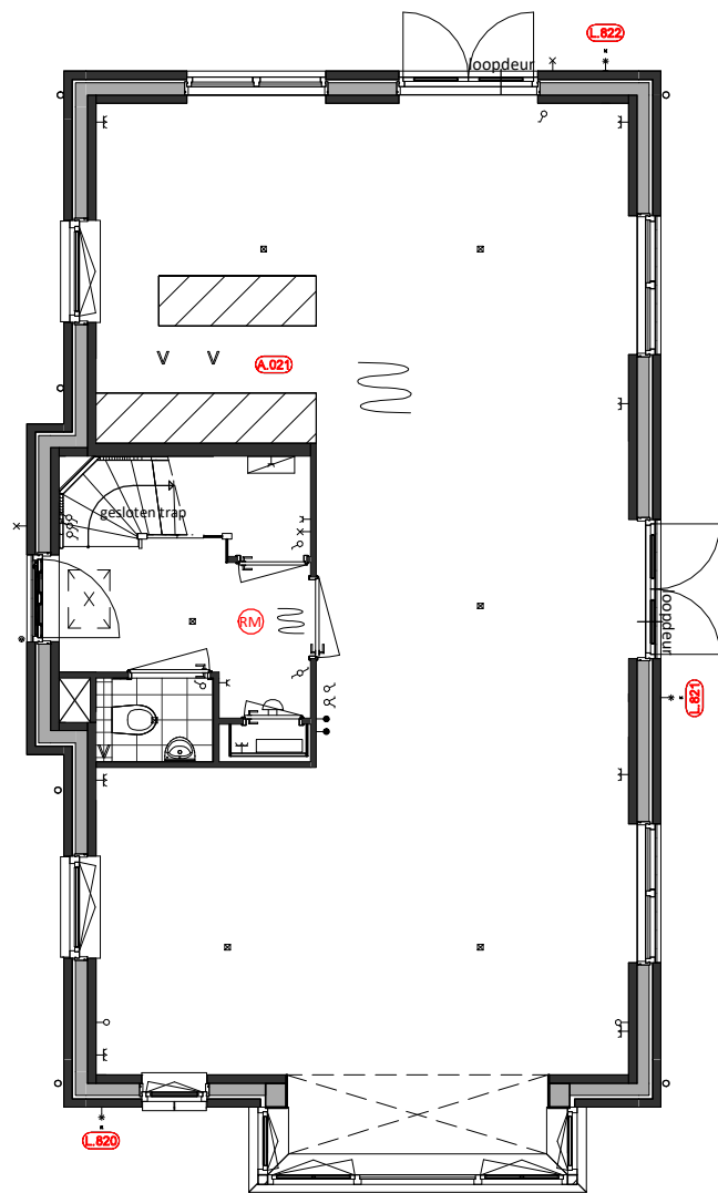
Begane grond A.021 = Keuken naar achterzijde woning L.820 = Buitenkraan voorgevel L.821 = Buitenkraan zijgevel L.822 = Buitenkraan achtergevel
