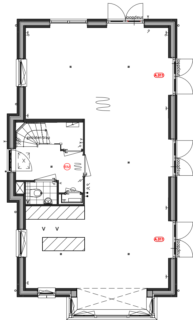
Begane grond A.011 = Zijgevel voorzien van openslaande deuren ipv vast venster
