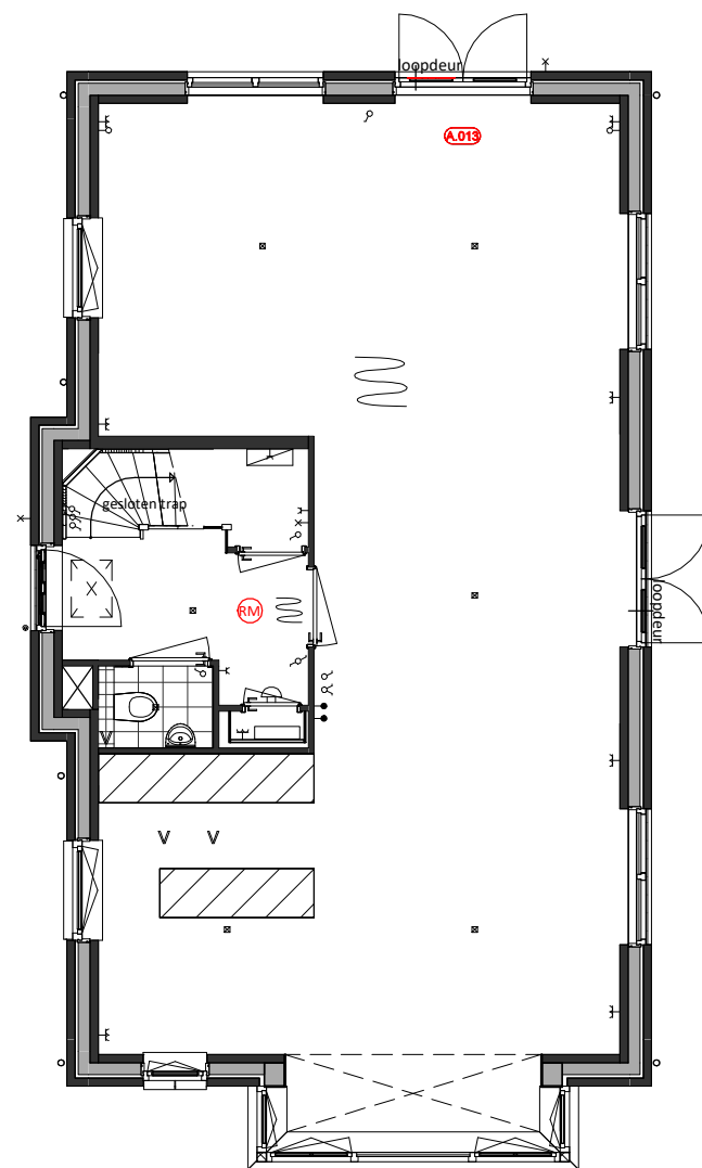
Begane grond A.013 = Wijzigen schuifpui of loopdeur openslaande deuren
