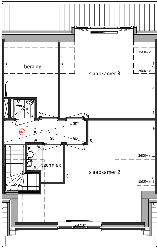
Eerste verdieping Basis
