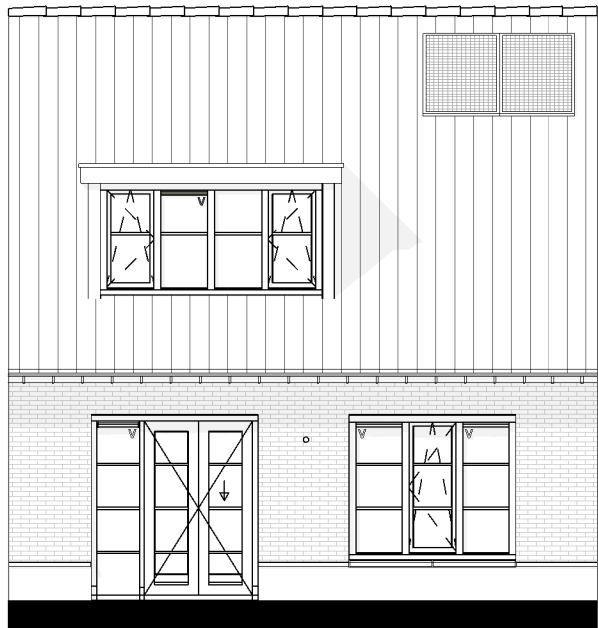
Achtergevel Basis
