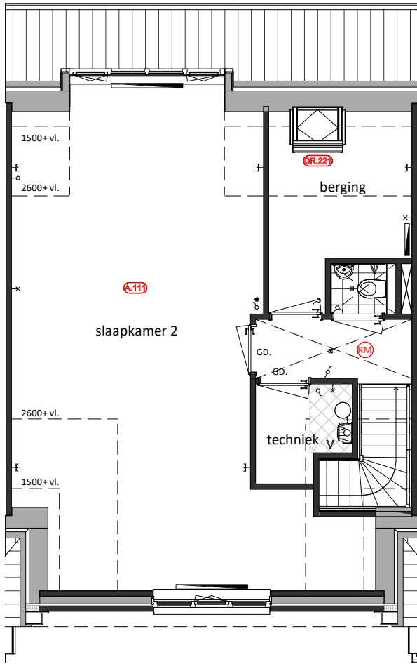
Eerste verdieping A.111 = Slaapkamer 2 en 3 samenvoegen DR.221 = Extra houten tuimeldakraam
