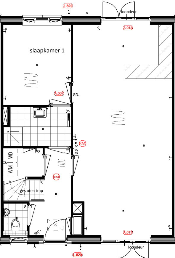
Begane Grond A.013 = Wijzigen loopdeur openslaande deuren A.057 = Slaapkamer 1 verkleinen L.820 = Vorstvrije buitenkraan (gevelplaat) op de voorgevel L.822 = Vorstvrije buitenkraan (gevelplaat) op de achtergevel
