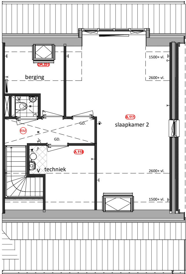
Eerste verdieping A.111 = Slaapkamer 2 en 3 samenvoegen DR.221 = Extra houten tuimeldakraam A.113 = Vergroten techniekruimte
