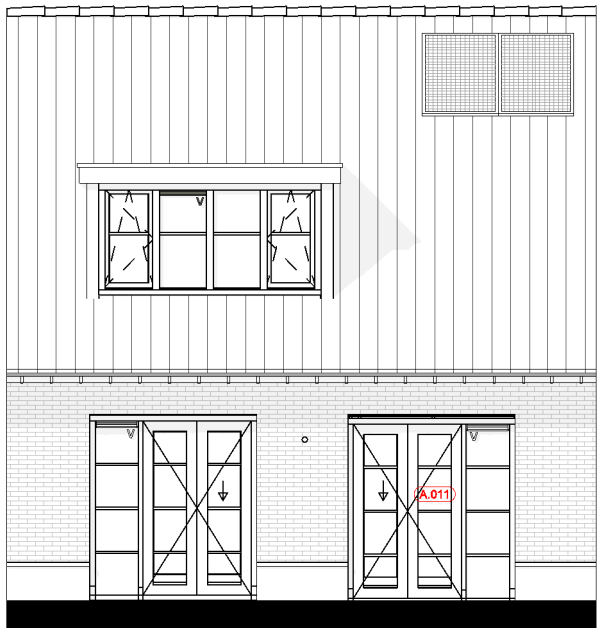
Achtergevel A.011 = Achtergevel voorzien van extra dubbele deuren
