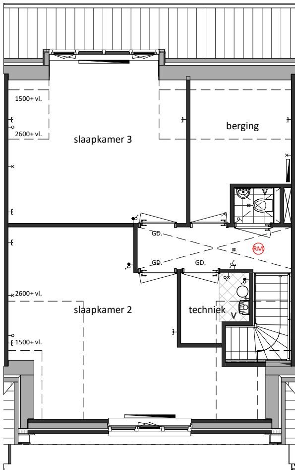
Eerste verdieping Basis
