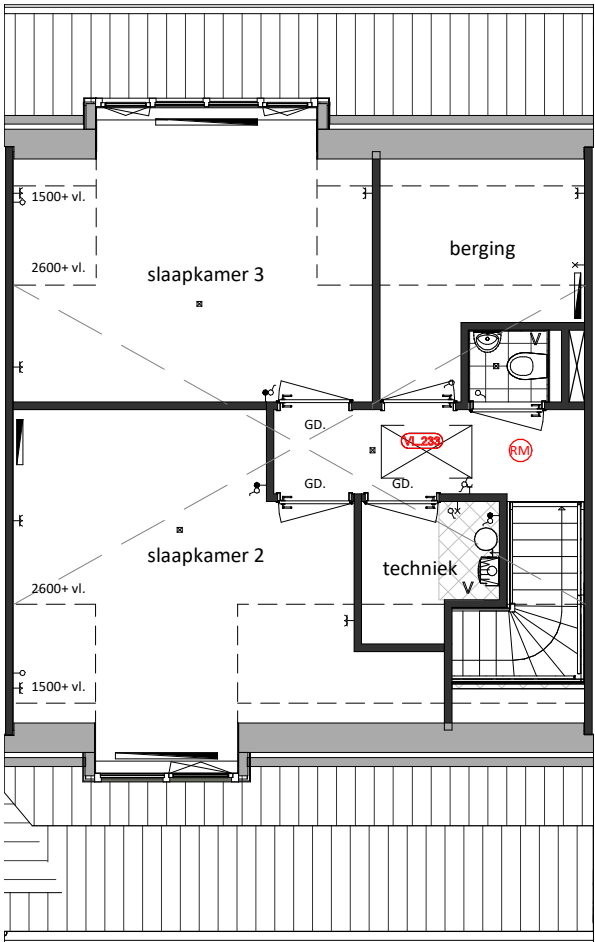
Eerste verdieping VL.233 = Vliering afgewerkt type H5-L
