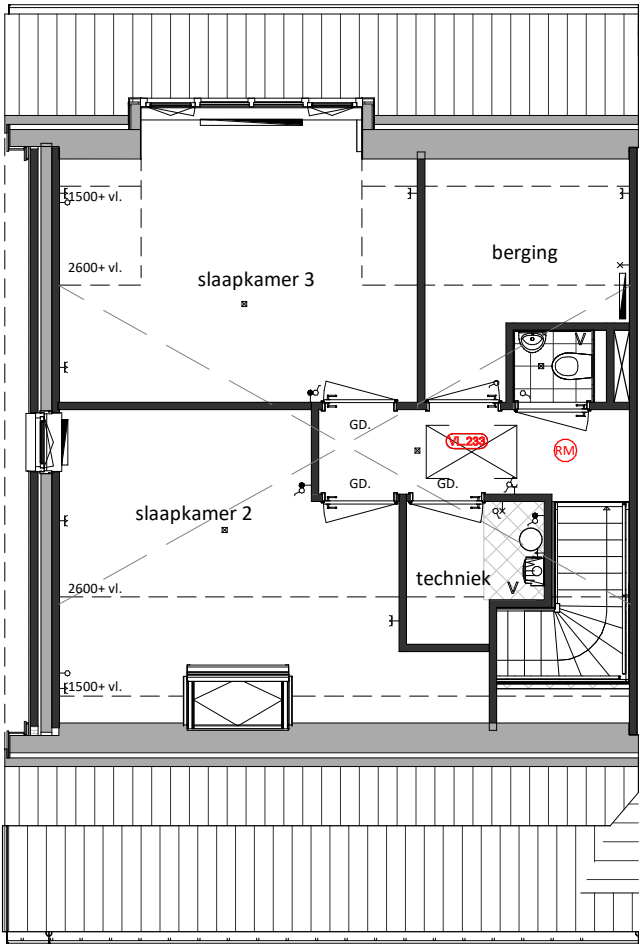
Eerste verdieping VL.233 = Vliering afgewerkt type H5-L
