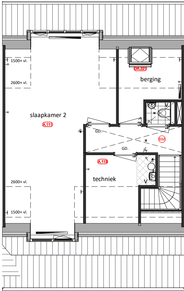
Eerste verdieping A.111 = Slaapkamer 2 en 3 samenvoegen DR.221 = Extra houten tuimeldakraam A.113 = Vergroten techniekruimte
