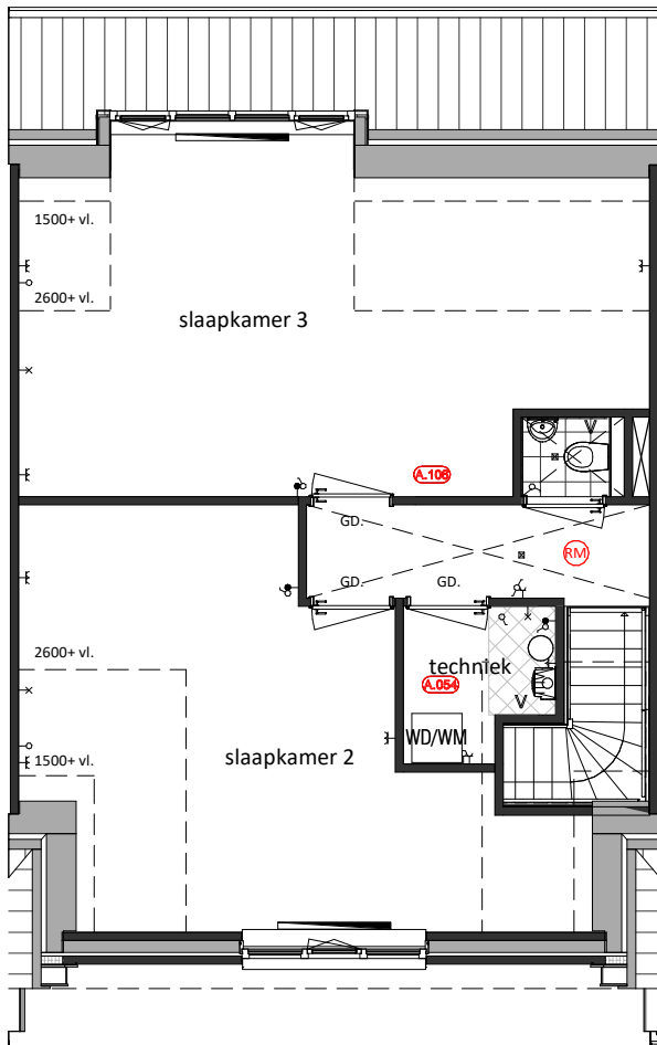
Eerste verdieping A.106 = Slaapkamer en berging achterzijde samenvoegen A.054 = verplaatsen wasmachine-opstelling naar eerste verdieping
