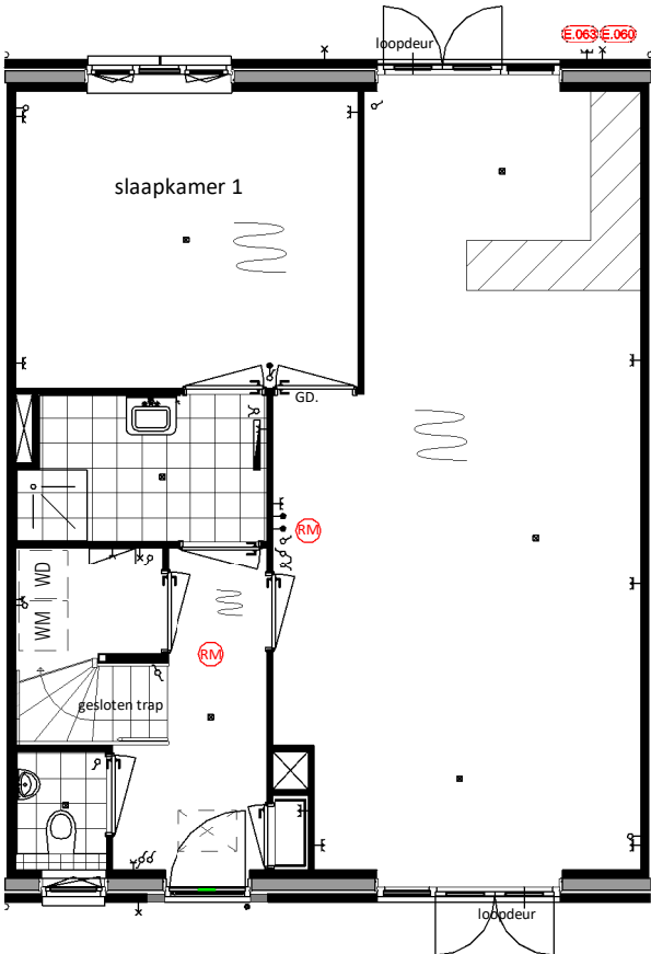
Begane Grond E.060 = Extra buitenlichtpunt E.063 = Dubbele WCD op achtergevel
