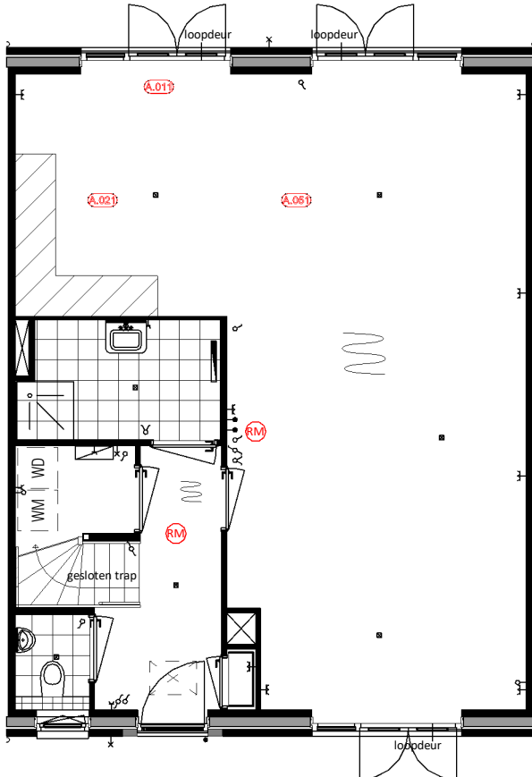
Begane Grond A.011 = Achtergevel voorzien van extra dubbele deuren A.021 = De keuken wordt naar de achterzijde van de woning verplaatst (trapzijde) A.051 = Woonkamer vergroten, slaapkamer 1 vervalt
