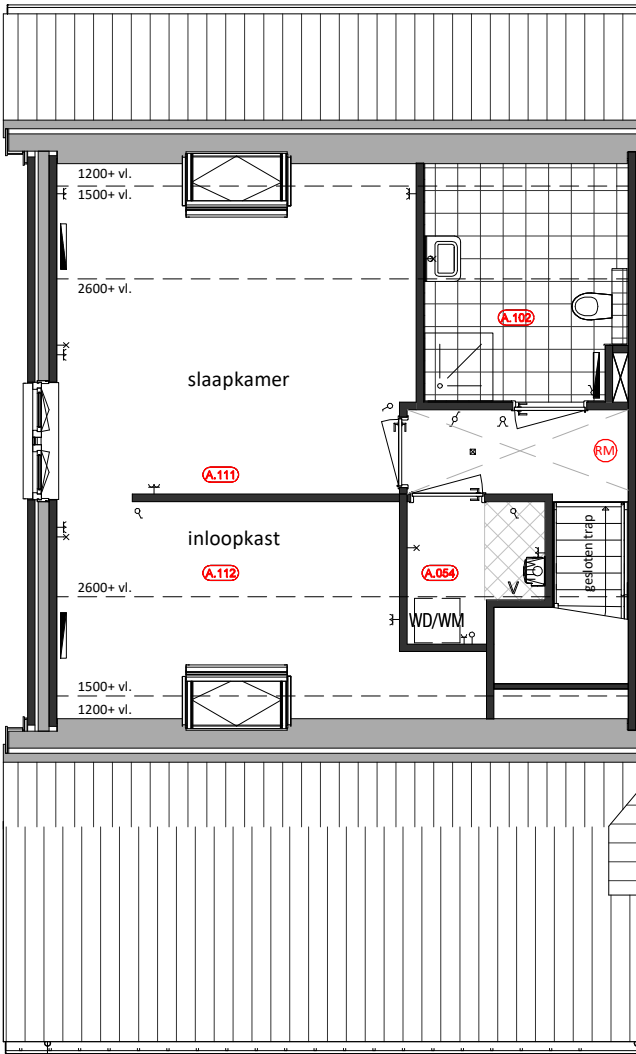
Eerste Verdieping A.102 = Badkamer op 1e verdieping A.111 = Samenvoegen slaapkamer 2 en 3 A.112 = Inloopkast in samengevoegde slaapkamer A.054 = Verplaatsing wasmachine opstelling
