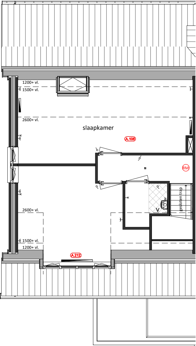
Eerste Verdieping A.106 = Slaapkamer en berging samenvoegen A.212 = Dakvenster vangen door dakkapel
