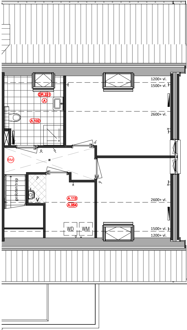
Eerste Verdieping A.102 = Badkamer op 1e verdieping A.113 = Vergroten techniek DR.221 = Dakraam
