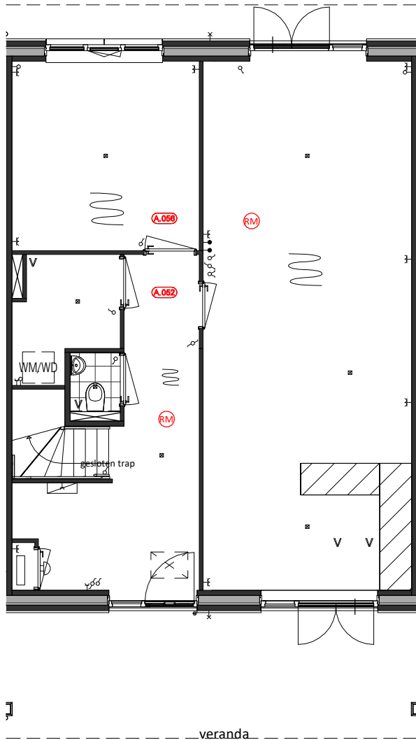
Begane Grond A.052 = Kleine berging ipv. badkamer A.056 = Deur woonkamer naar slaapkamer vervalt
