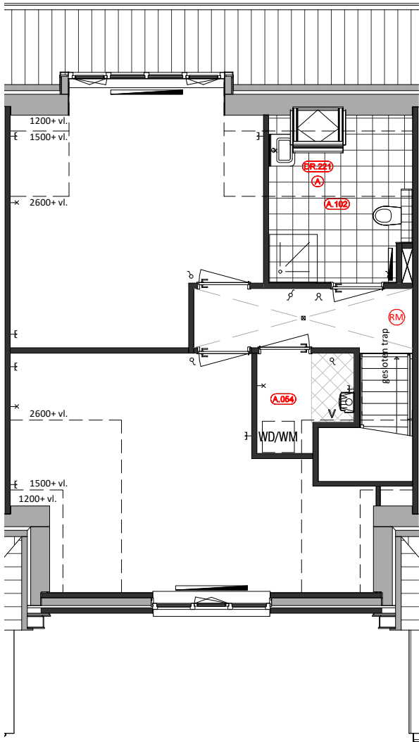
Eerste Verdieping A.102 = Badkamer op 1e verdieping A.054 = Verplaatsing wasmachine opstelling DR.221 = Dakraam
