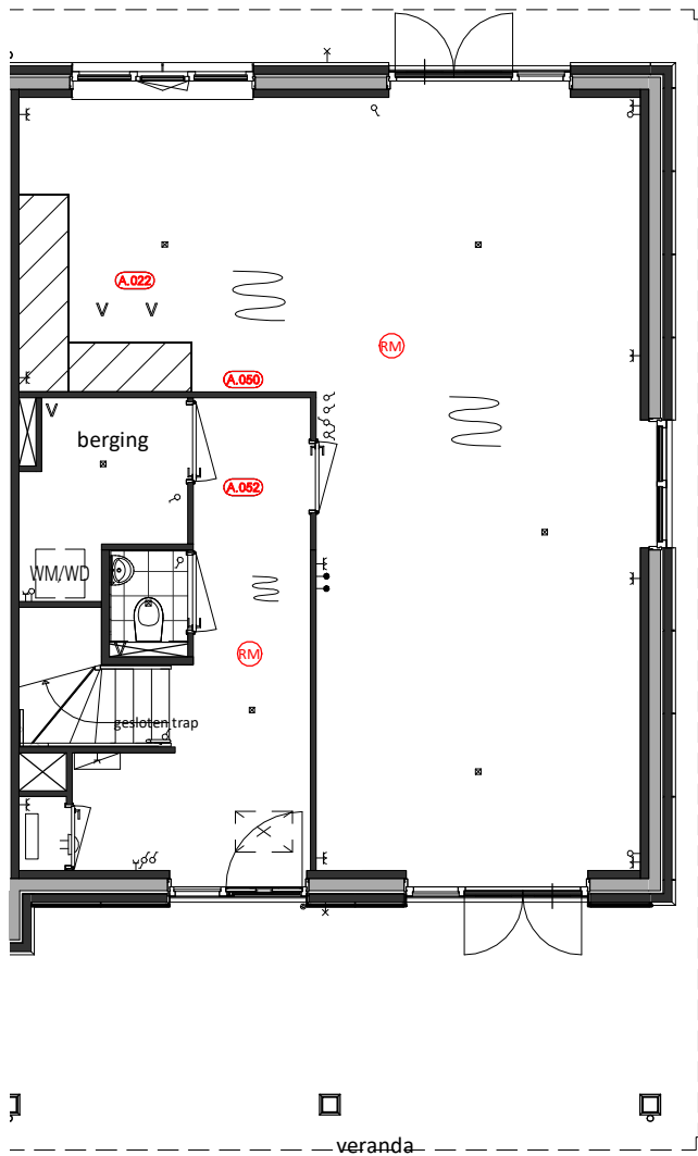
Begane Grond A.022 = Keuken naar achterkant (trapzijde) A.050 = Deur naar badkamer vervalt A.052 = Kleine berging ipv. badkamer
