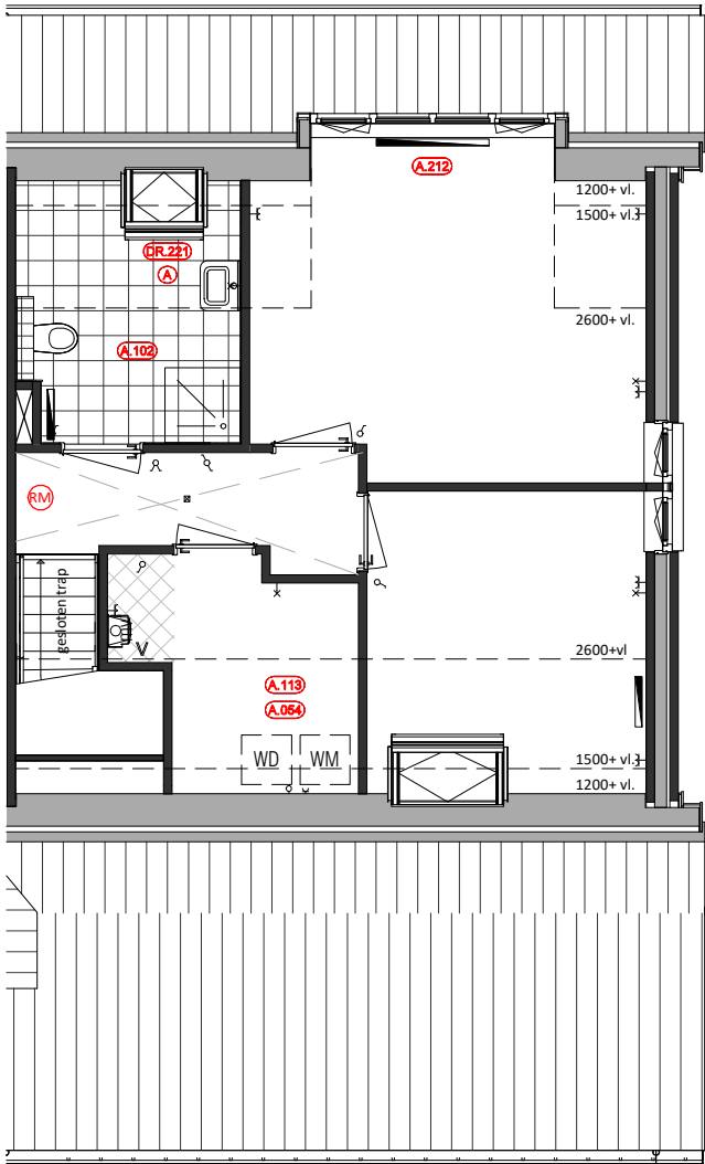
Eerste Verdieping A.102 = Badkamer op 1e verdieping A.113 = Vergroten techniek A.054 = Verplaatsing wasmachine opstelling DR.221 = Dakraam A.212 = Dakraam vervangen door dakkapel
