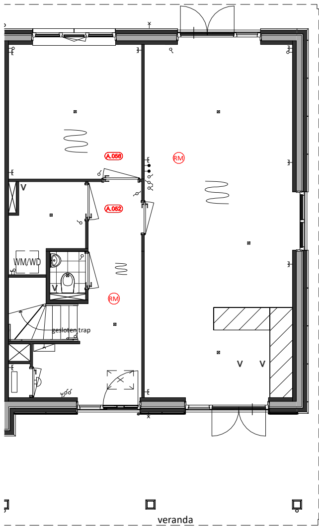
Begane Grond A.052 = Kleine berging ipv. badkamer A.056 = Deur woonkamer naar slaapkamer vervalt
