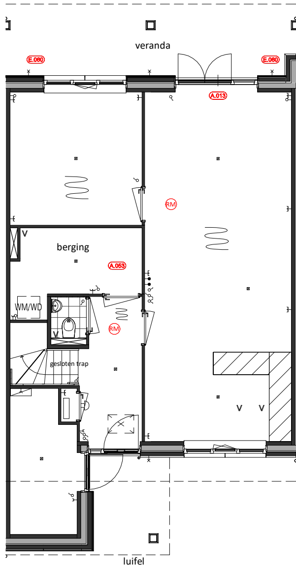
Begane Grond A.013 = Wijziging loopdeur A.053 = Berging ipv. badkamer E.000 = Extra buitenlichtpunt
