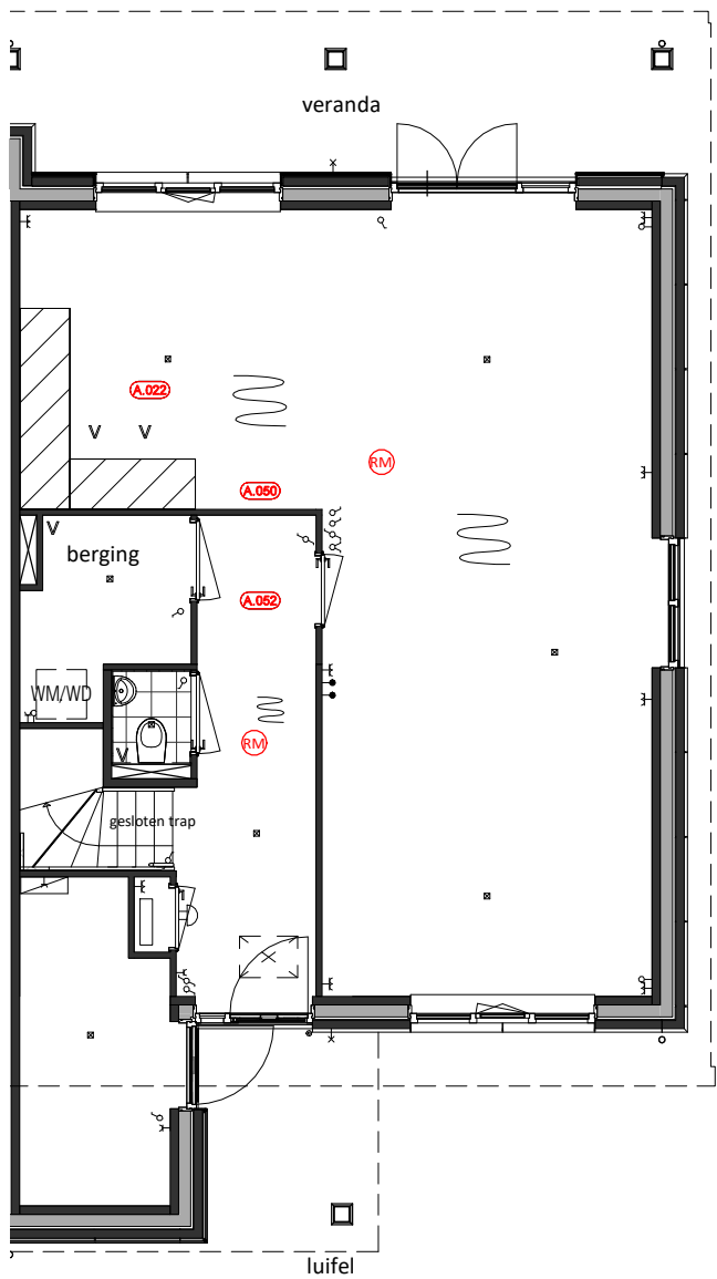
Begane Grond A.022 = Keuken naar achterkant (trapzijde) A.050 = Deur naar badkamer vervalt A.052 = Kleine berging ipv. badkamer
