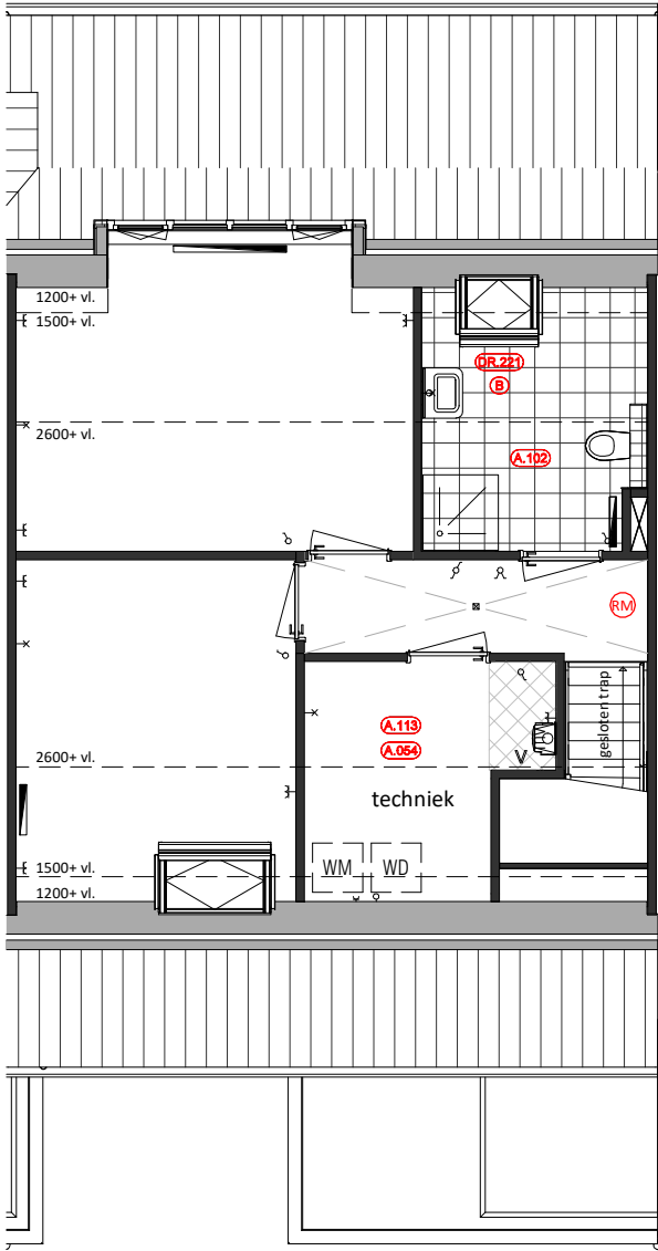
Eerste Verdieping A.102 = Badkamer op 1e verdieping A.113 = Vergroten techniek A.054 = Dakraam
