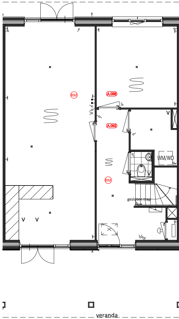
Begane Grond A.052 = Kleine berging ipv. badkamer A.056 = Deur woonkamer naar slaapkamer verval
