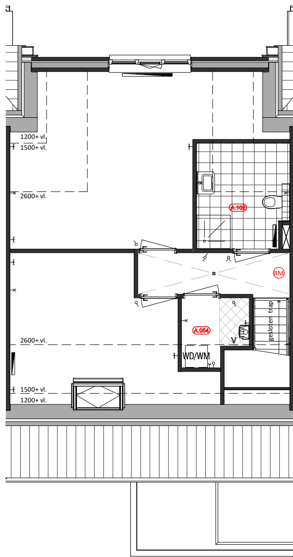
Eerste Verdieping A.102 = Badkamer op 1e verdieping A.054 = Verplaatsing wasmachine opstelling
