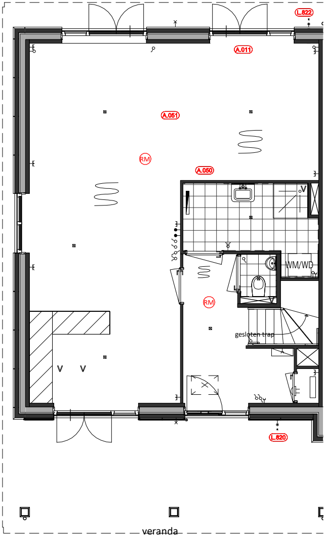
Begane Grond A.011 = Extra dubbele deuren A.050 = Deur naar badkamer vervalt A.051 = Woonkamer vergroten L.820 = Buitenkraan voorgevel L.822 = Buitenkraan achtergevel
