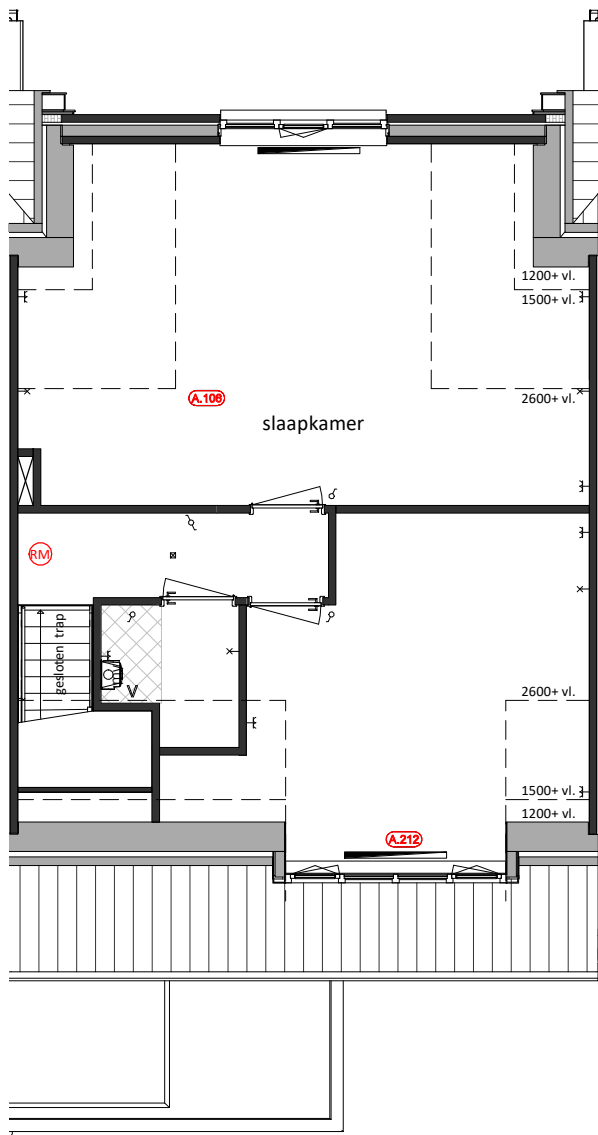
Eerste Verdieping A.106 = Slaapkamer en berging samenvoegen A.212 = Dakvenster vangen door dakkapel
