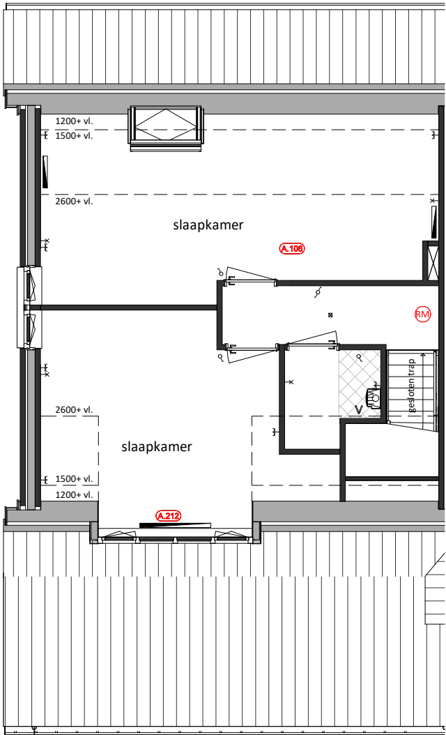
Eerste Verdieping A.106 = Slaapkamer en berging samenvoegen A.212 = Dakvenster vangen door dakkapel
