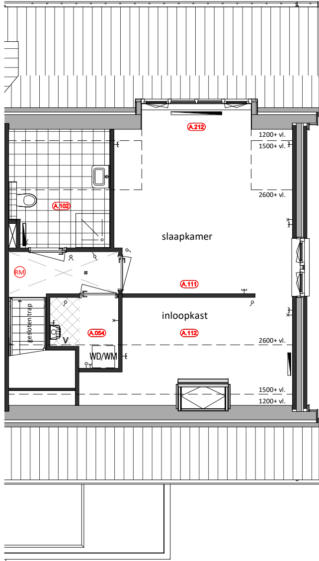
Eerste Verdieping A.102 = Badkamer op 1e verdieping A.111 = Samenvoegen slaapkamer 2 en 3 A.112 = Inloopkast in samengevoegde slaapkamer A.054 = Verplaatsing wasmachine opstelling A.212 = Dakraam vervangen door dakkapel
