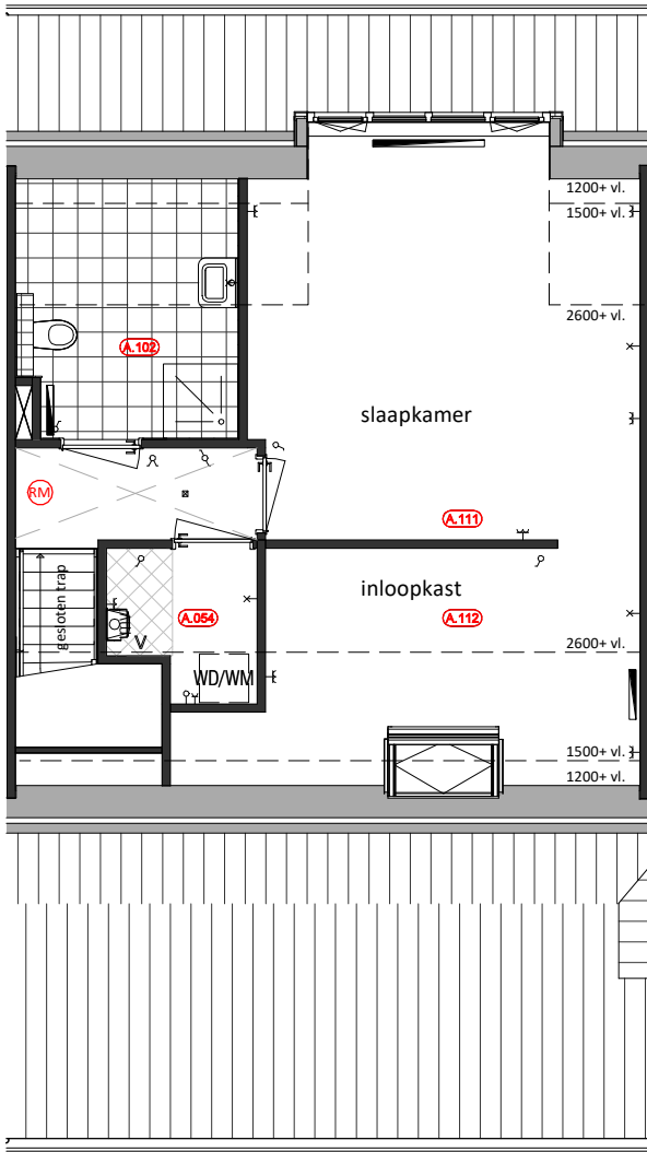
Eerste Verdieping A.102 = Badkamer op 1e verdieping A.111 = Samenvoegen slaapkamer 2 en 3 A.112 = Inloopkast in samengevoegde slaapkamer A.054 = Verplaatsing wasmachine opstelling
