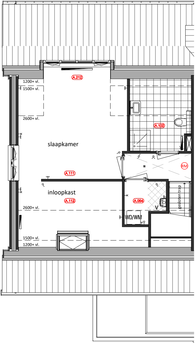
Begane Grond A.102 = Badkamer op 1e verdieping A.111 = Samenvoegen slaapkamer 2 en 3 A.112 = Inloopkast in samengevoegde slaapkamer A.054 = Verplaatsing wasmachine opstelling A.212 = Dakraam vervangen door dakkapel
