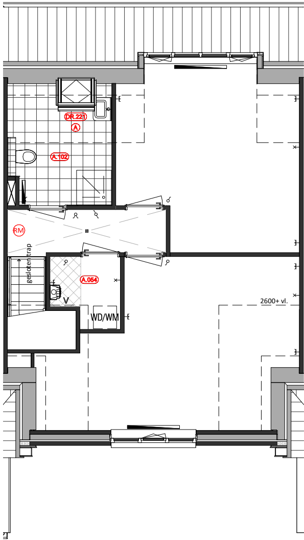
Eerste Verdieping A.102 = Badkamer op 1e verdieping A.212 = Dakvenster vangen door dakkapel A.054 = Verplaatsing wasmachine opstelling DR.221 = Dakraam
