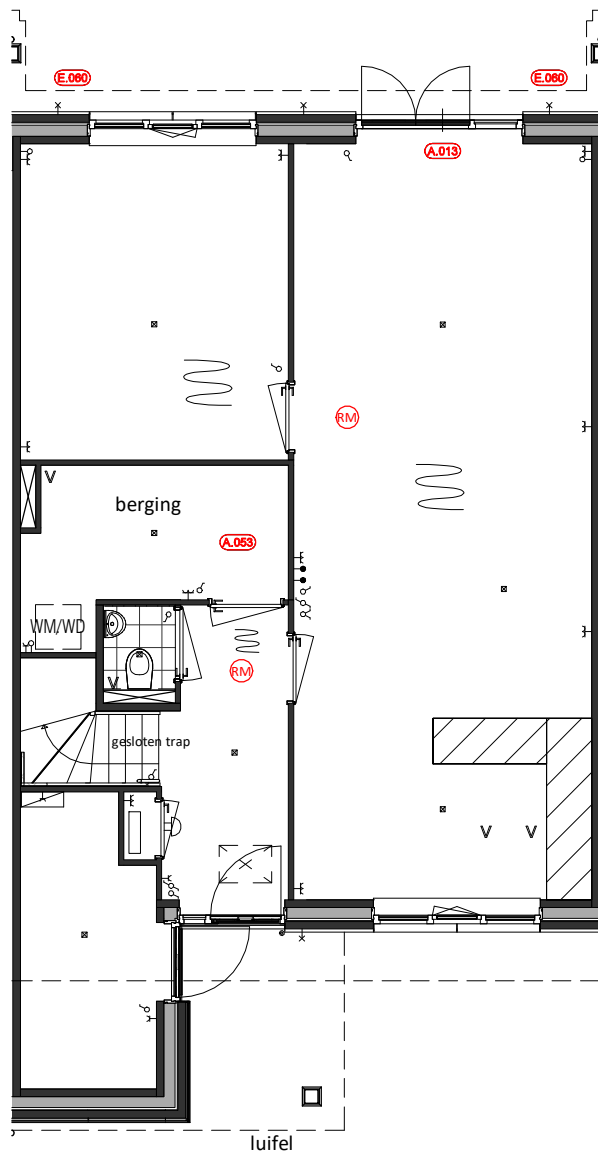
Begane Grond A.013 = Wijziging loopdeur A.053 = Berging ipv. badkamer E.060 = Extra buitenlichtpunt
