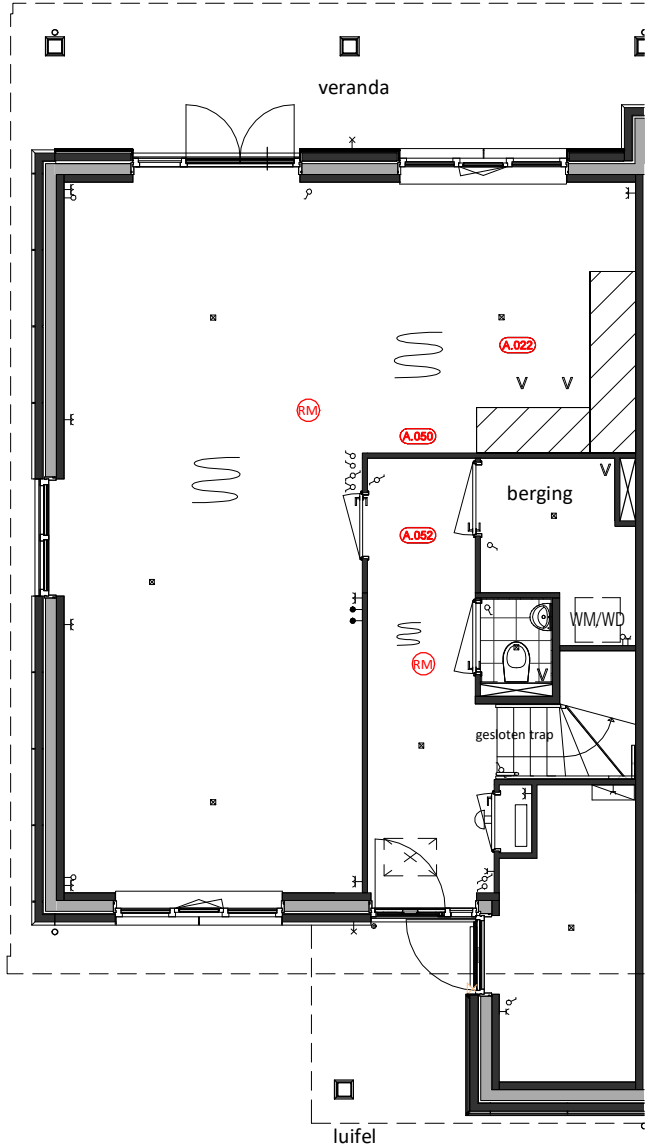
Begane Grond A.022 = Keuken naar achterkant (trapzijde) A.050 = Deur naar badkamer vervalt A.052 = Kleine berging ipv. badkamer
