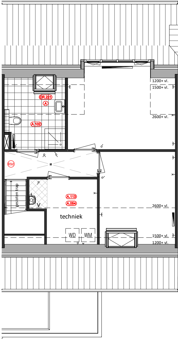
Eerste Verdieping A.102 = Badkamer op 1e verdieping A.113 = Vergroten techniek A.054 = Verplaatsing wasmachine opstelling DR.221 = Dakraam
