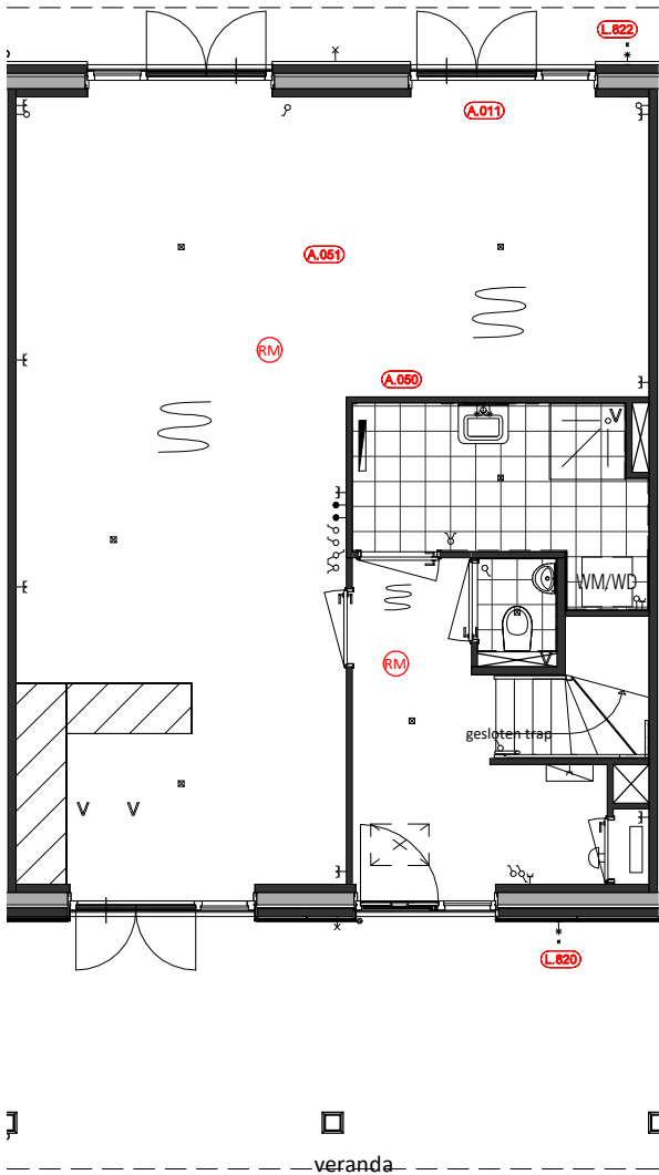
Begane Grond A.011 = Extra dubbele deuren A.050 = Deur naar badkamer vervalt A.051 = Woonkamer vergroten L.820 = Buitenkraan voorgevel L.822 = Buitenkraan achtergevel
