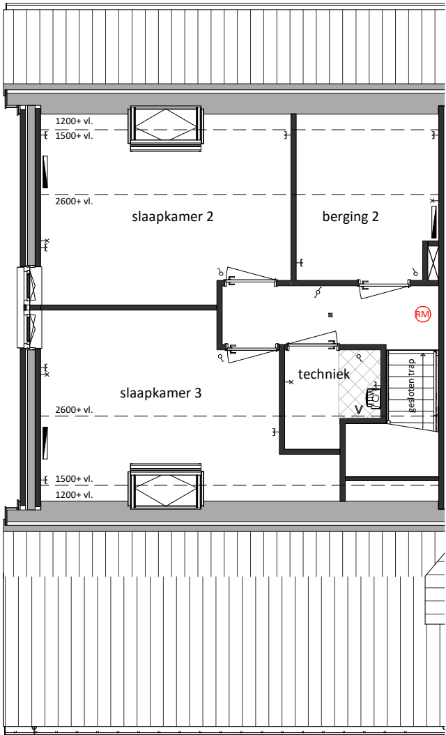
Eerste Verdieping Basis
