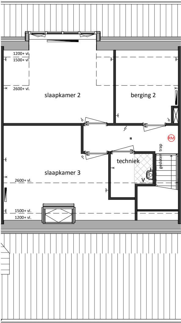
Eerste Verdieping Basis
