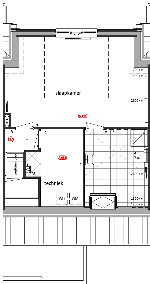
Eerste Verdieping A.114 = Masterbedroom met badkamer voorzijde A.054 = Verplaatsing wasmachine opstelling
