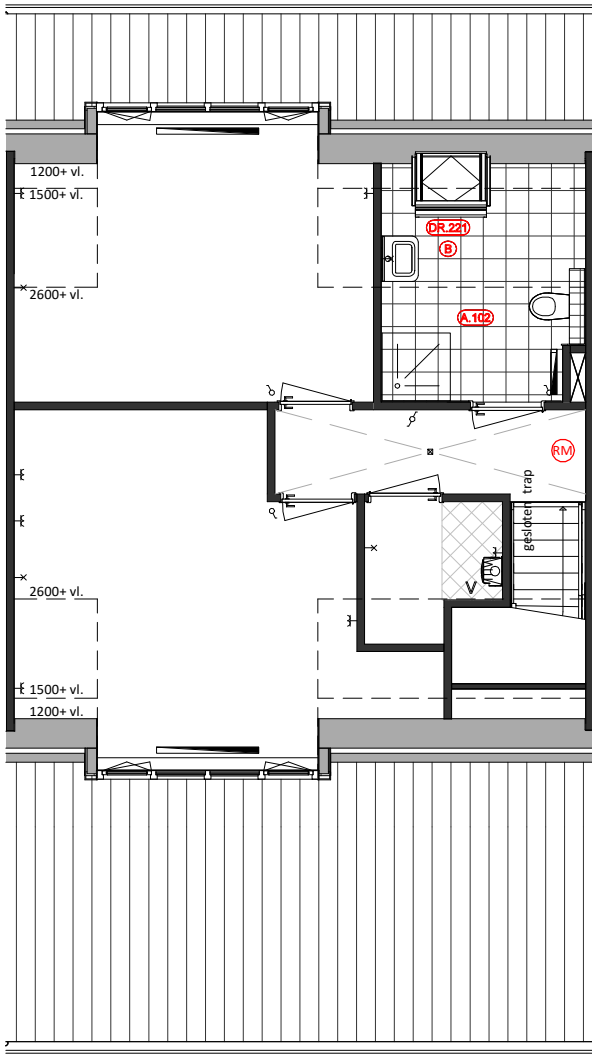
Eerste Verdieping A.102 = Badkamer op 1e verdieping DR.221 = Dakraam
