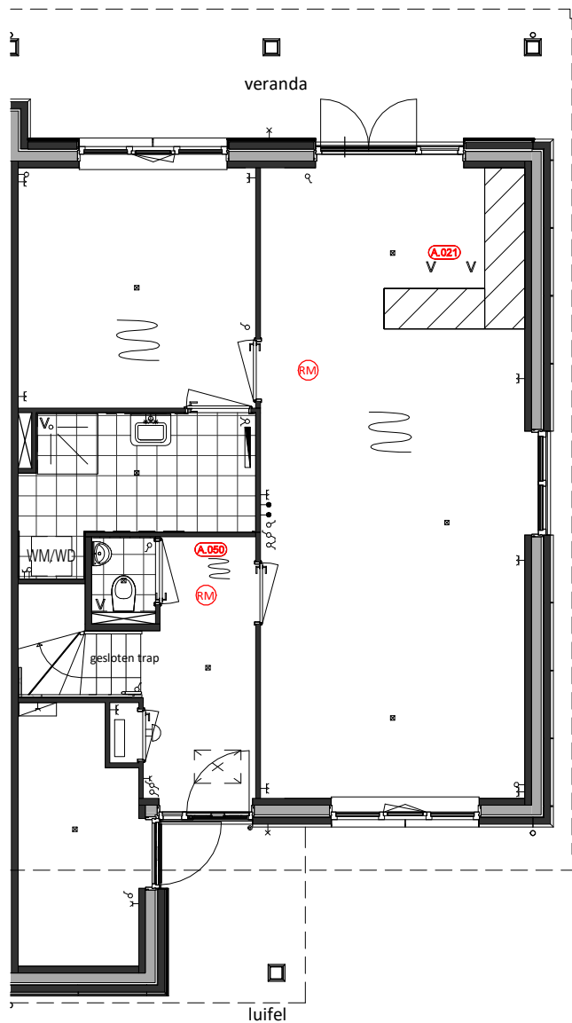
Begane Grond A.021 = Keuken naar achterkant (niet trapzijde) A.050 = Deur naar badkamer vervalt
