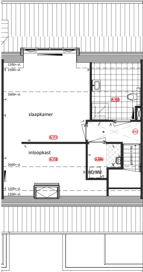
Eerste Verdieping A.102 = Badkamer op 1e verdieping A.111 = Samenvoegen slaapkamer 2 en 3 A.112 = Inloopkast in samengevoegde slaapkamer A.054 = Verplaatsing wasmachine opstelling
