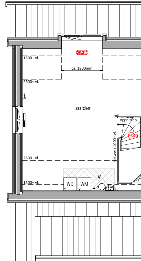
Tweede verdieping DK.211 = Dakkapel type 1 (breedte circa 1800mm) achterzijde
