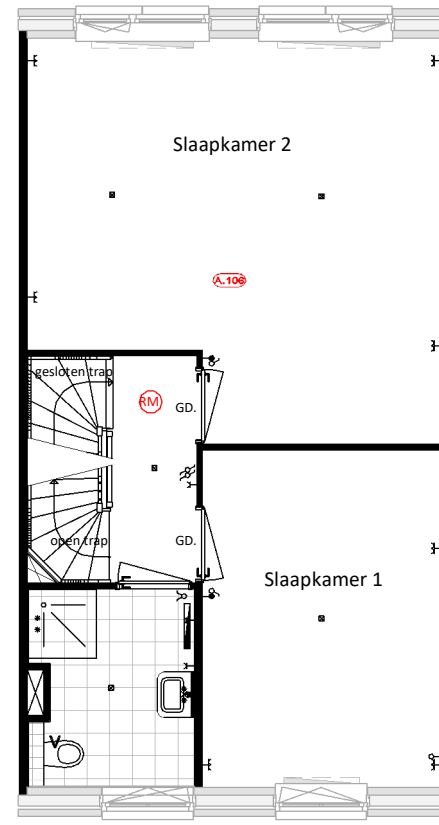
Eerste Verdieping A.106 = Slaapkamers achterzijde van de woning samenvoegen
