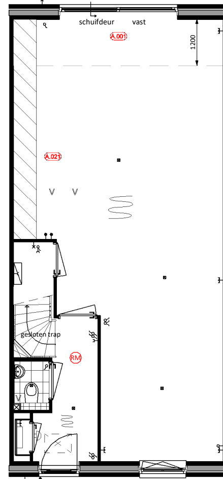
Begane grond A.001 = Uitbouw achtergevel 1,2m A.021 = De keuken wordt naar de achterzijde van de woning geplaatst
