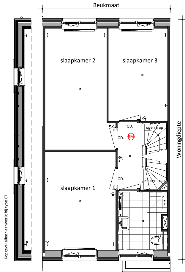
Eerste Verdieping Basis
