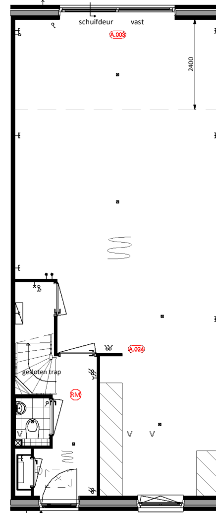
Begane grond A.003 = Uitbouw achtergevel 2,4m A.024 = Kopse wand bij keuken
