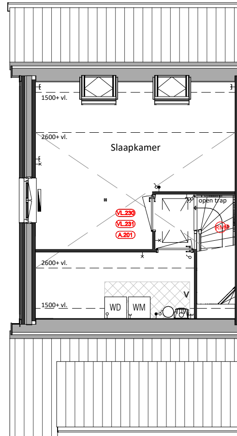
Tweede verdieping VL.230 = Vliering (onafgewerkt) t.b.v. type C5-L VL.231 = Vliering laten afwerken t.b.v. type C5-L A.201 = Zolderindeling 1: Overloop met één slaapkamer en afgesloten techniekruimte
