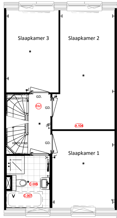
Eerste Verdieping A.104 = Scheidingswand tussen slaapkamer 1 en 2 verplaatsen C.005 = Toilet verplaatsen C.007 = Casco-badaansluitingen
