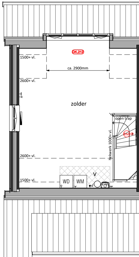
Tweede verdieping DK.212 = Dakkapel type 2 (breedte circa 2900 mm) achterzijde
