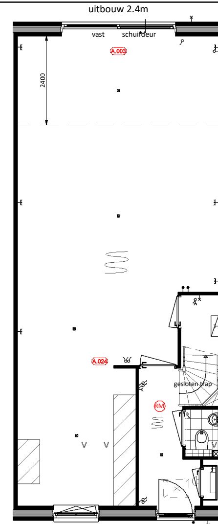
Begane grond A.003 = Uitbouw achtergevel 2,4m A.024 = Kopse wand bij keuken
