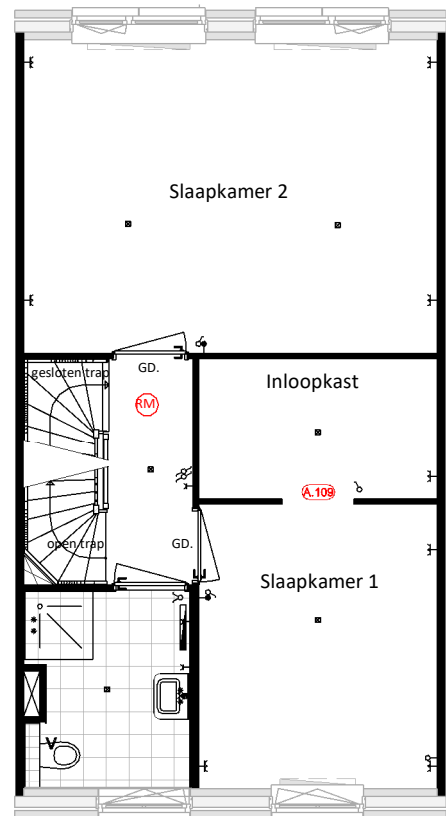
Eerste Verdieping A.109 = Masterbedroom met inloopkast aan voorzijde van de woning
