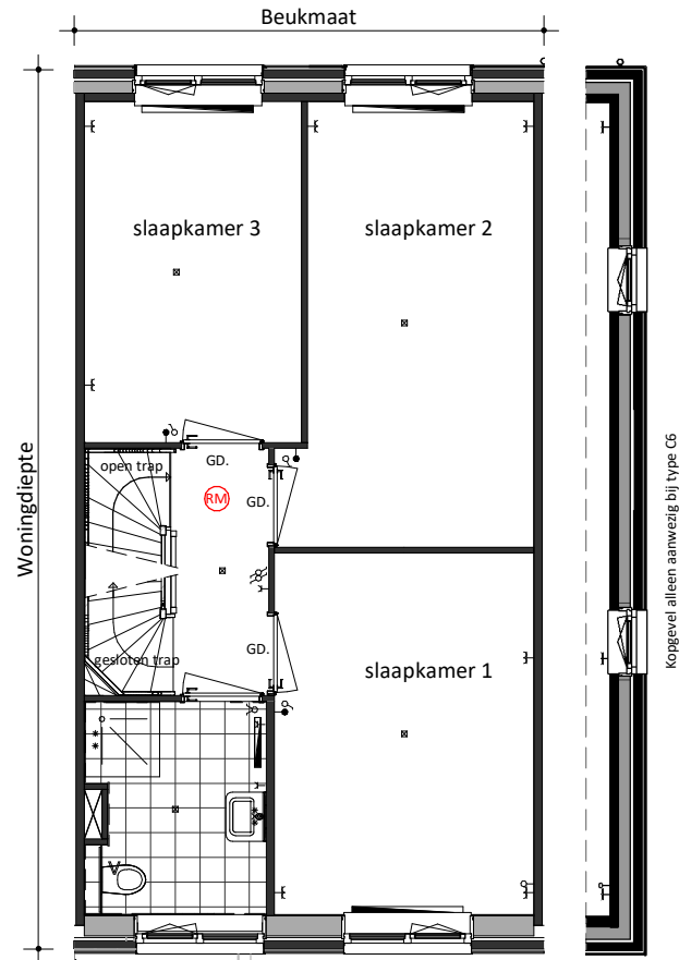
Eerste Verdieping Basis
