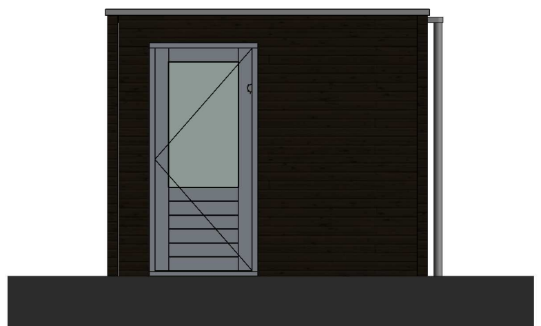
rechtergevel schaal 1:50
