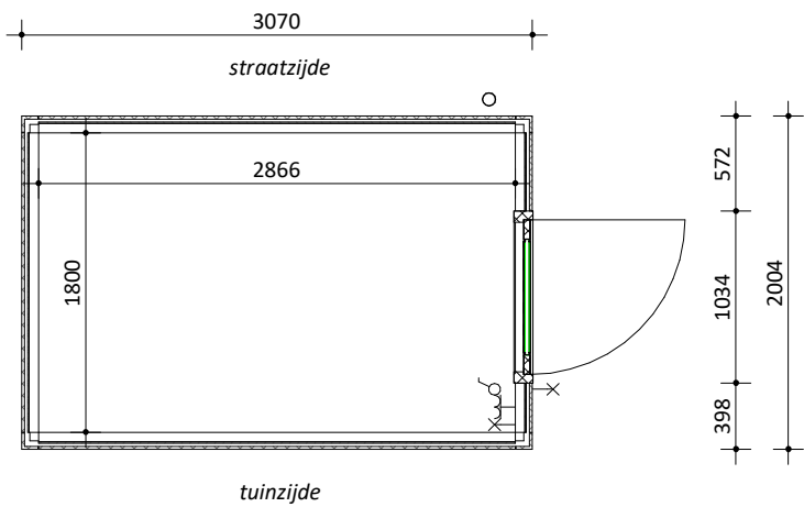
begane grond schaal 1:50
