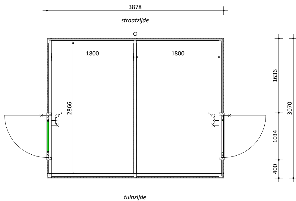
begane grond schaal 1:50
