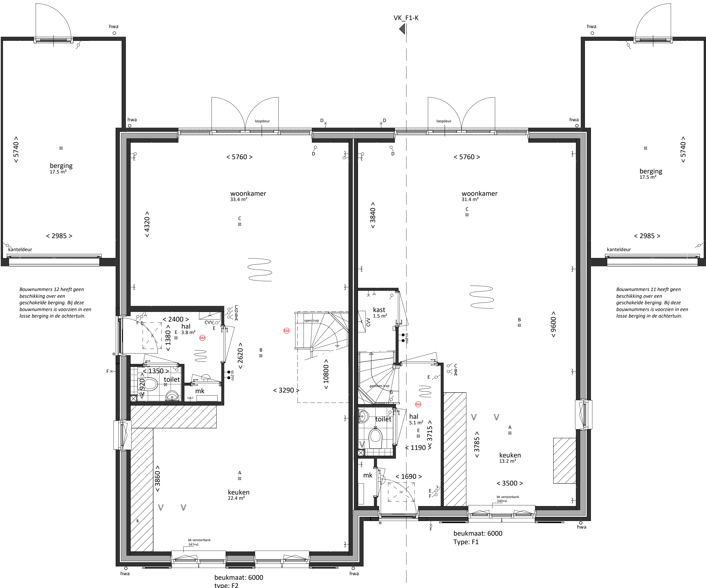
begane grond bk. vloer = P = 0 schaal 1:50
