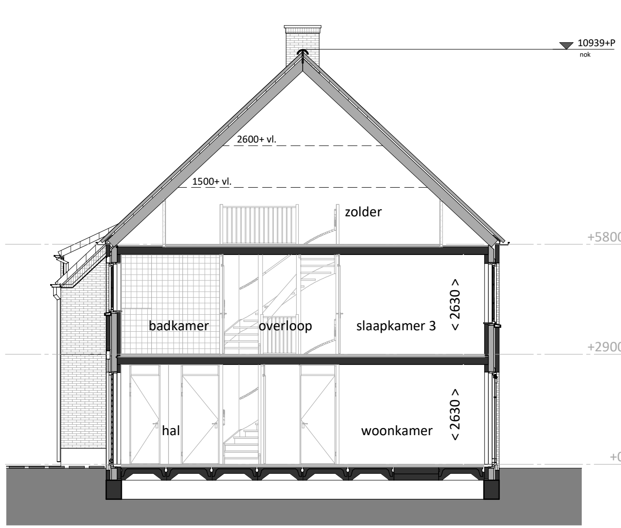
doorsnede schaal 1:100
