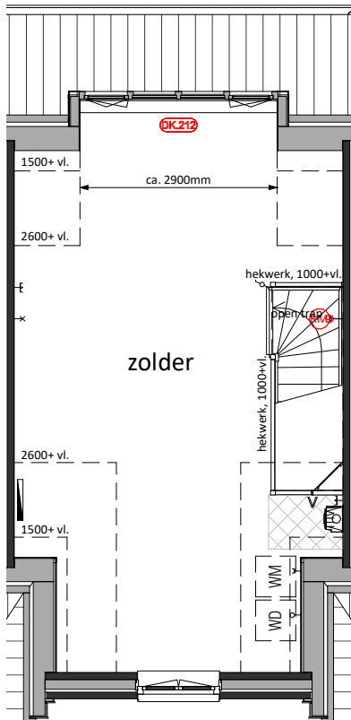
Tweede Verdieping DK.212 = Dakkapel ca.2900mm
