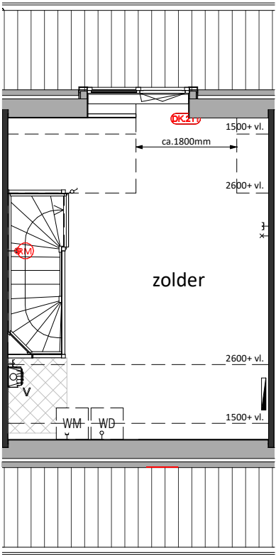
Tweede Verdieping DK.211 = Dakkapel ca.1800mm
