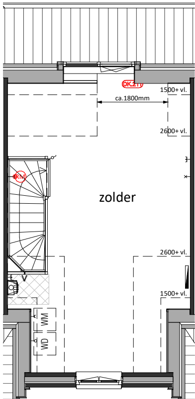
Tweede Verdieping DK.211= Dakkapel ca.1800mm
