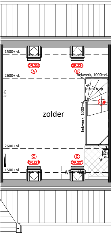
Tweede Verdieping DR.221 = Dakraam
