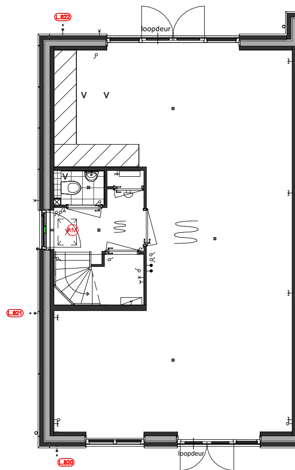
Begane grond L.820 = Vorstvrije buitenkraan (gevelplaat) op de voorgevel L.821 = Vorstvrije buitenkraan (gevelplaat) op de Zijgevel L.822 = Vorstvrije buitenkraan (gevelplaat) op de achtergevel
