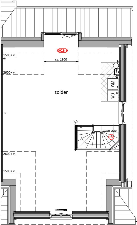
Tweede verdieping DK.211 = Dakkapel type 1 (breedte circa 1800mm) achterzijde
