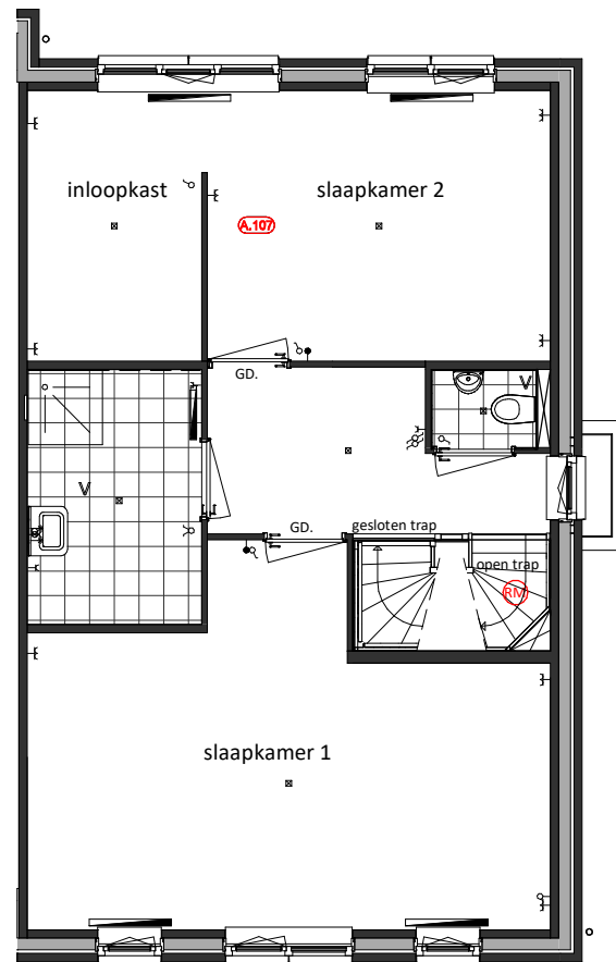
Eerste verdieping A.107 = Masterbedroom met inloopkast achterzijde woning
