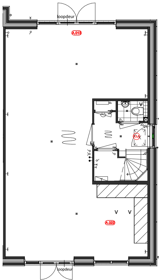
Begane grond A.013 = Wijzigen schuwend deel schuifpui A.022 = De keuken wordt naar de voorzijde van de woning verplaatst
