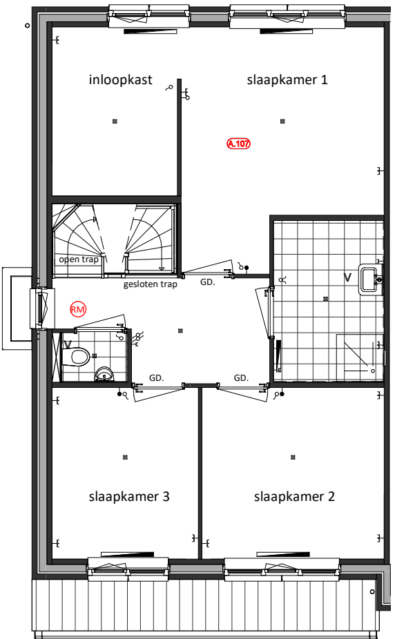
Eerste verdieping
