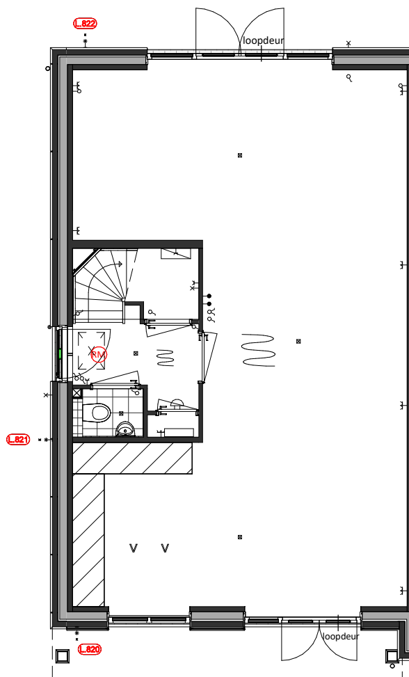
Begane grond L.820 = Vorstvrije buitenkraan (gevelplaat) op de voorgevel L.821 = Vorstvrije buitenkraan (gevelplaat) op de Zijgevel L.822 = Vorstvrije buitenkraan (gevelplaat) op de achtergevel
