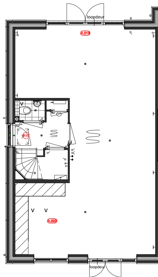
Begane grond A.013 = Wijzigen schuivende deel schuifpui of loopdeur openslaande deuren A.022 = De keuken wordt naar de voorzijde van de woning verplaatst
