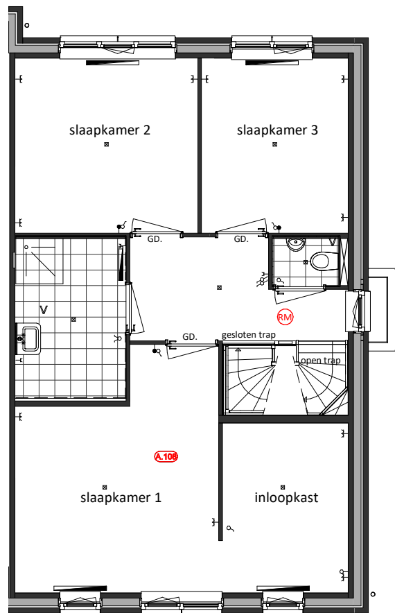
Eerste verdieping A.108 = Masterbedroom met inloopkast voorzijde woning
