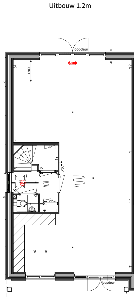
Begane grond A.001 = Uitbouw achtergevel 1.2m
