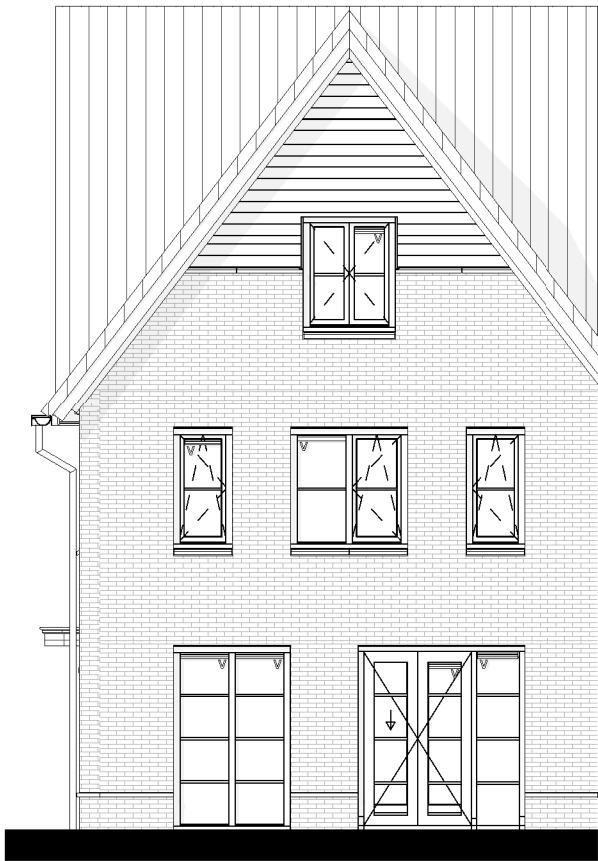
Voorgevel Basis
