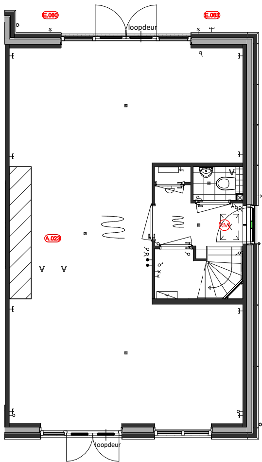
Begane grond A.023 =Keuken in het midden van de woning A.060 = Extra buitenlichtpunt E.063 = Dubbele WCD op achtergevel
