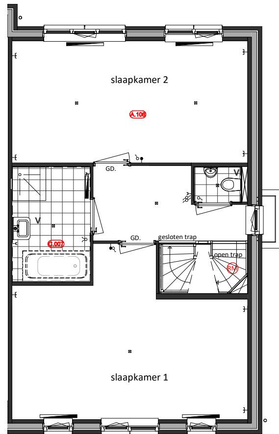
Eerste verdieping A.106 = Slaapkamers voorzijde samenvoegen C.007 = Casco Badaansluiting
