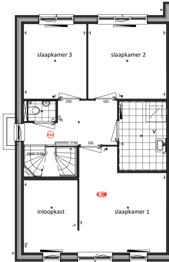
Eerste verdieping
