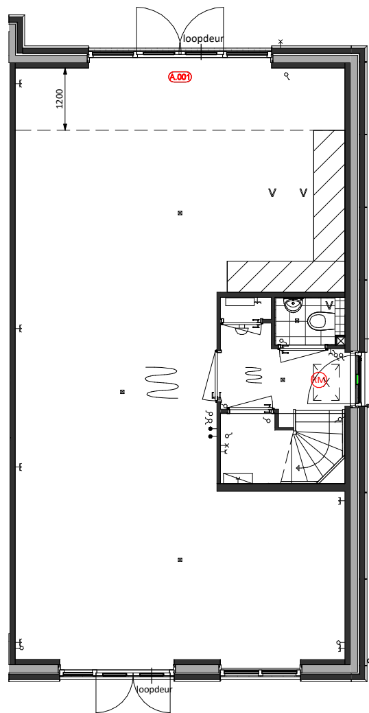
Begane grond A.001 = Uitbouw achtergevel 1.2m
