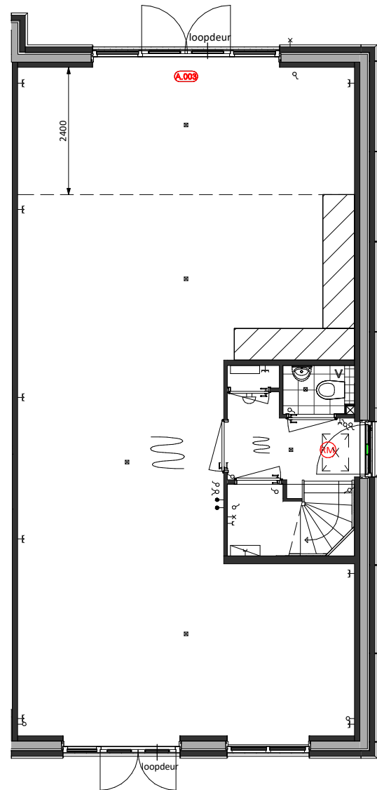
Begane grond A.003 = Uitbouw achtergevel 2.4m
