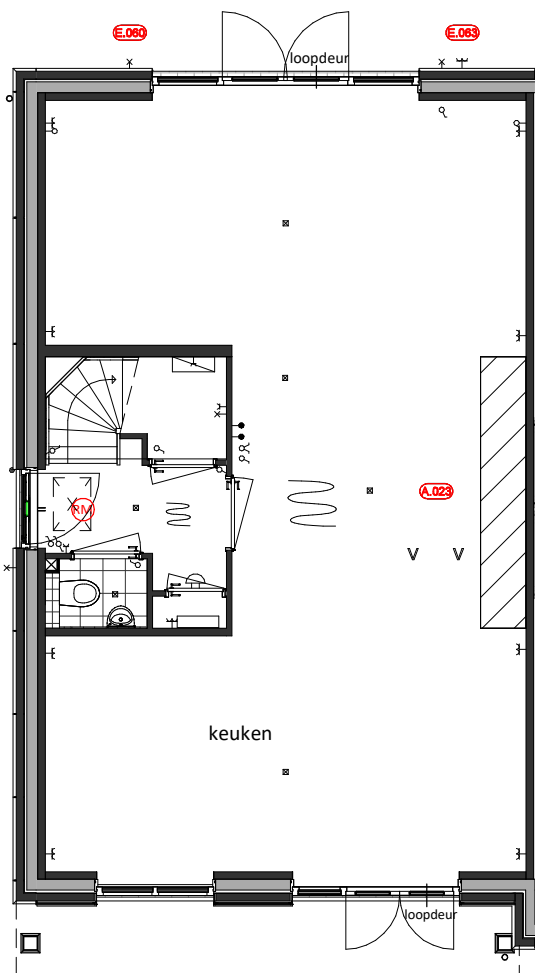
Begane grond A.023 = Keuken in het midden van de woning A.060 = Extra buitenlichtpunt E.063 = Dubbele WCD op achtergevel
