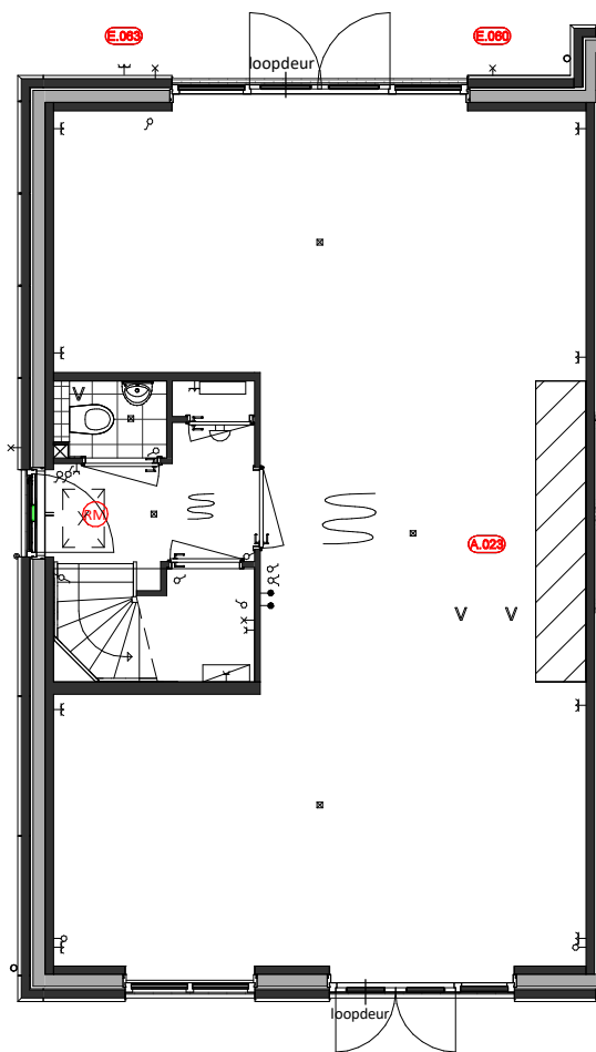
Begane grond A.023 = Keuken in het midden van de woning E.060 = Extra buitenlichtpunt E.063 = Dubbele WCD op achtergevel
