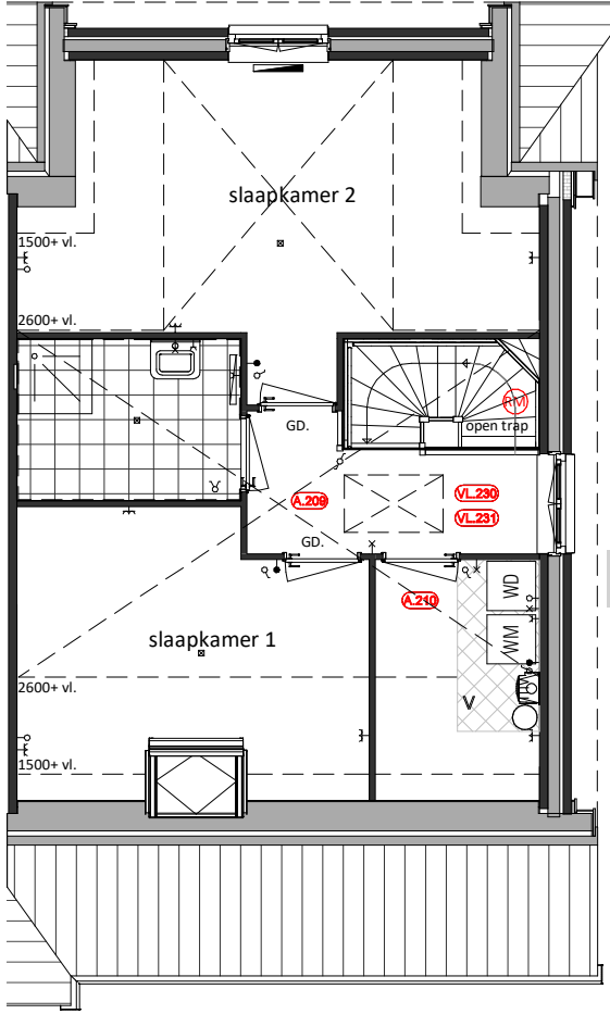
Tweede verdieping A.209 = Zolderindeling; Overloop met twee slaapkamers en badkamer A.210 = Zolderindeling; Afgesloten techniek-/wasruimte (alleen i.c.m. optie 2 of 7) VL.230 = Vliering (onafgewerkt) t.b.v. type G1-L VL.231 = Vlieringlaten afwerken t.b.v. type G1-L
