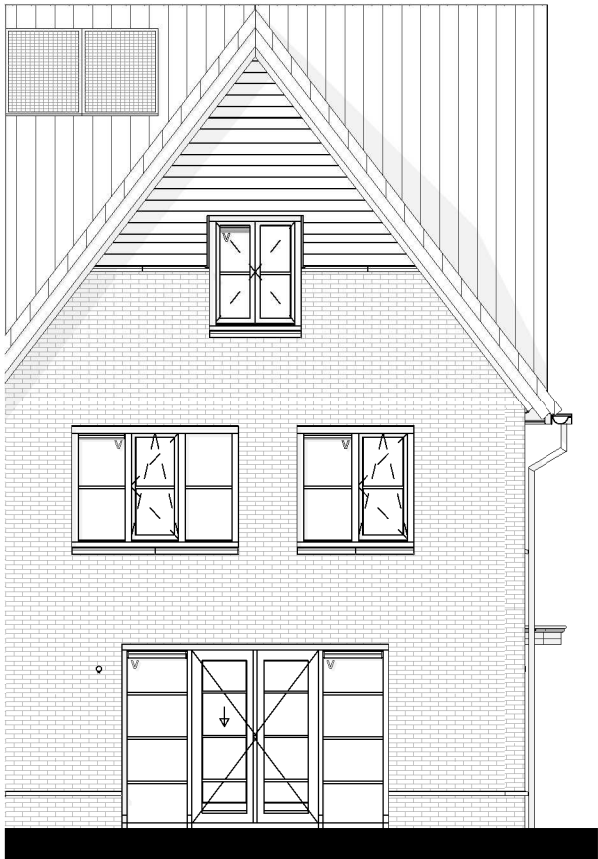
Achtergevel Basis
