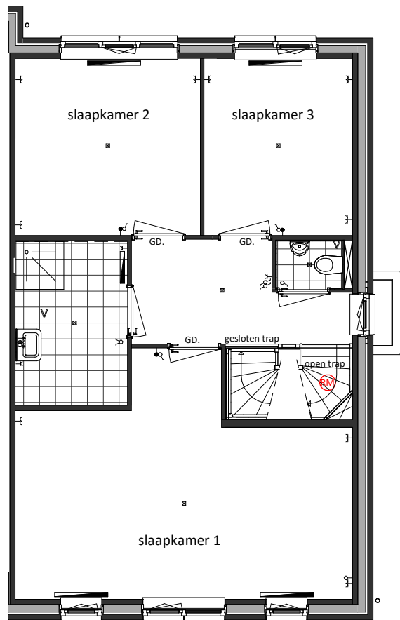
Eerste verdieping Basis
