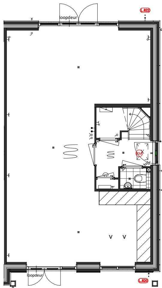
Begane grond L.820 = Vorstvrije buitenkraan (gevelplaat) op de voorgevel L.821 = Vorstvrije buitenkraan (gevelplaat) op de Zijgevel L.822 = Vorstvrije buitenkraan (gevelplaat) op de achtergevel
