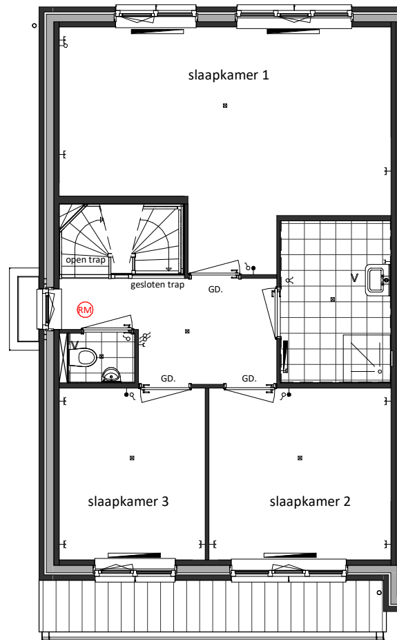
Eerste verdieping
