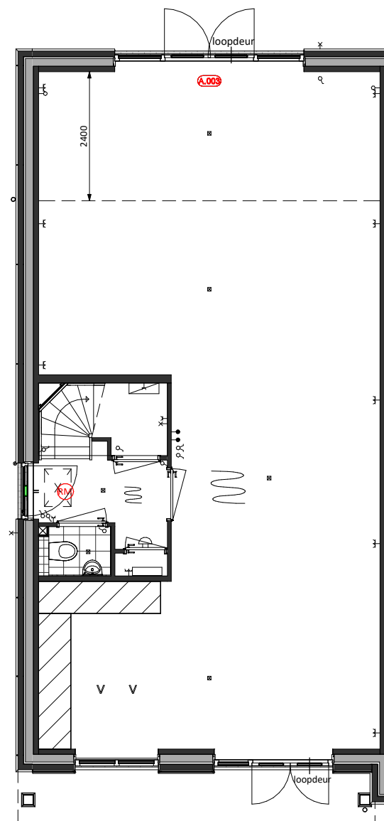
Begane grond A.003 = Uitbouw achtergevel 2.4m
