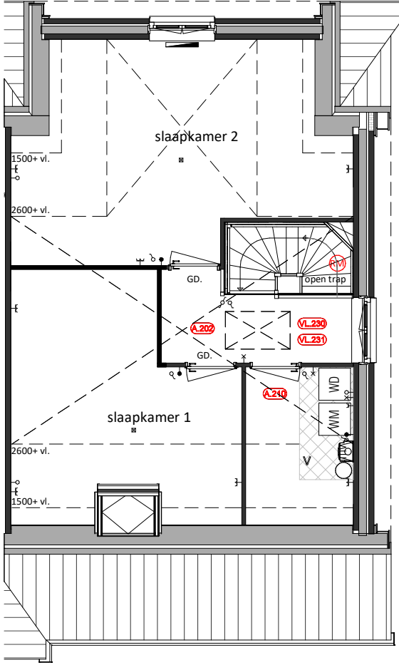
Tweede verdieping A.202 = Zolderindeling; Overloop met twee slaapkamers A.210 = Zolderindeling; Afgesloten techniek-/wasruimte VL.230 = Vliering (onafgewerkt) t.b.v. type G1-L VL.231 = Vlieringlaten afwerken t.b.v. type G1-L
