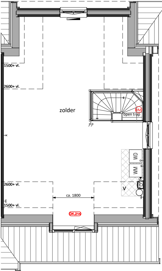
Tweede verdieping DK.214 = Dakkapel type 4 (breedte circa 1800 mm) voorzijde
