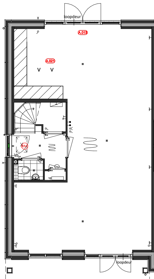
Begane grond A.013 = Wijzigen schuivende deel schuifpui of loopdeur openslaande deuren A.021 = De keuken wordt naar de achterzijde van de woning geplaatst
