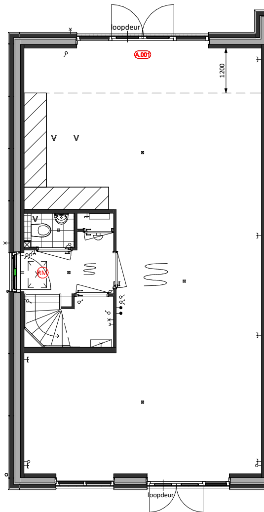
Begane grond A.001 = Uitbouw achtergevel 1.2m
